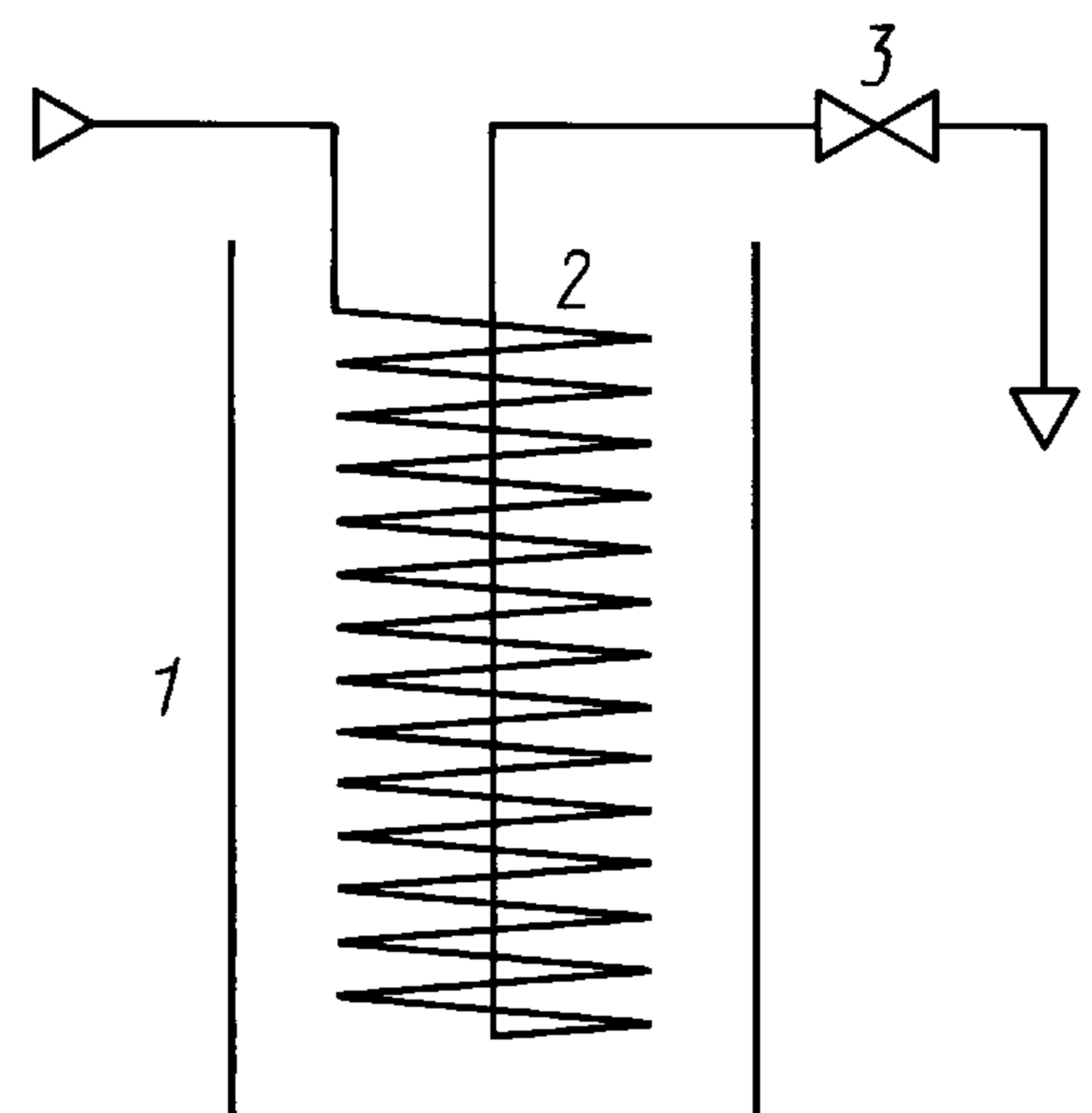
Устройство для охлаждения сжиженного углеводородного газа
