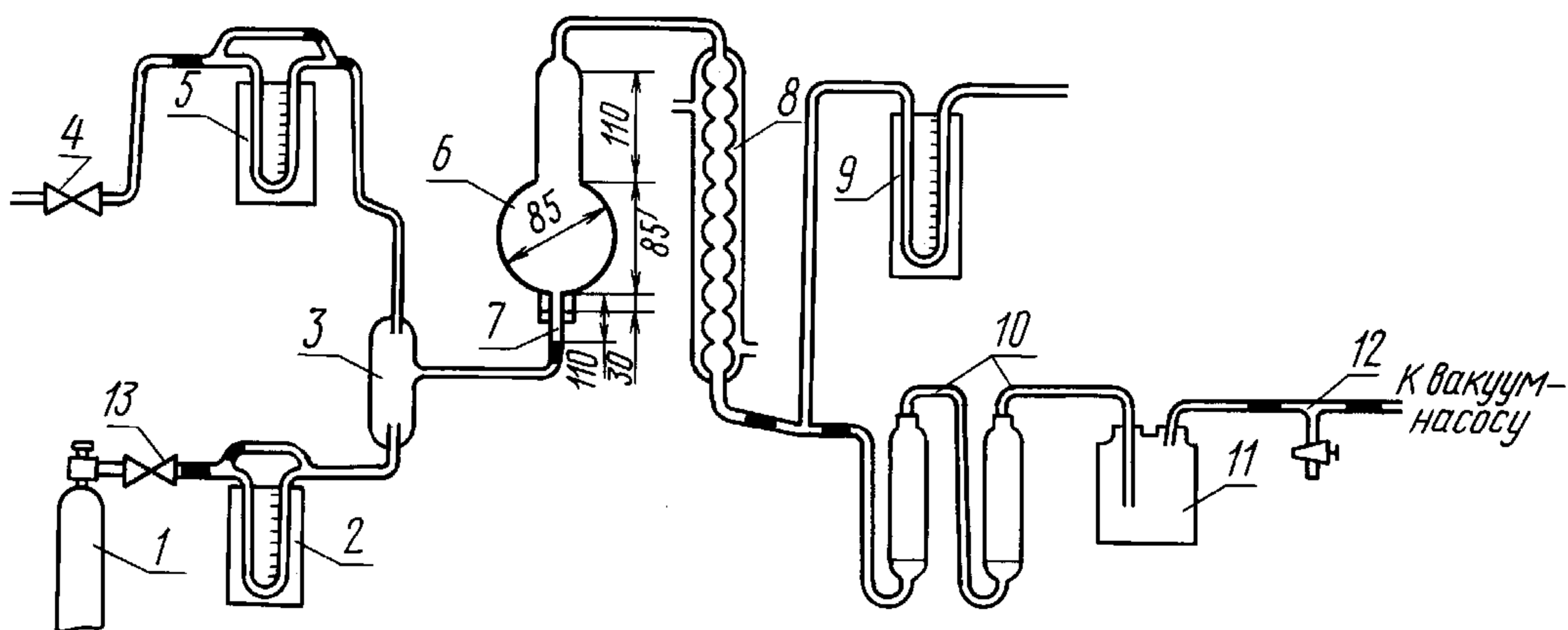
Прибор для определения массовой доли общей серы
