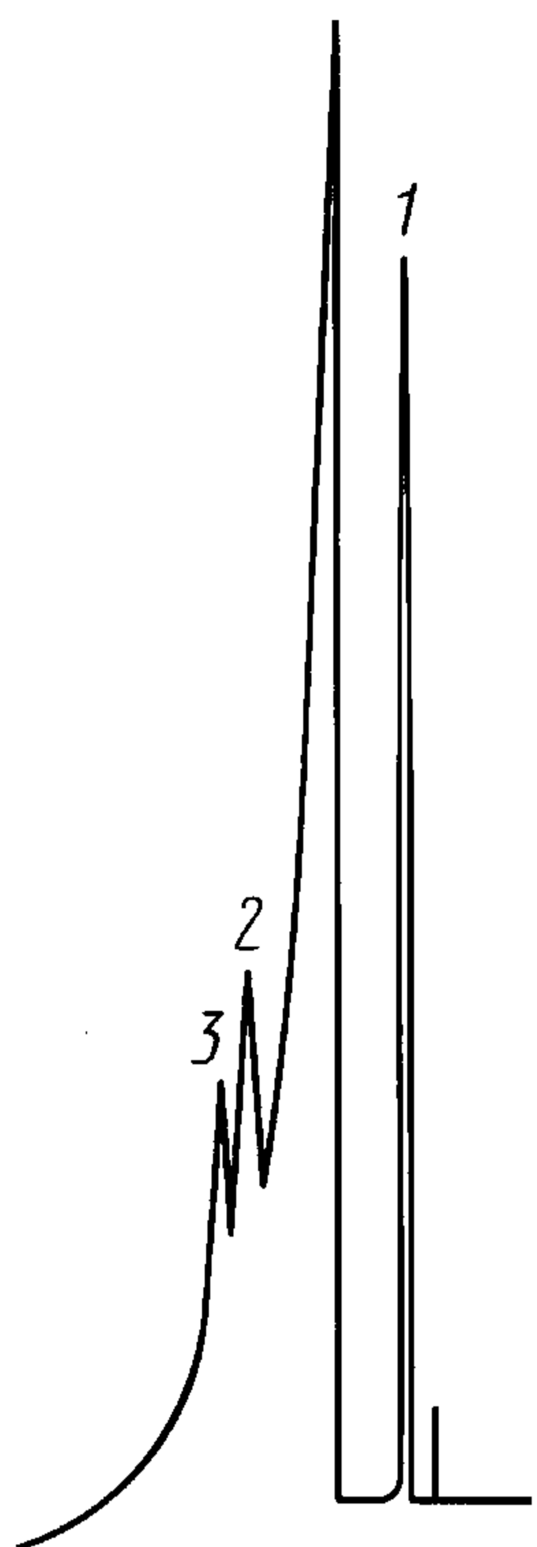
1 — сумма углеводородов; 2 — метанол; 3 — бензол Черт. 5
