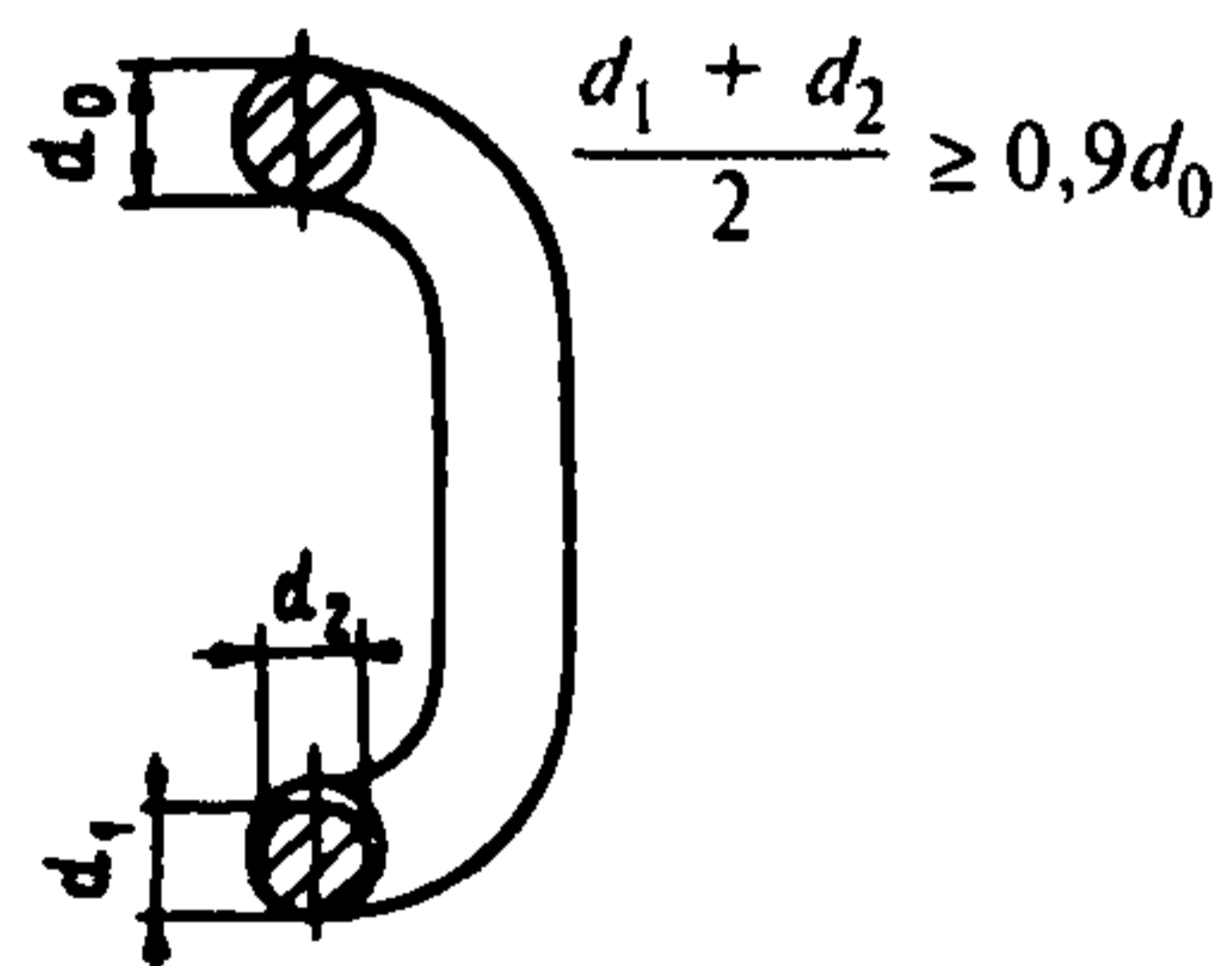
Рис. 2. Уменьшение диаметра сечения звена цепи:
