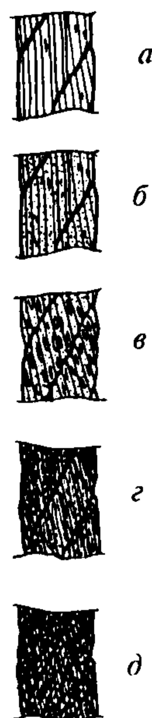
Рис. 6. Поверхностная коррозия проволок каната крестовой свивки: a — начальное окисление поверхности; б — общее окисление поверхности; в — заметное окисление; г — сильное окисление; д — интенсивная коррозия
