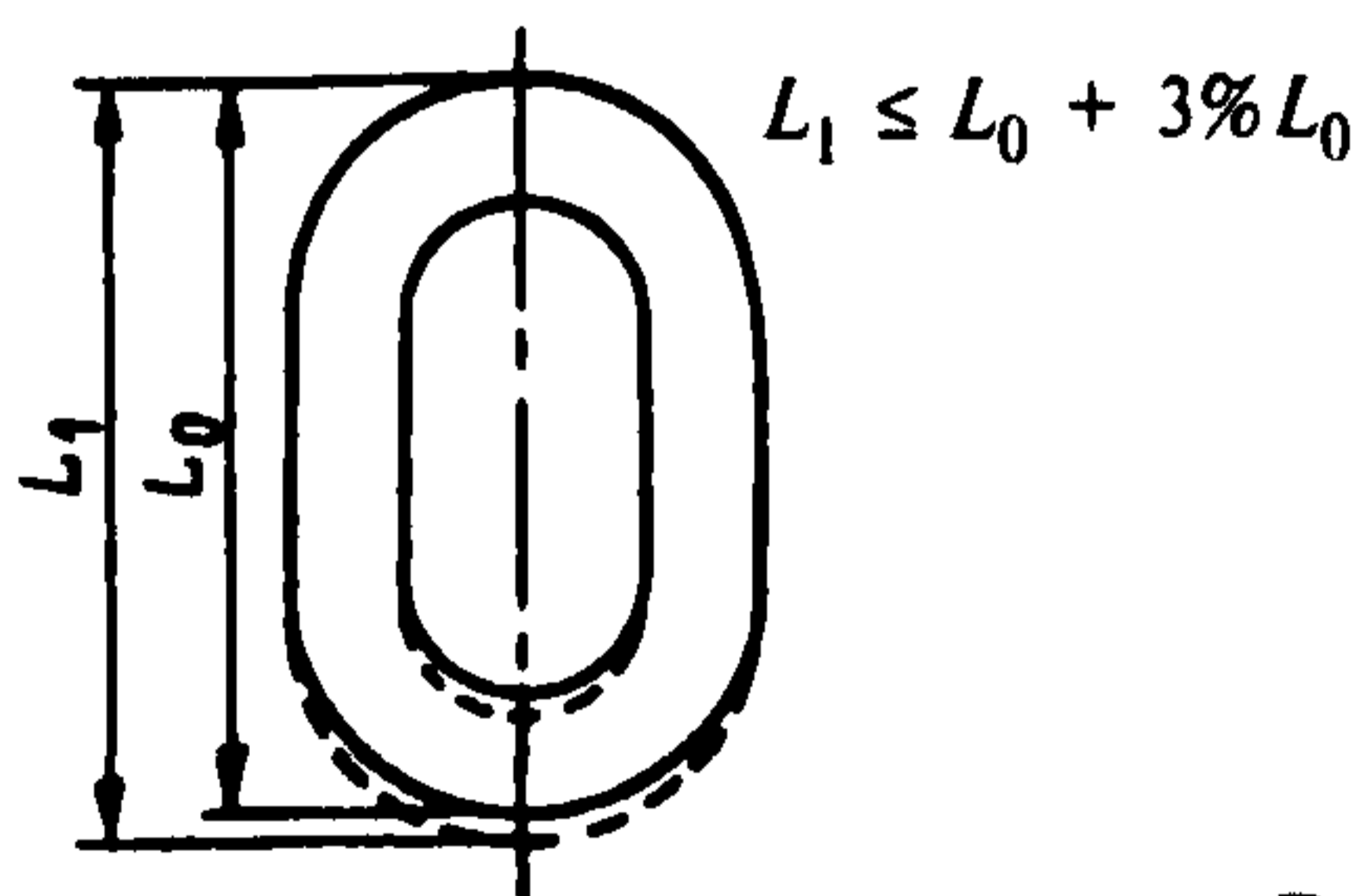
Рис. 1. Увеличение звена цепи:
