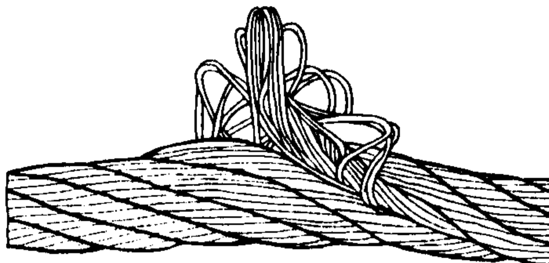
Рис. 11. Выдавливание сердечника
