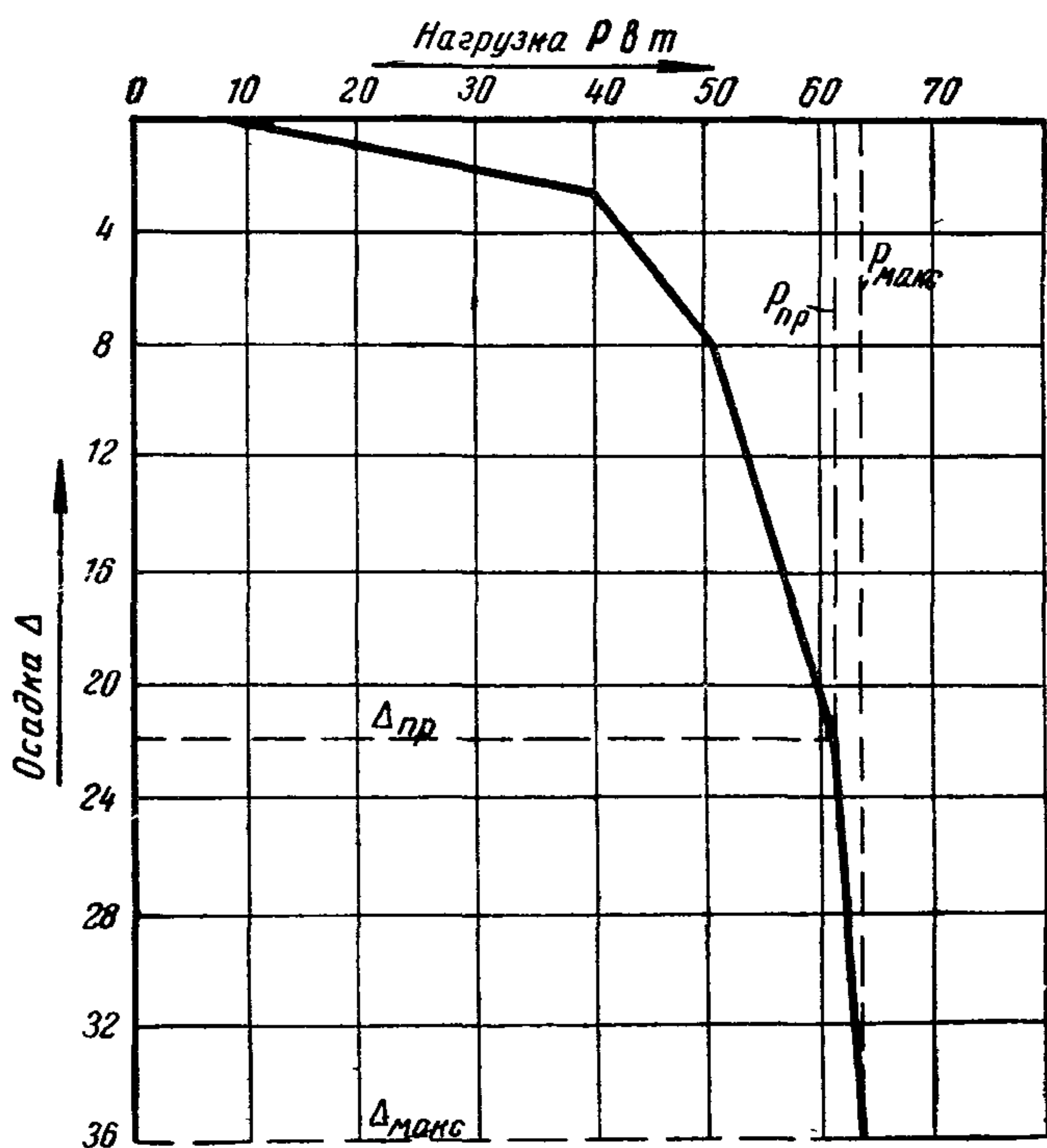
График зависимости осадки сваи \Delta в мм от нагрузки P в т ( P_{\text{макс}} и \Delta_{\text{макс}} — соответственно нагрузка и осадка, достигнутые в конце опыта)
