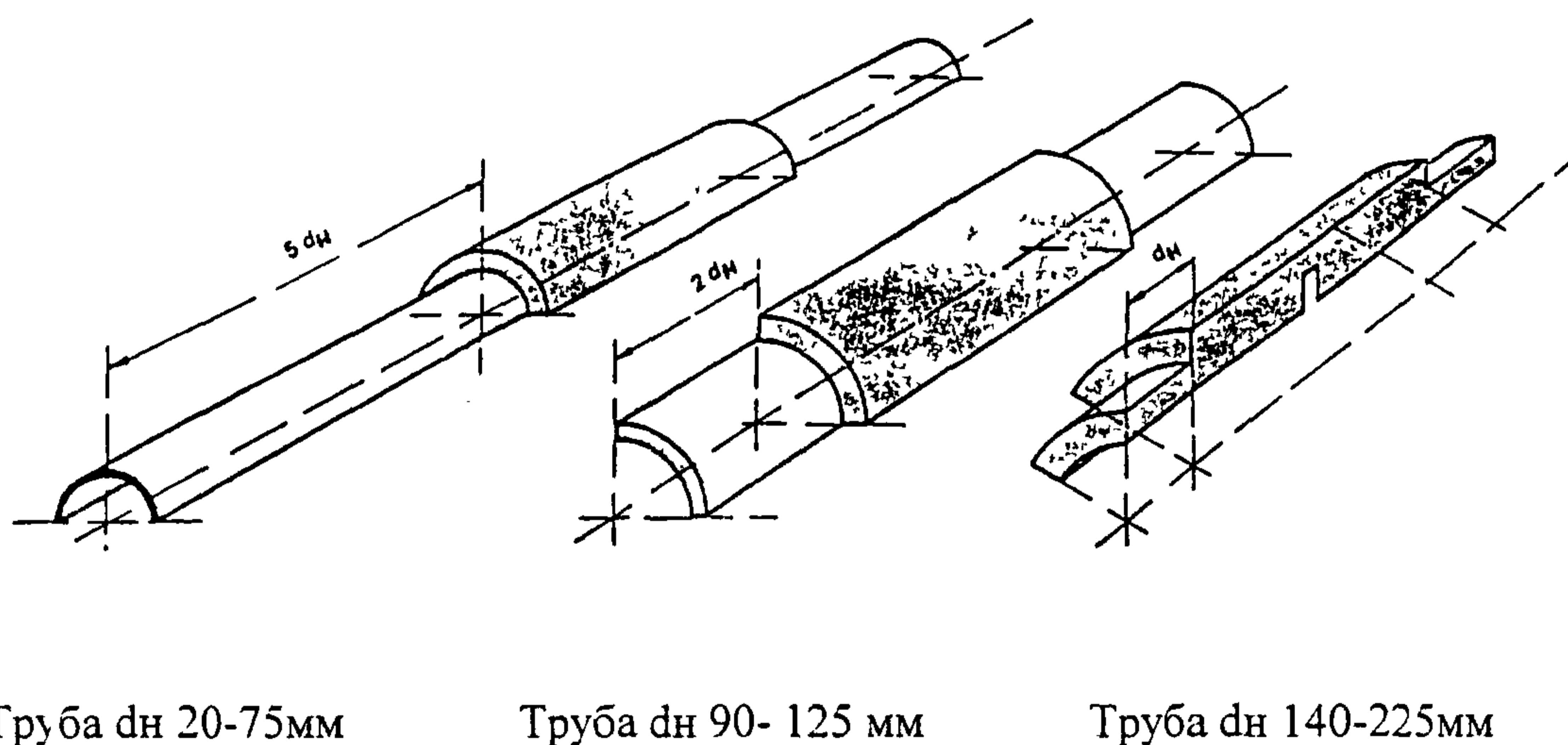
Рисунок Е.1 - Общий вид образцов - сегментов
