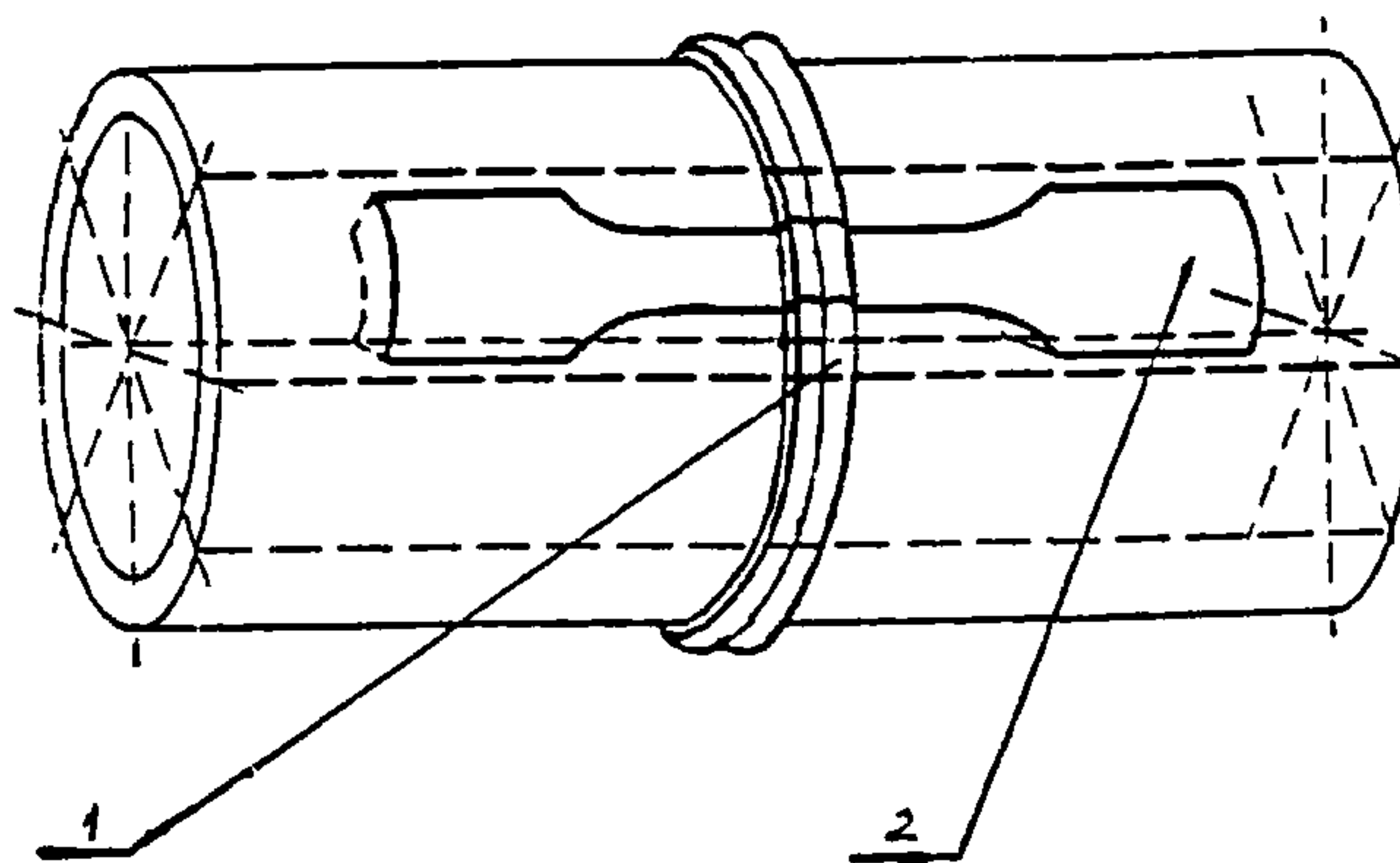
1 - патрубок со сварным соединением, 2 - расположение образцов
