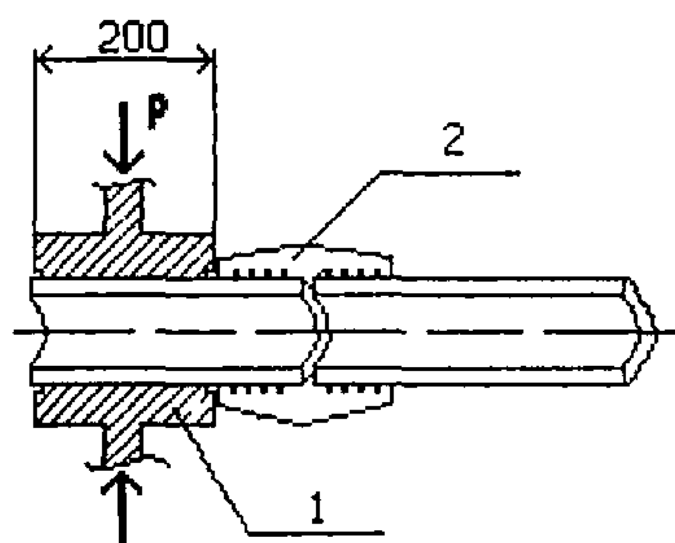
1-обжимные плиты, 2-испытываемый образец
