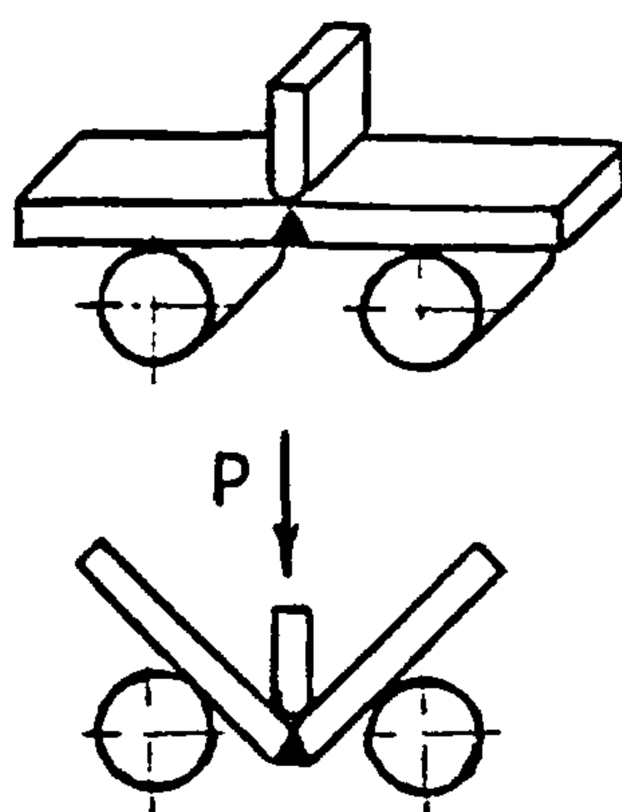
Рисунок И 1 - Схема испытания на статический изгиб
