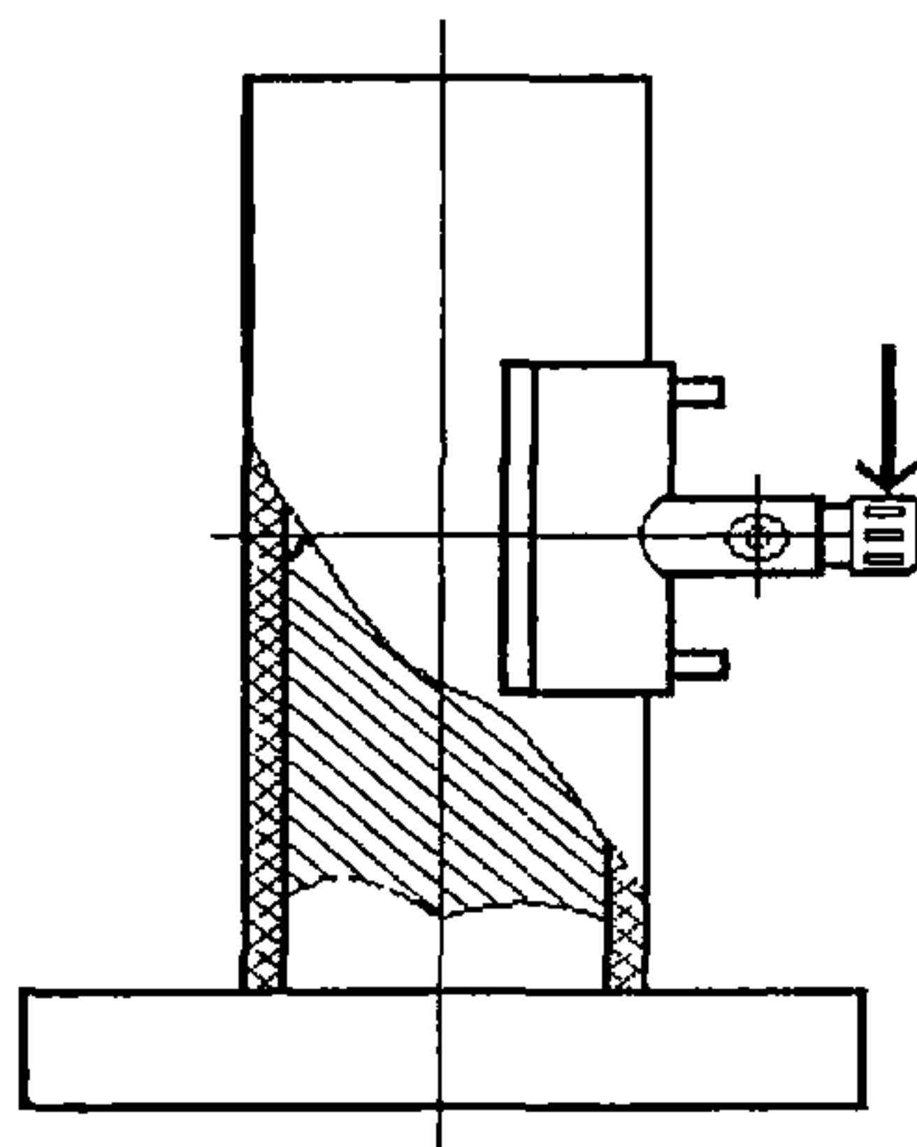
Рисунок М 1 - Схема испытания на стойкость к удару
