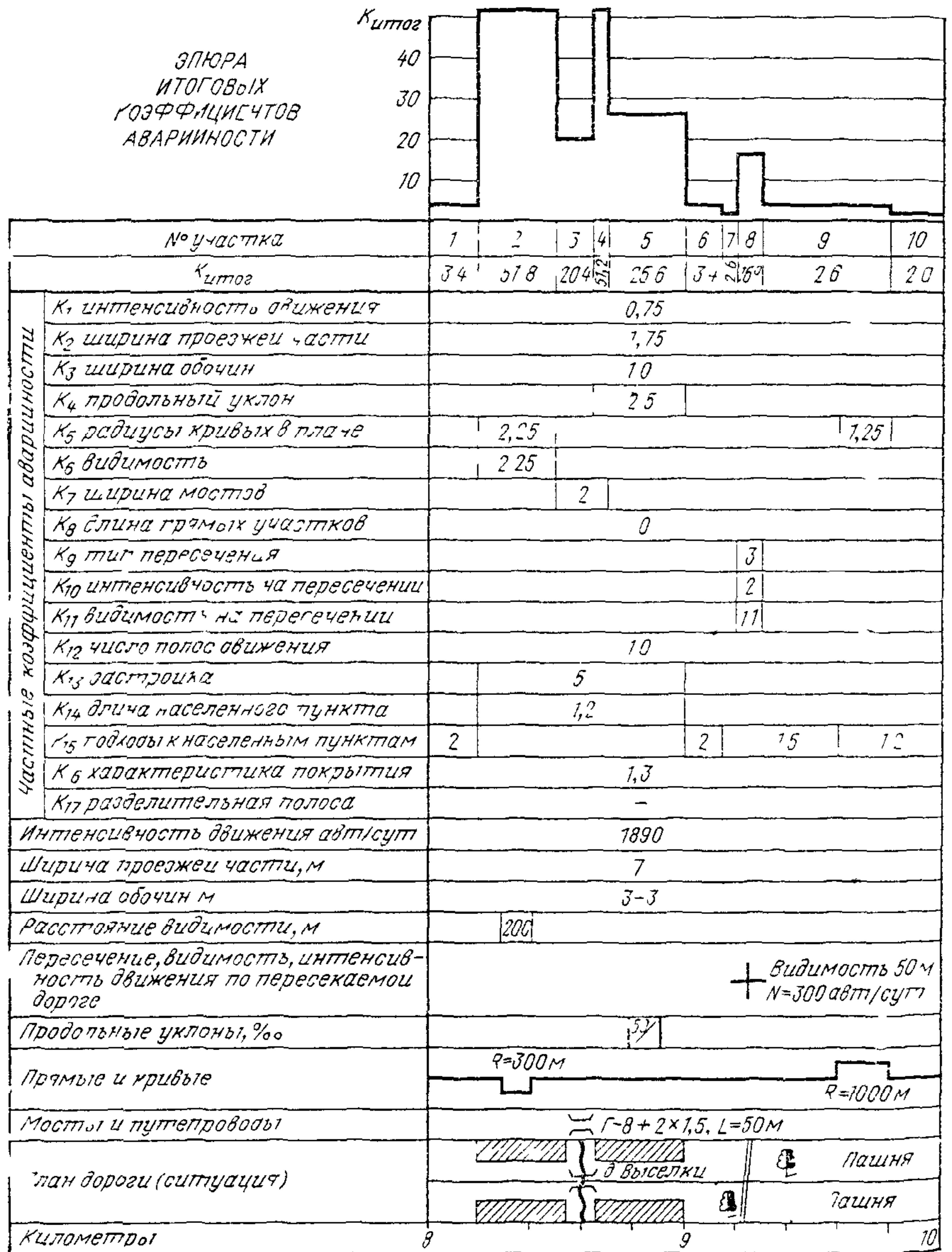
Рис 1 График коэффициентов аварийности на участке автомобильной дороги
