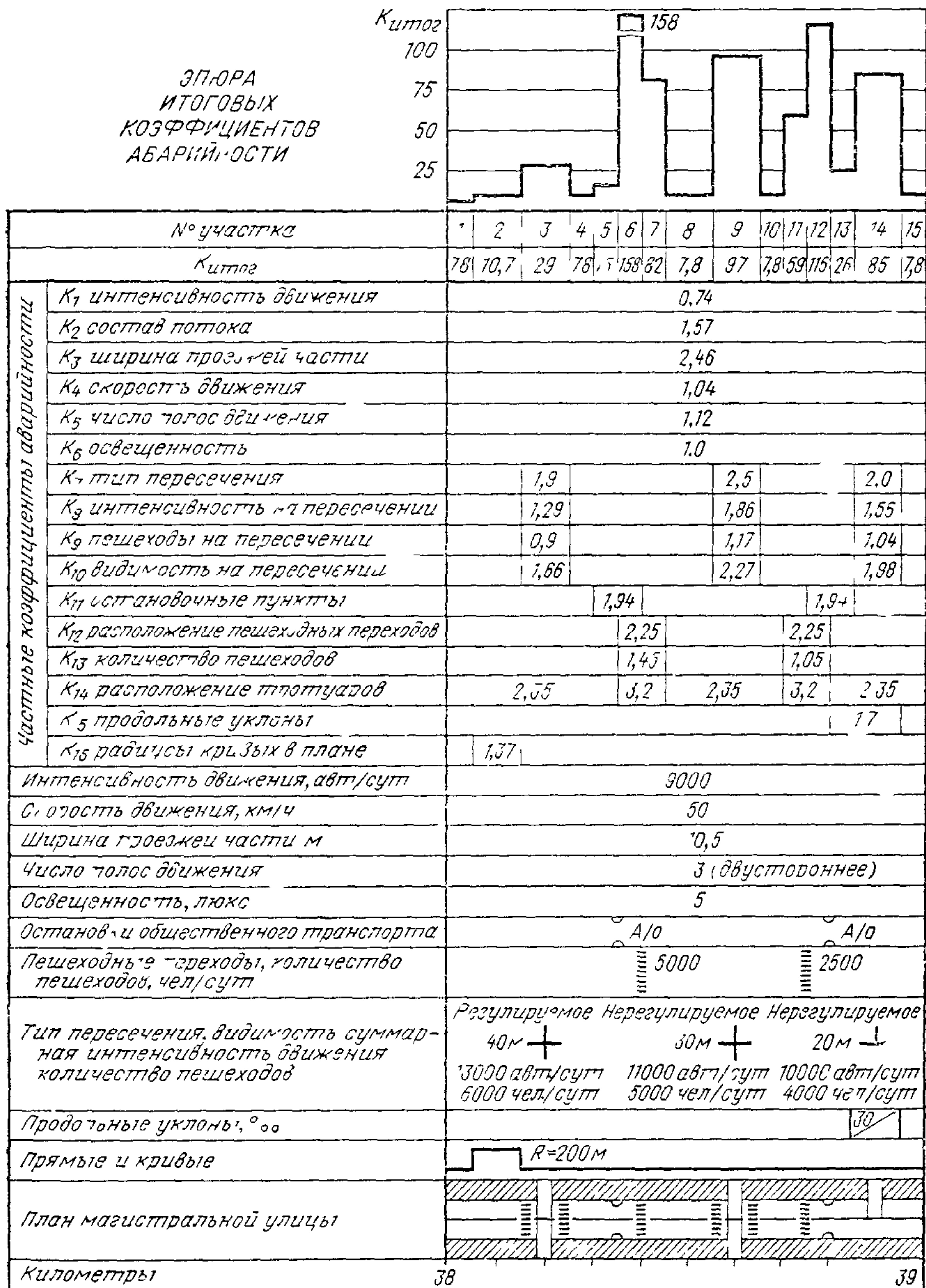
Рис 3 График коэффициентов аварийности на участке магистральной улицы
