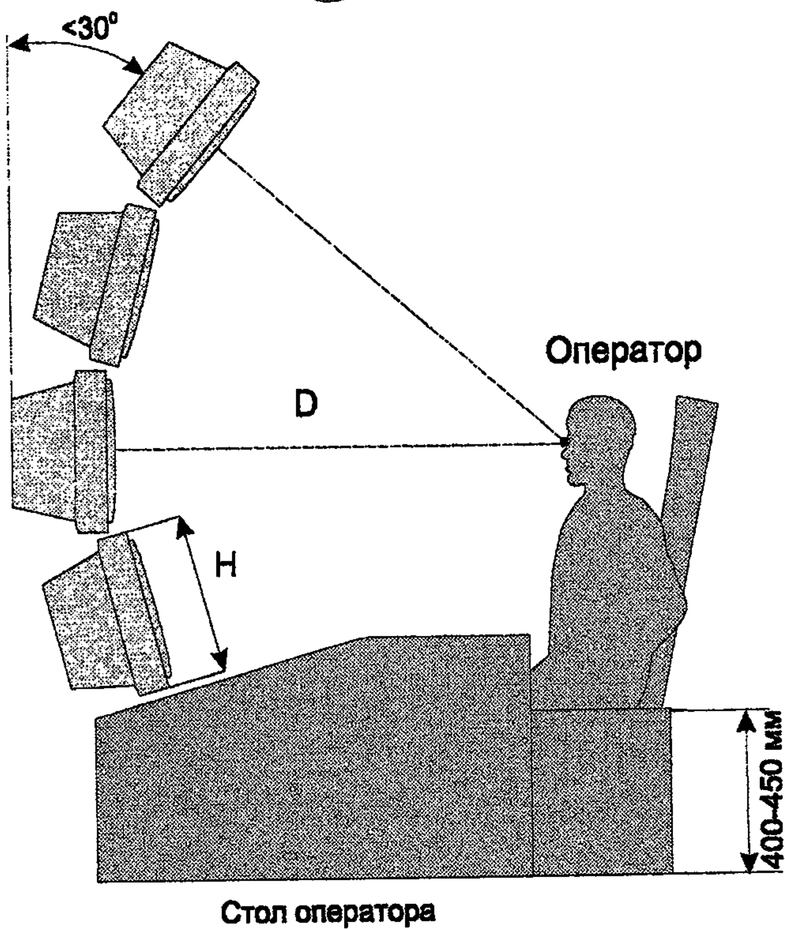
Рисунок 3 – Схема рабочего места оператора
