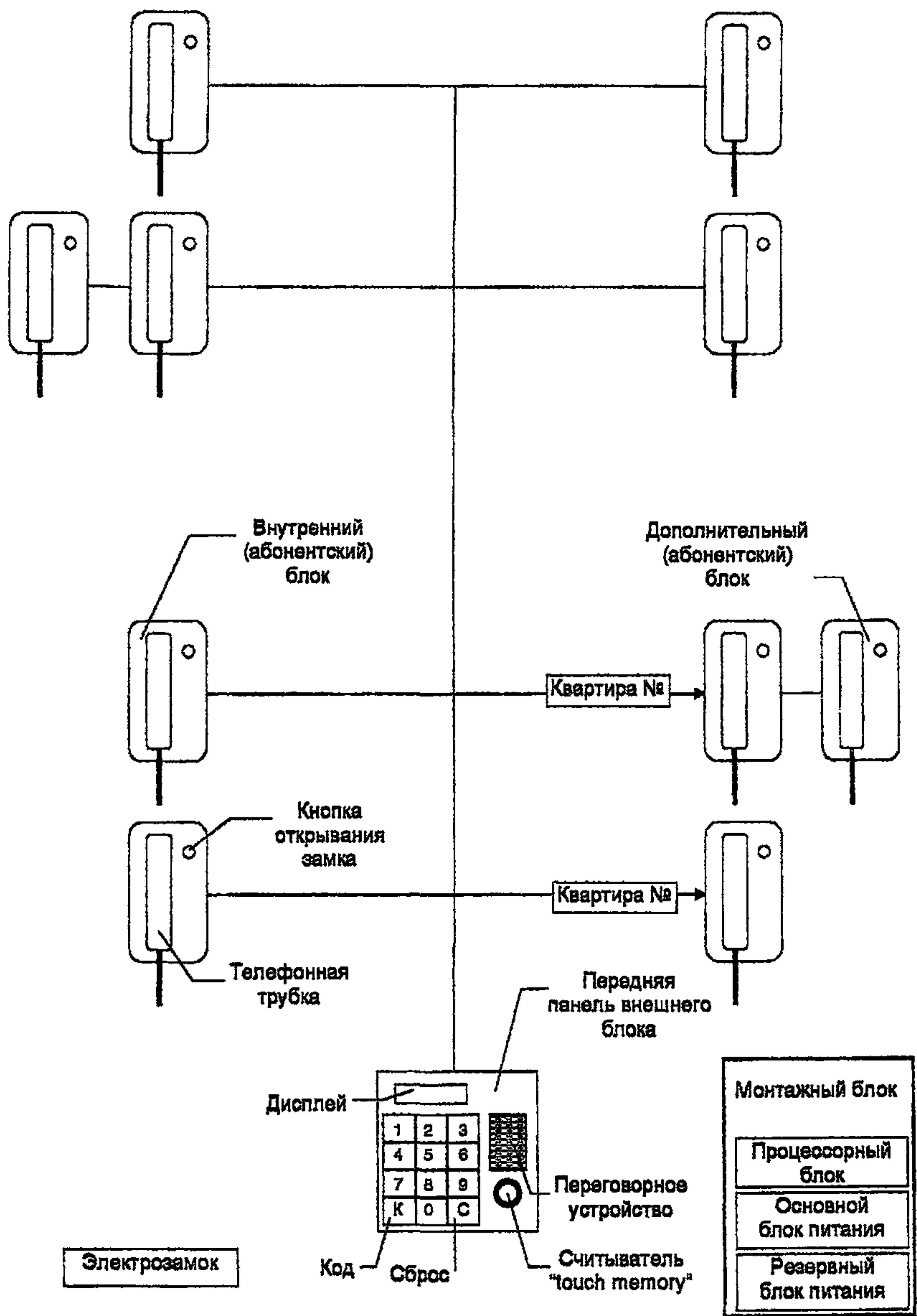
Рисунок 12 - Типовая конфигурация одноуровневого подъездного аудиодомофона
