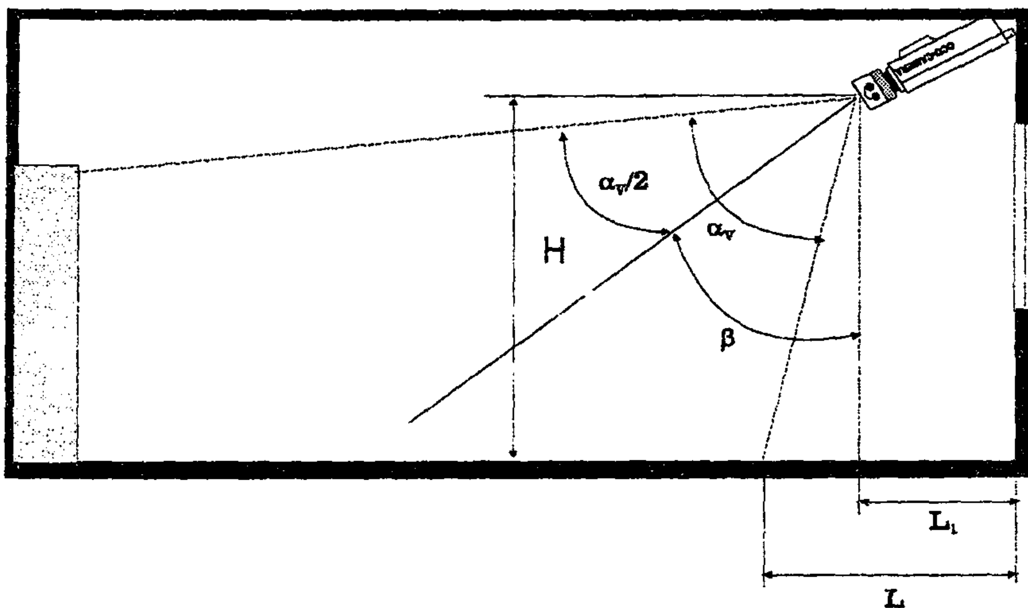
Рисунок 2 - “Мертвая” зона ТК (вид сбоку)
