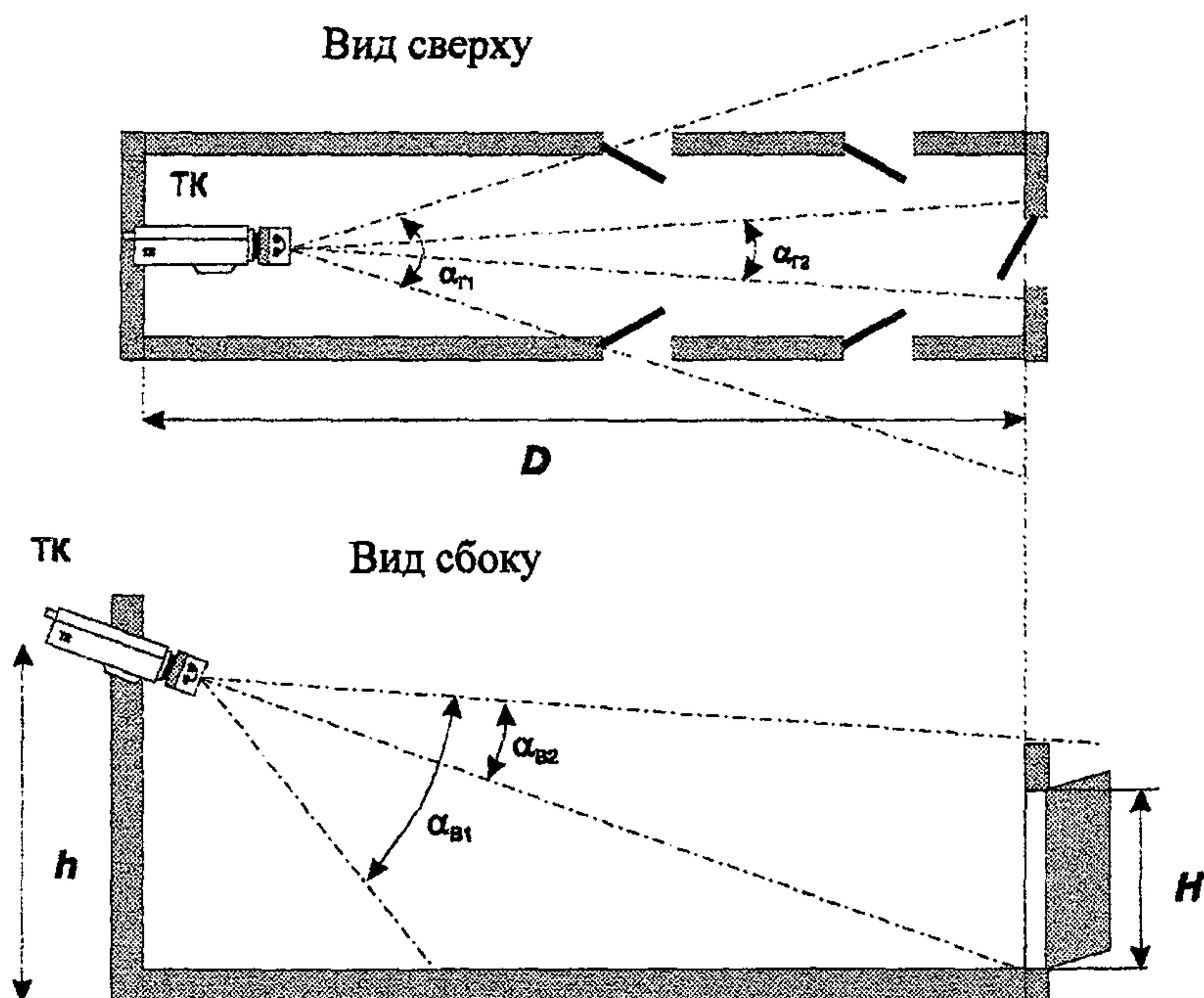
Рисунок 5 - Схемы охраны коридора
