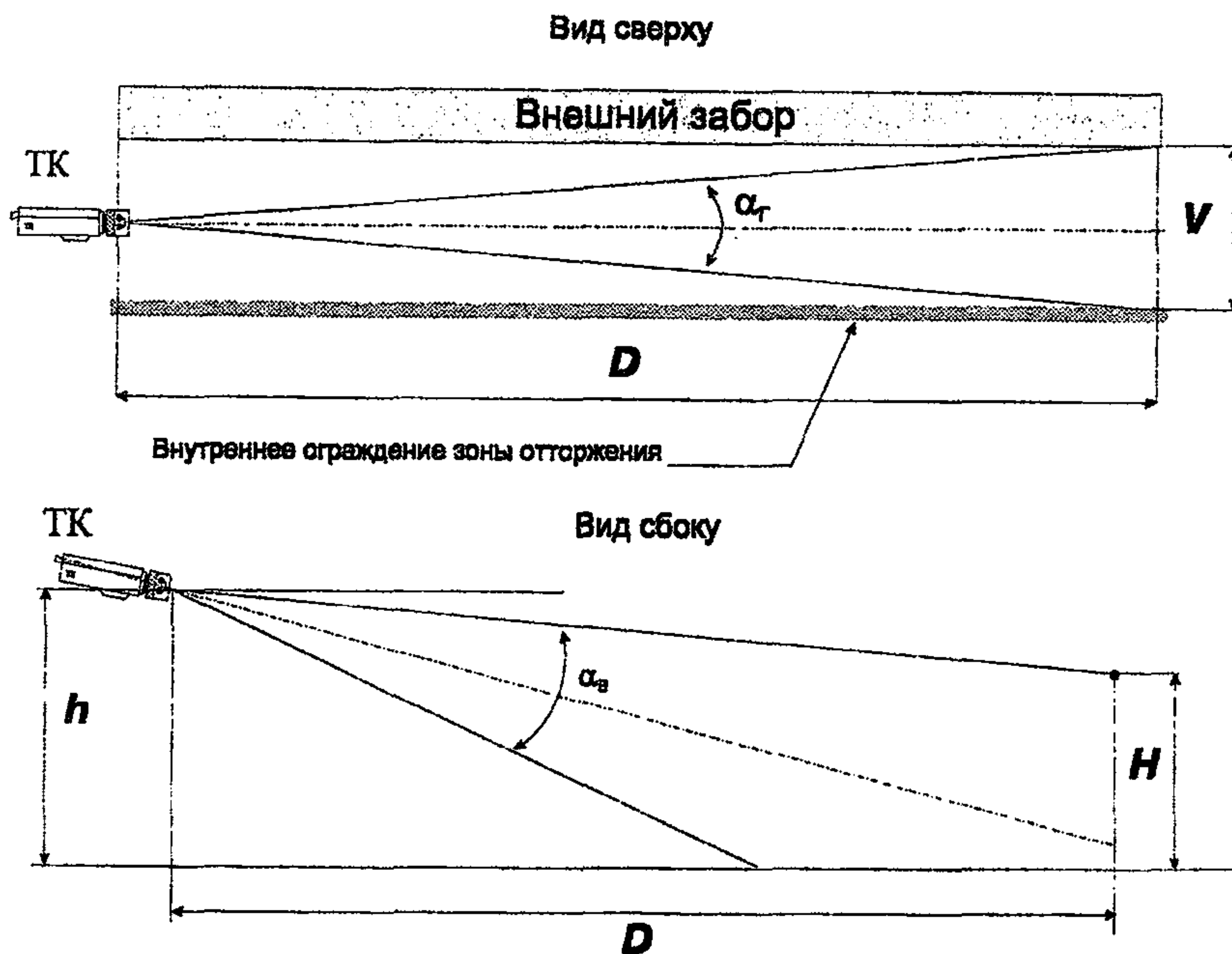
Рисунок 7 - Схемы охраны периметра
