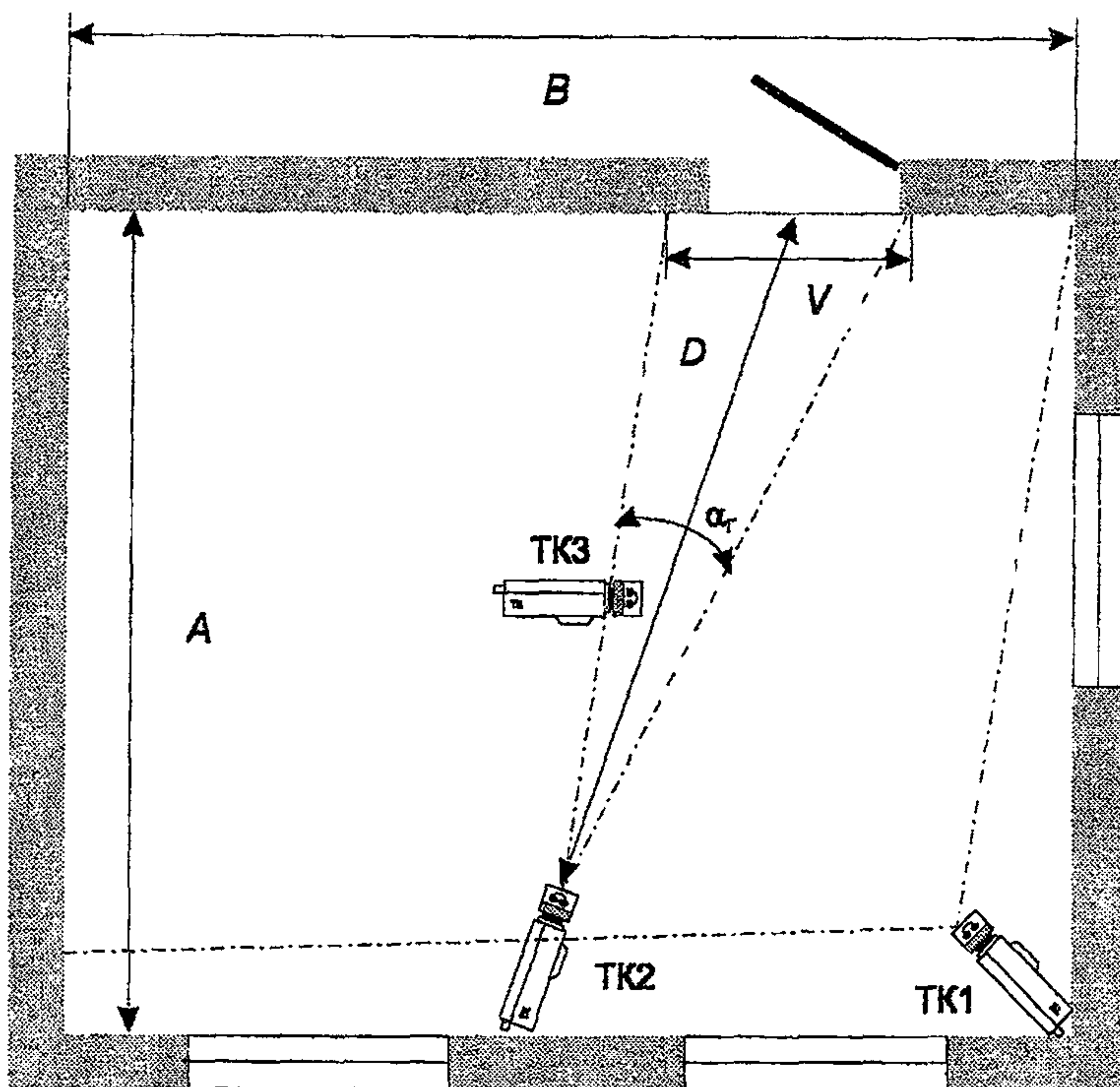
Рисунок 4 – Схема охраны помещения
