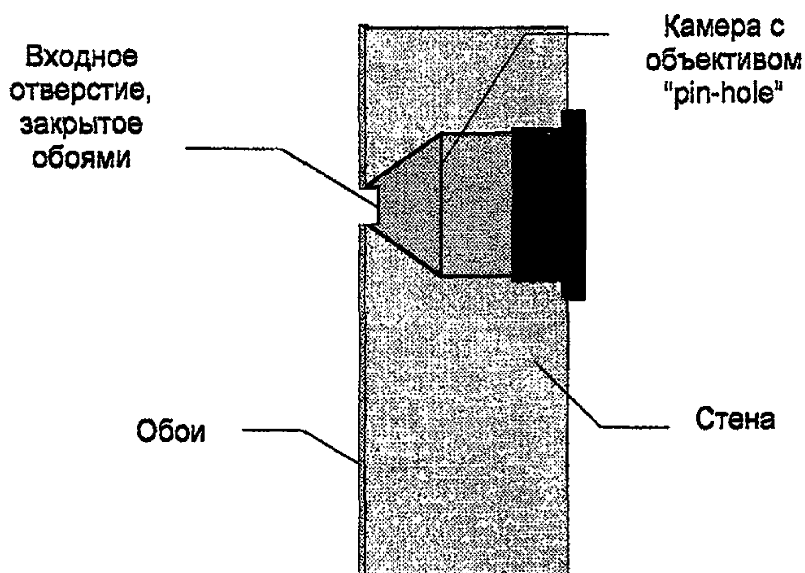
Рисунок 16 - Вариант установки видеоглазка в стене под обоями
