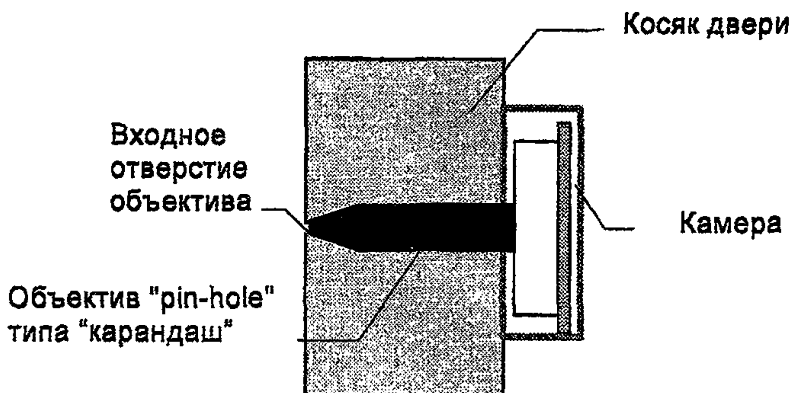
Рисунок 15 – Вариант установки видеоглазка в дверном косяке
