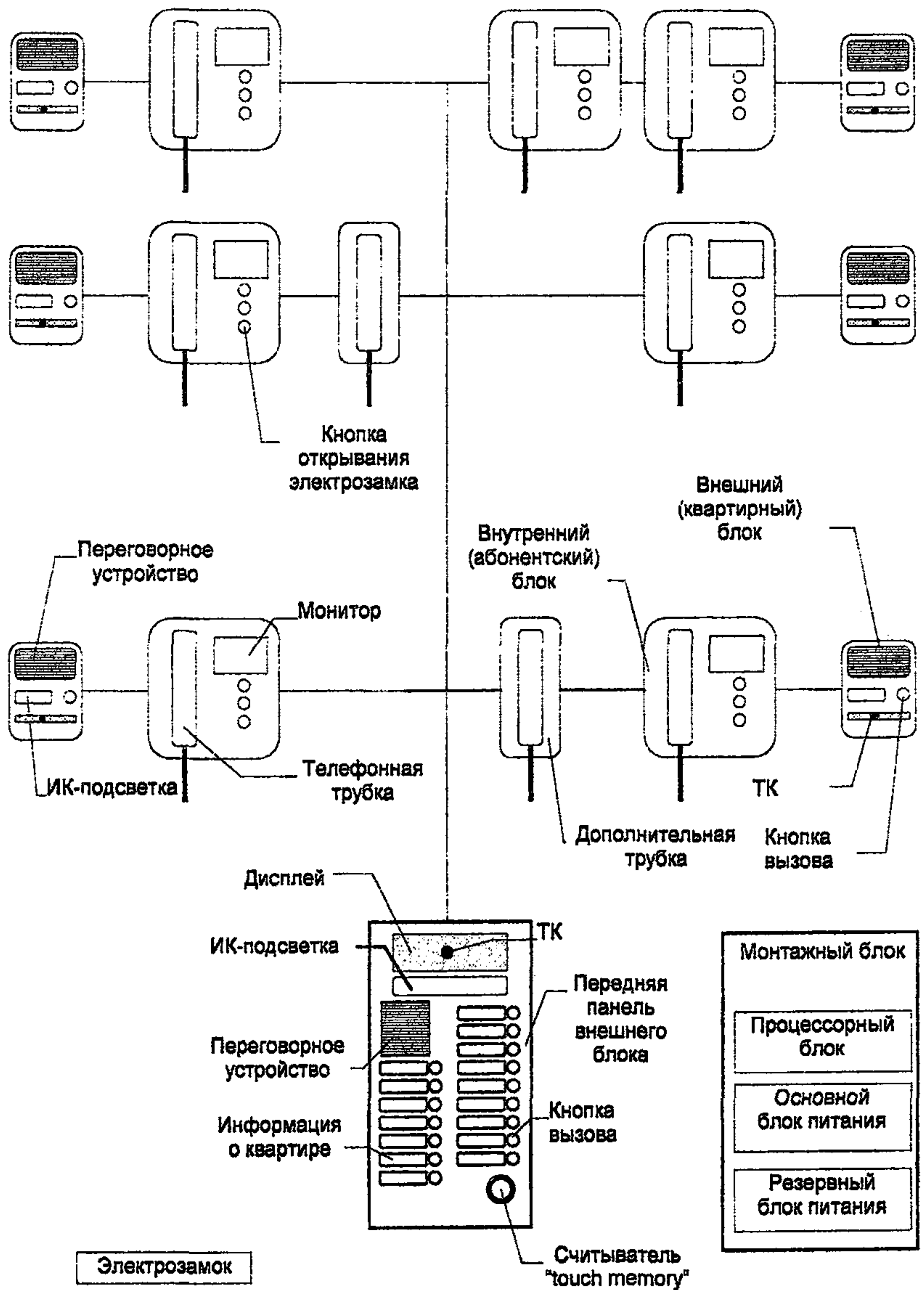
Рисунок 13 - Типовая конфигурация двухуровневого подъездного видеодомофона
