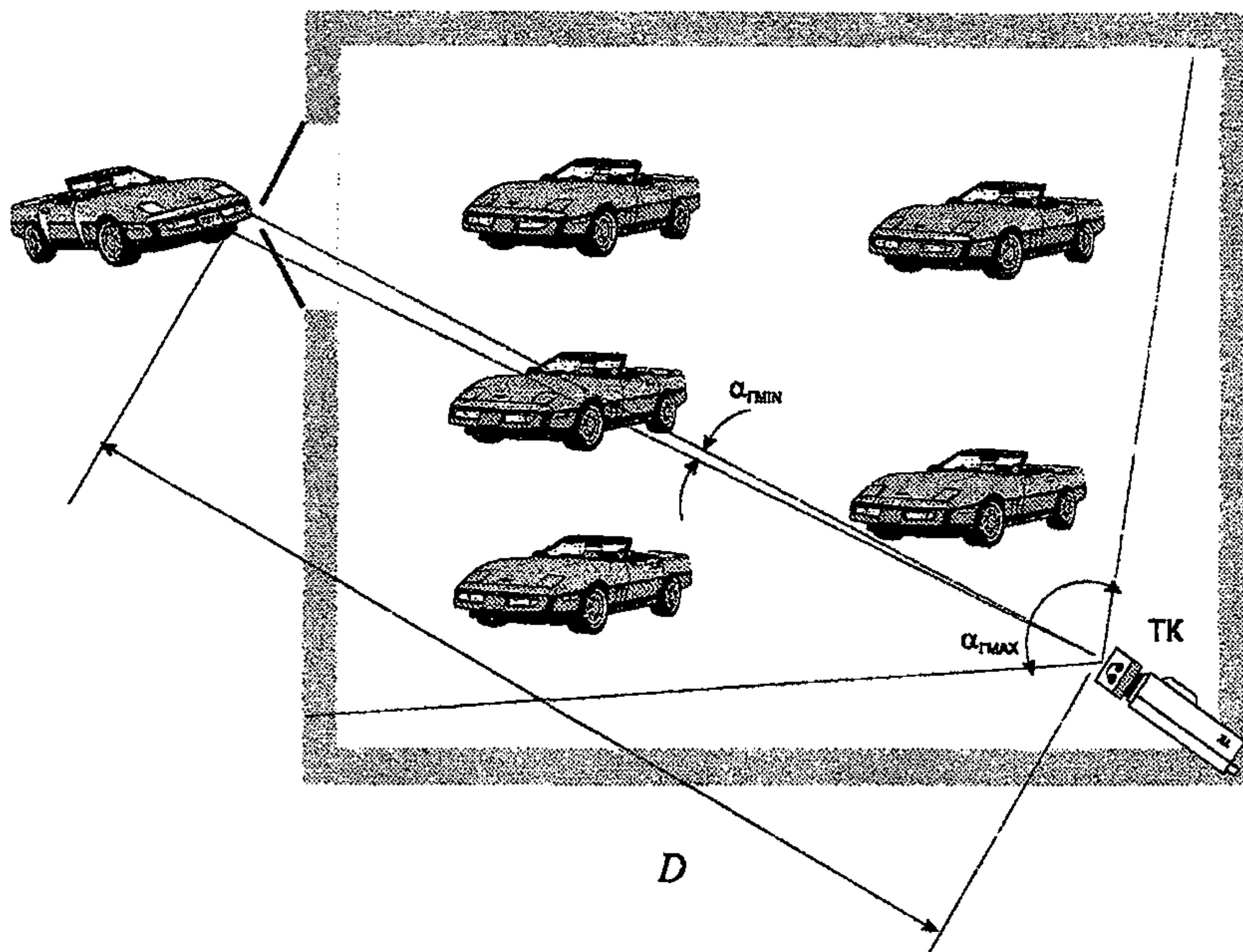
Рисунок 8 – Схема охраны стоянки автомобилей
