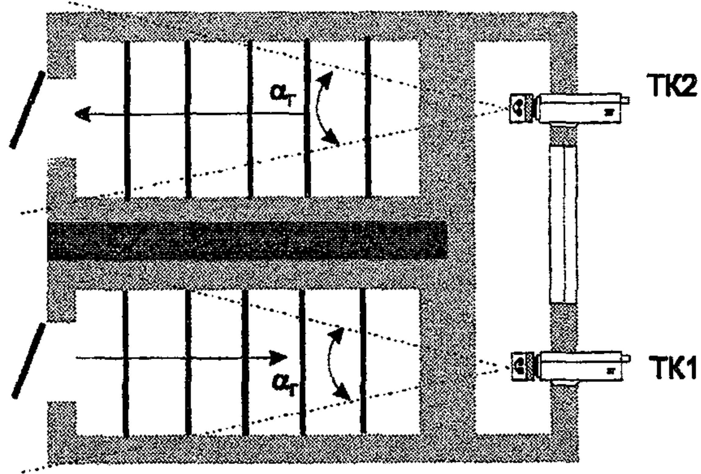
Рисунок 6 – Схемы охраны лестничных пролетов
