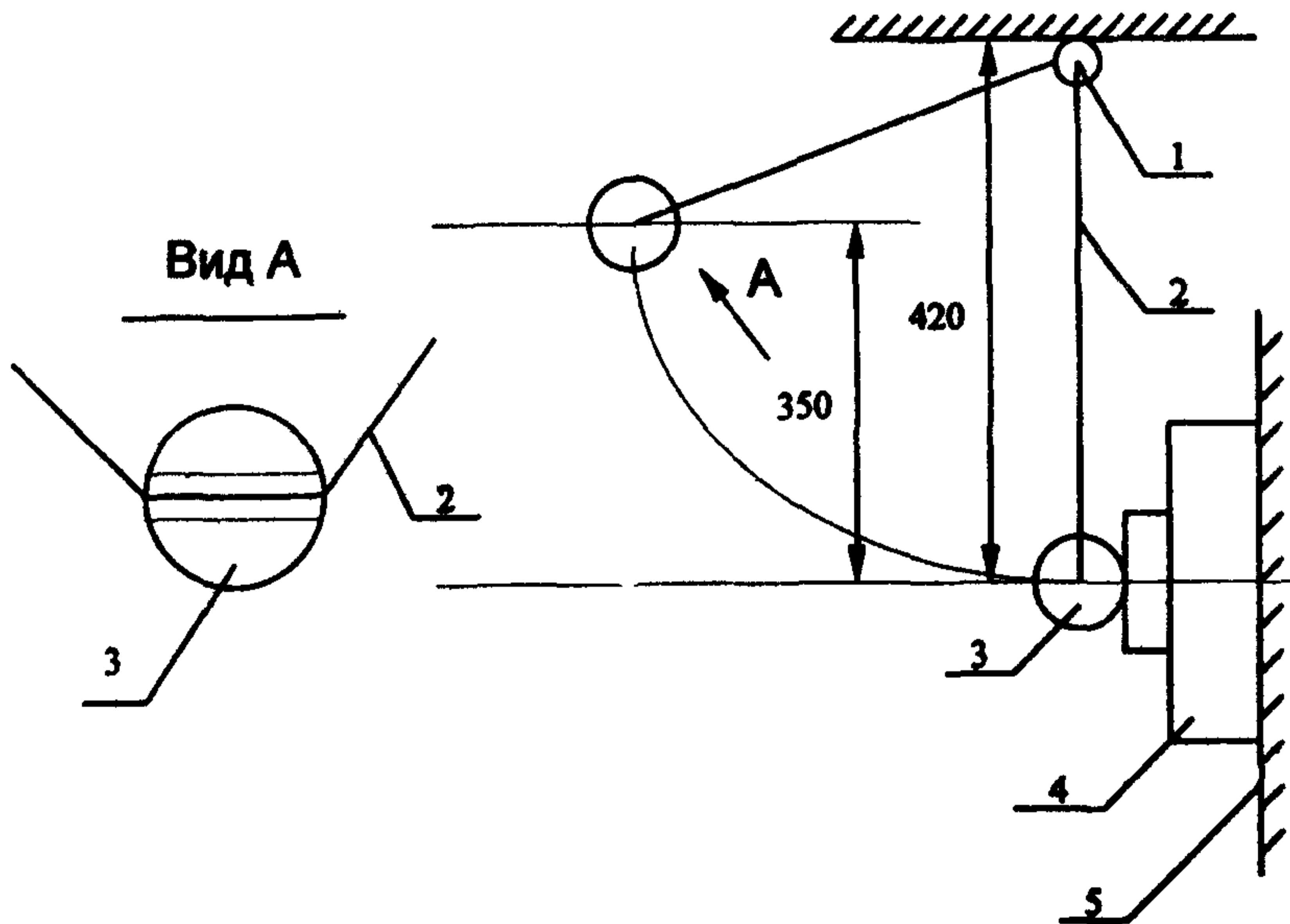
1 - горизонтальная штанга; 2 - нить маятника; 3 - латунный шар; 4 - испытуемый шар; 5 - опора
