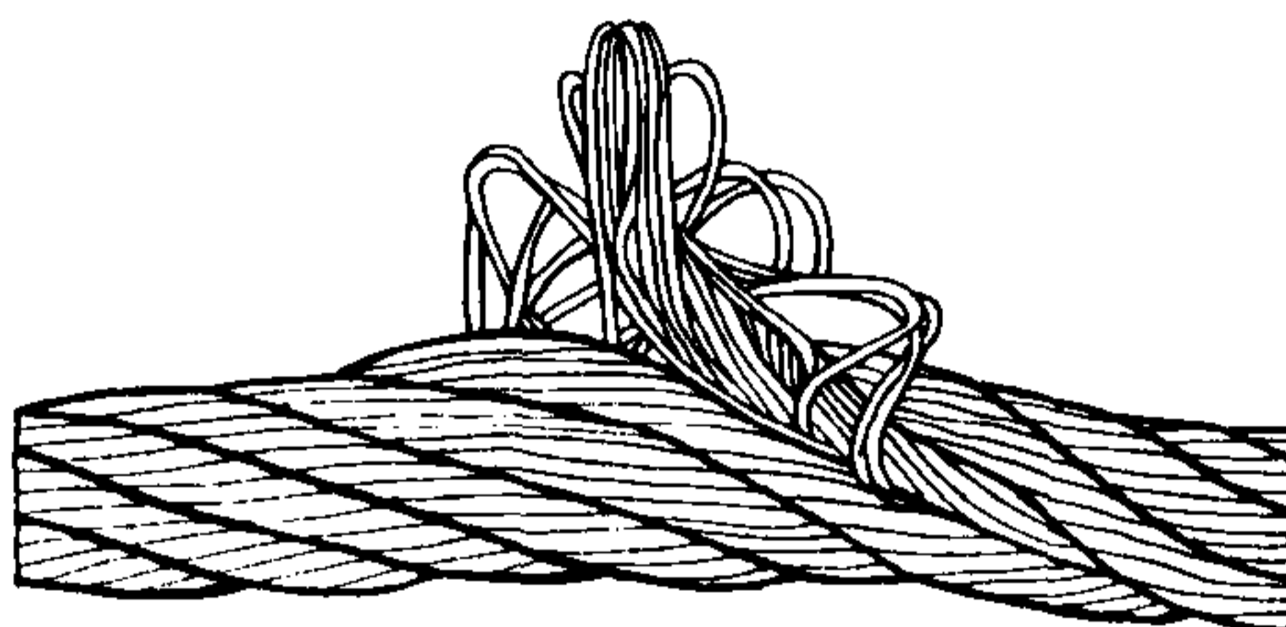
Рис. 10. Выдавливание сердечника
