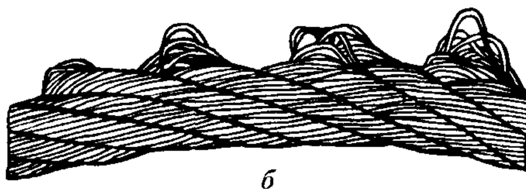
Рис. 11. Выдавливание проволок прядей: a — в одной пряди; б — в нескольких прядях
