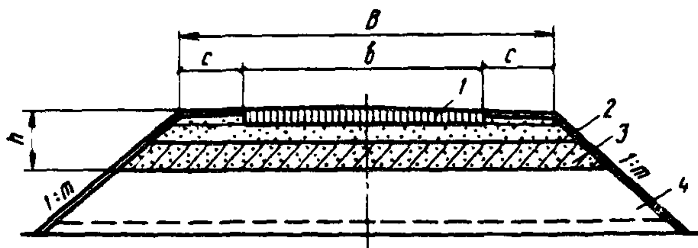
Рис.1. Конструкция насыпи из грунтов повышенной влажности с рабочим слоем из улучшенного грунта или обработанного золой уноса, известью, цементом; 1 - основание и покрытие; 2 - морозозащитный (дренирующий) слой (по расчету); 3 - рабочий слой из грунта с K_y = 1 \pm 0,98 ; 4 - тело насыпи из грунта повышенной влажности с K_y \geq 0,93
