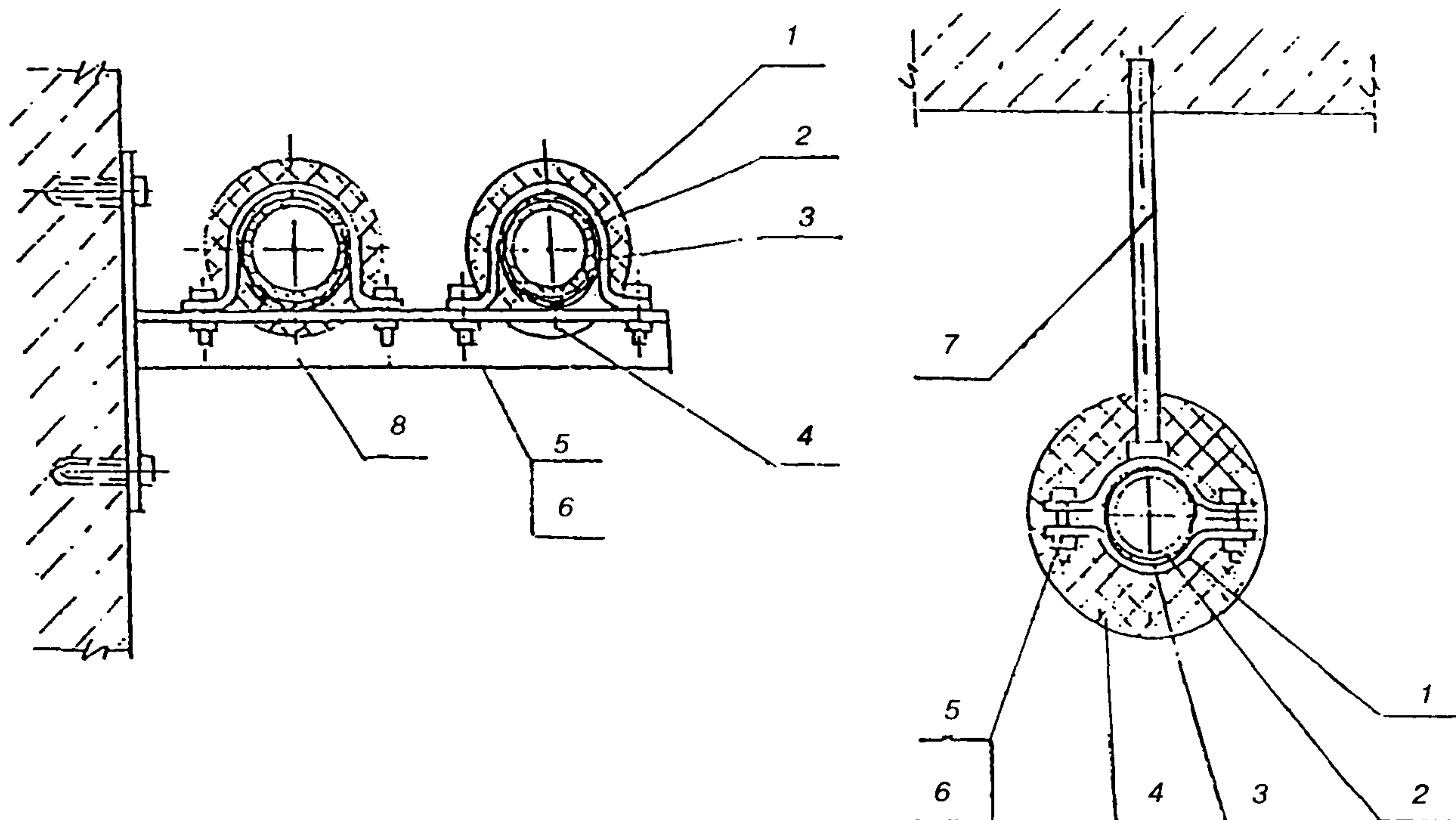
Рисунок 17 — Крепление труб к стенам и перегородкам
