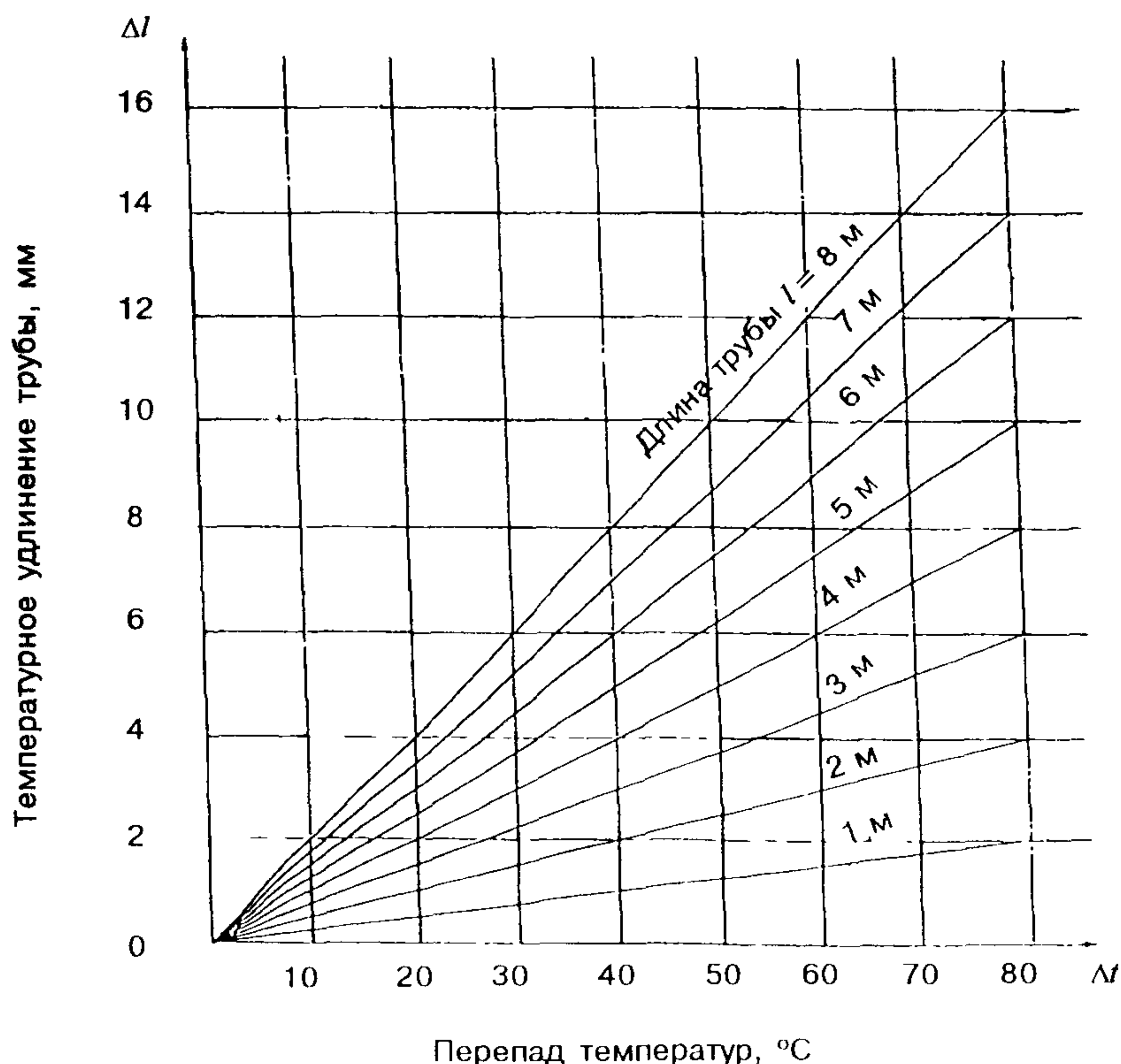
Рисунок 10 — Диаграмма для определения удлинения труб
