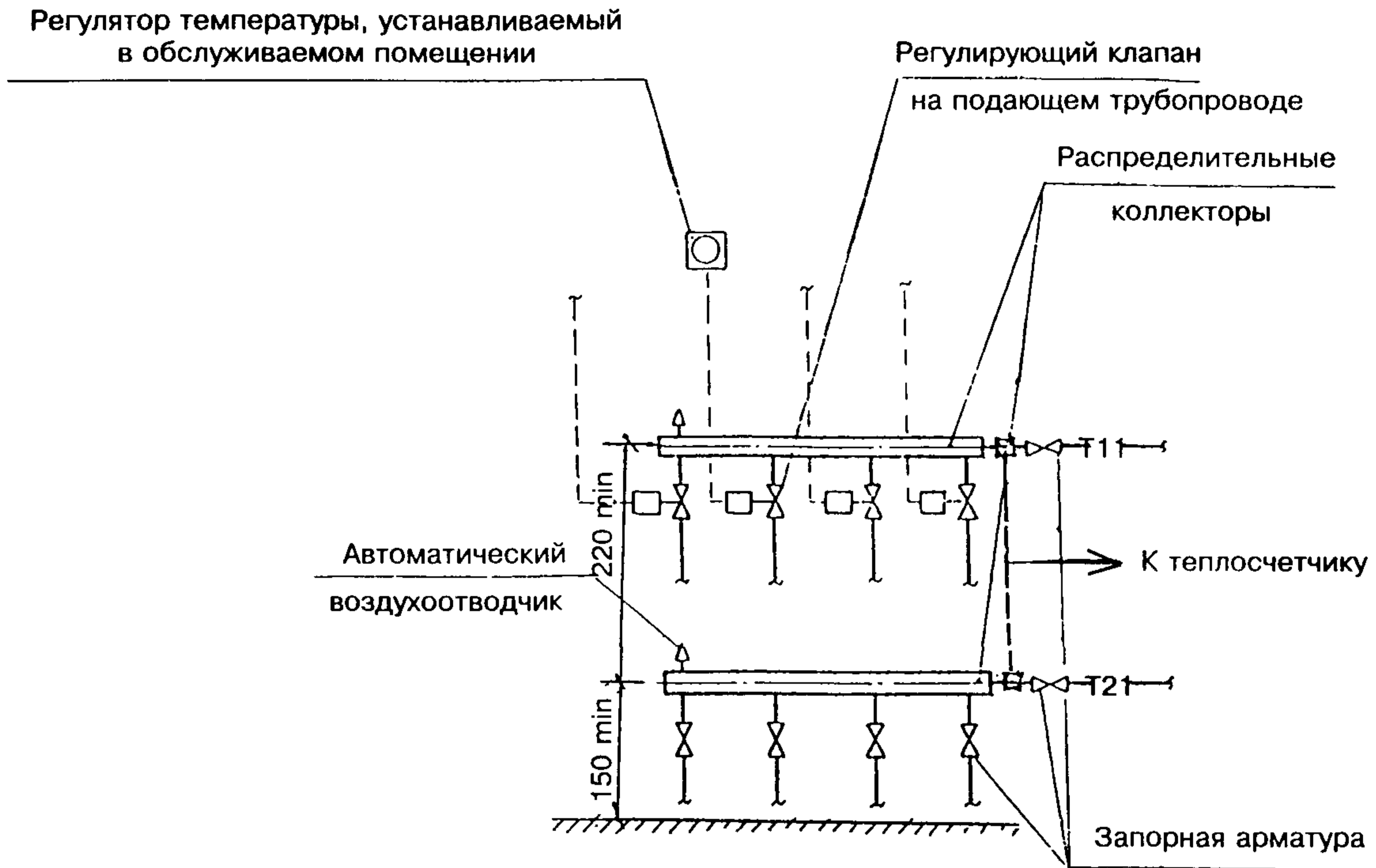
Рисунок 7 — Распределительный коллектор системы отопления
