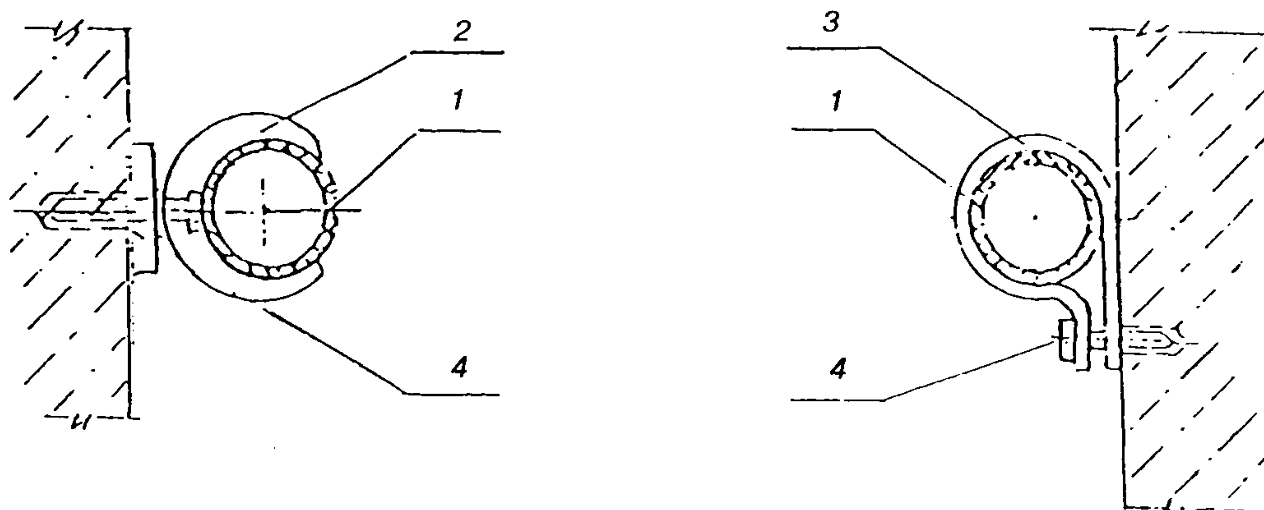
Рисунок 17 — Крепление труб к стенам и перегородкам
