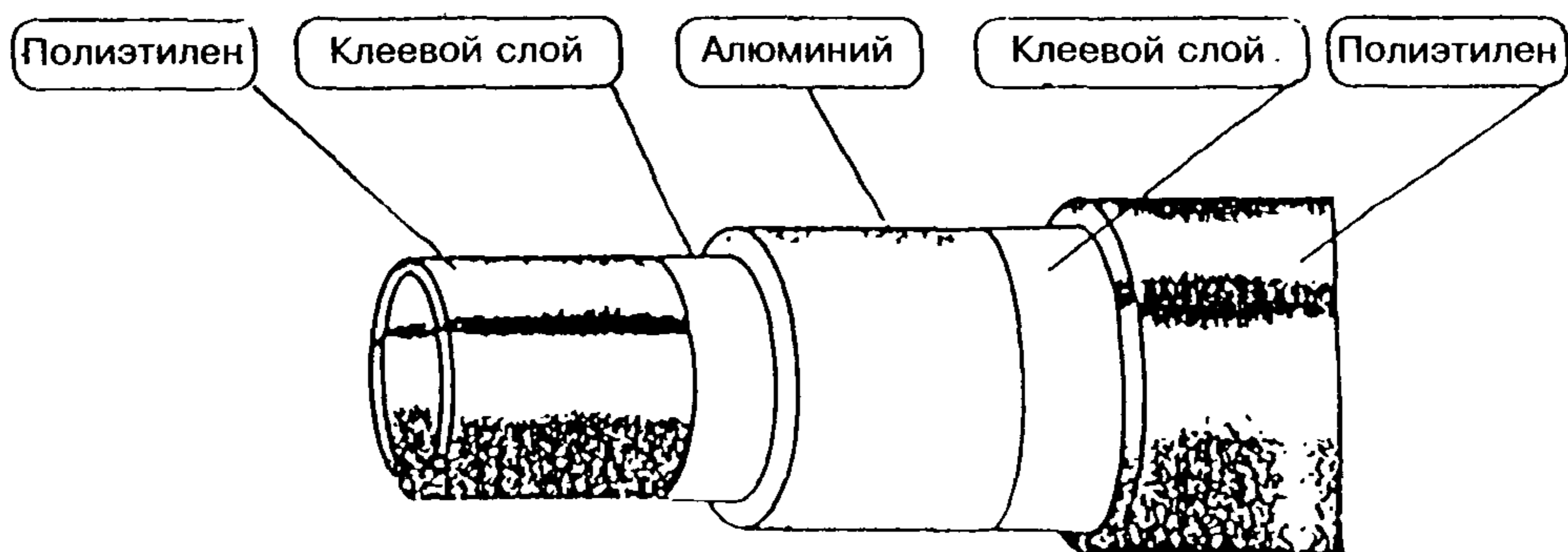
Рисунок 1 — Структура металлополимерной трубы
