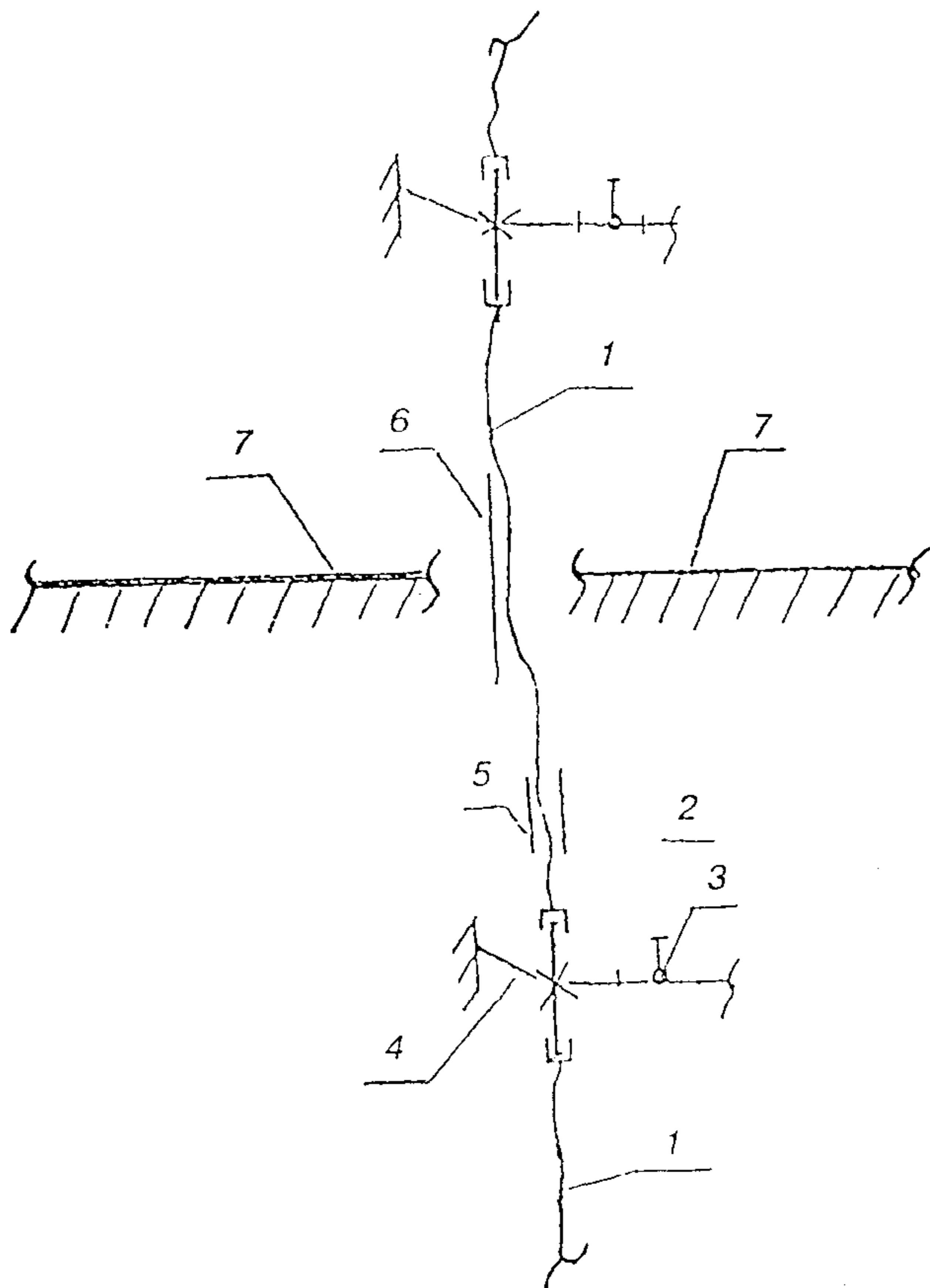
1 — междуэтажная вставка из МПТ 2025; 2 — латунный тройник; 3 — вентиль; 4 — неподвижное крепление; 5 — подвижное крепление; 6 — гильза; 7 — междуэтажное перекрытие
