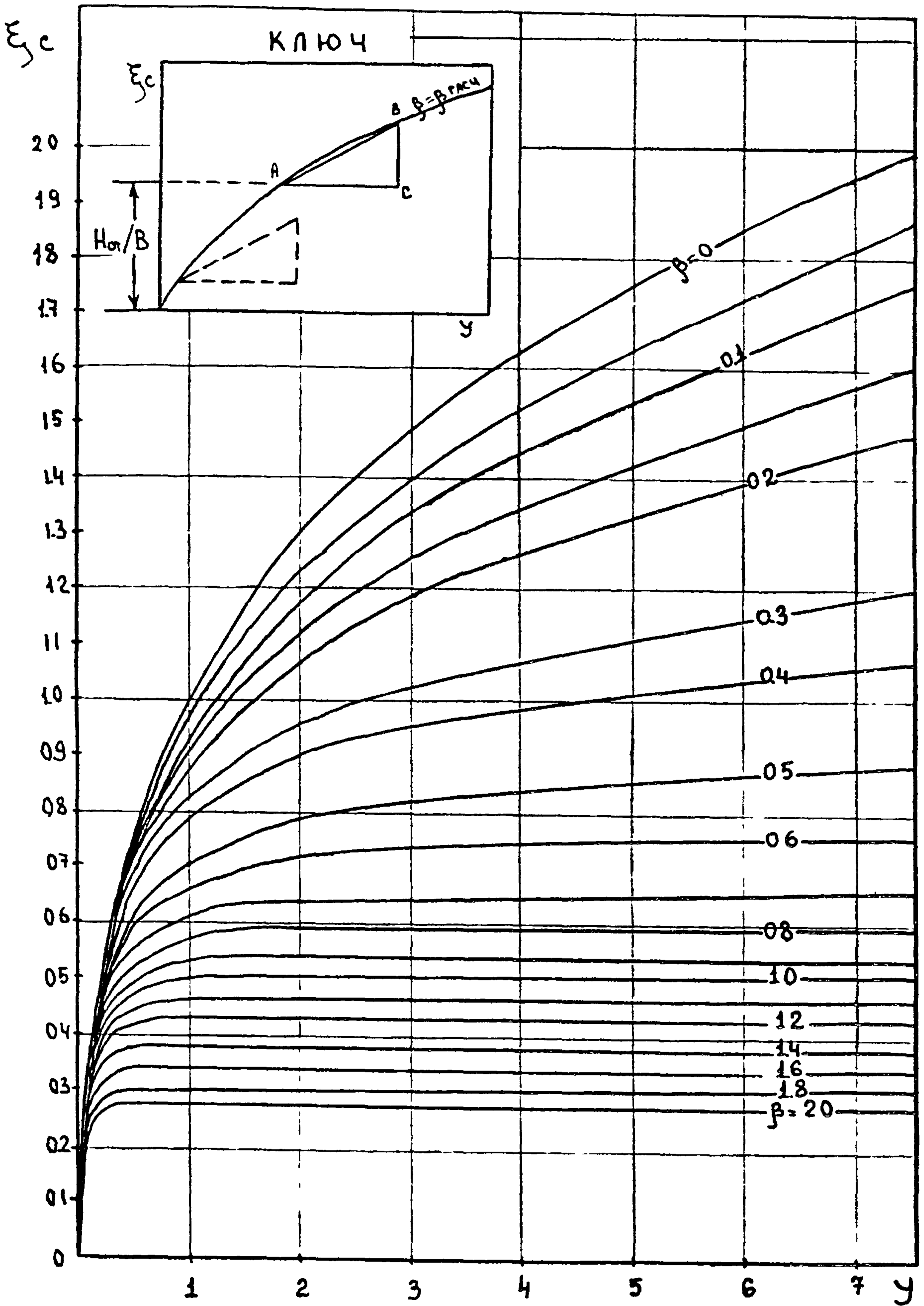
Рис. 3.1 Номограмма для определения H_{\sigma}/B Примечание: является известной номограммой \xi_c = f(\gamma) СНИП П-18-76, в которой логарифмическая шкала \gamma заменена равномерной и продлена до 7.
