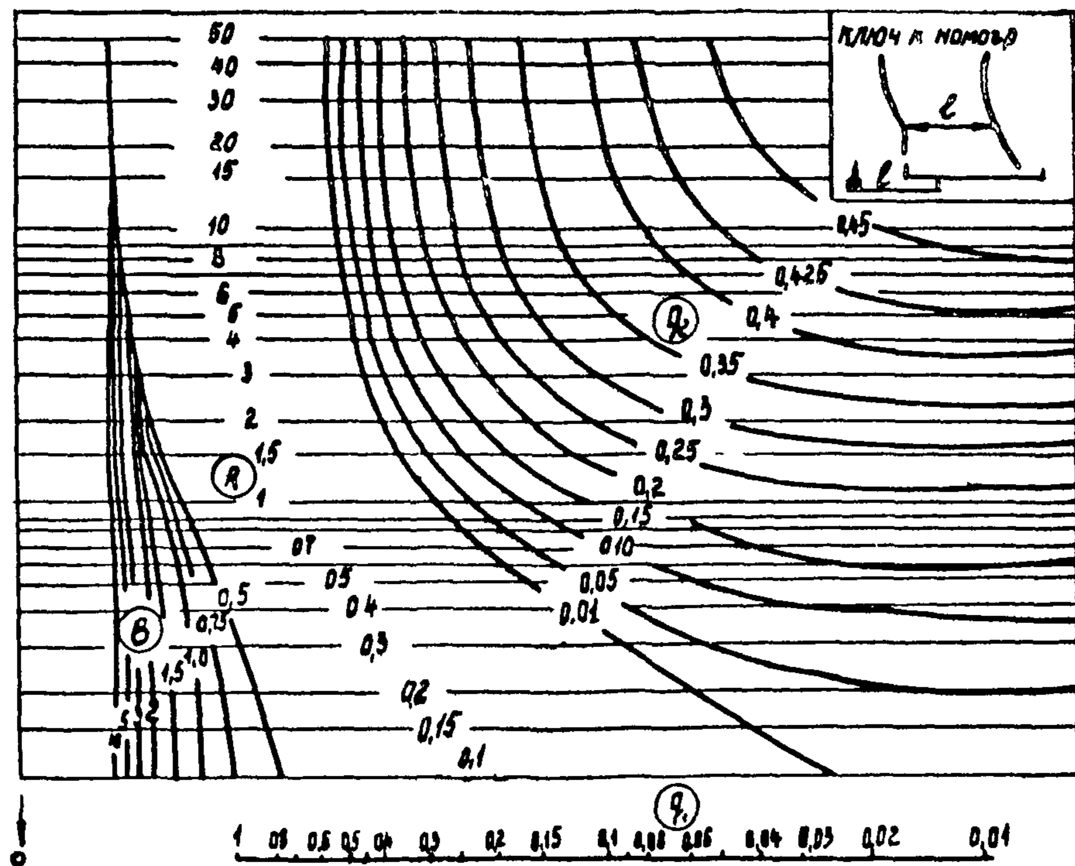
Рис 3.2 Номограмма для определения R
