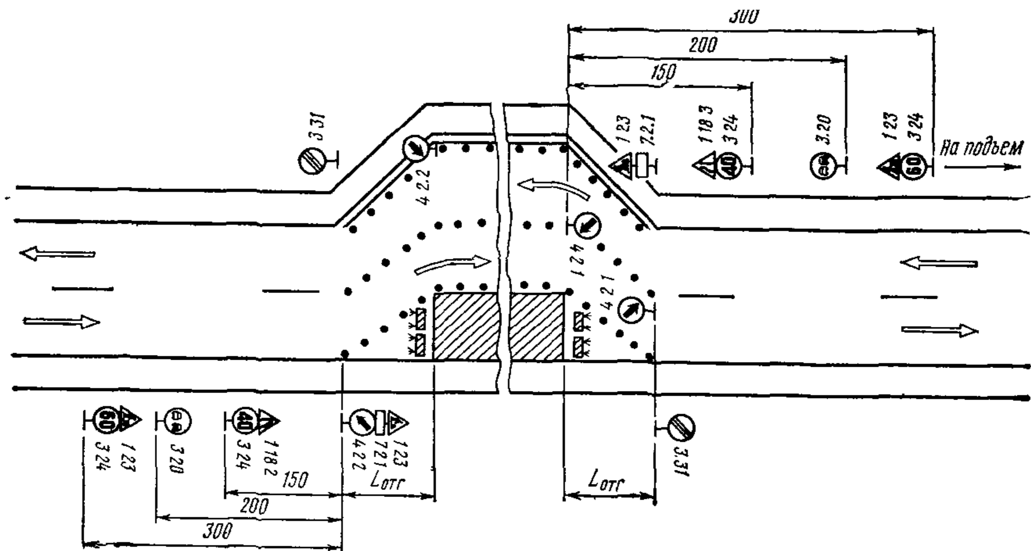
Рис. 3.9. Организация движения и ограждение места дорожных работ в случае уширения проезжей части на участках затяжных подъемов двухполосных дорог
