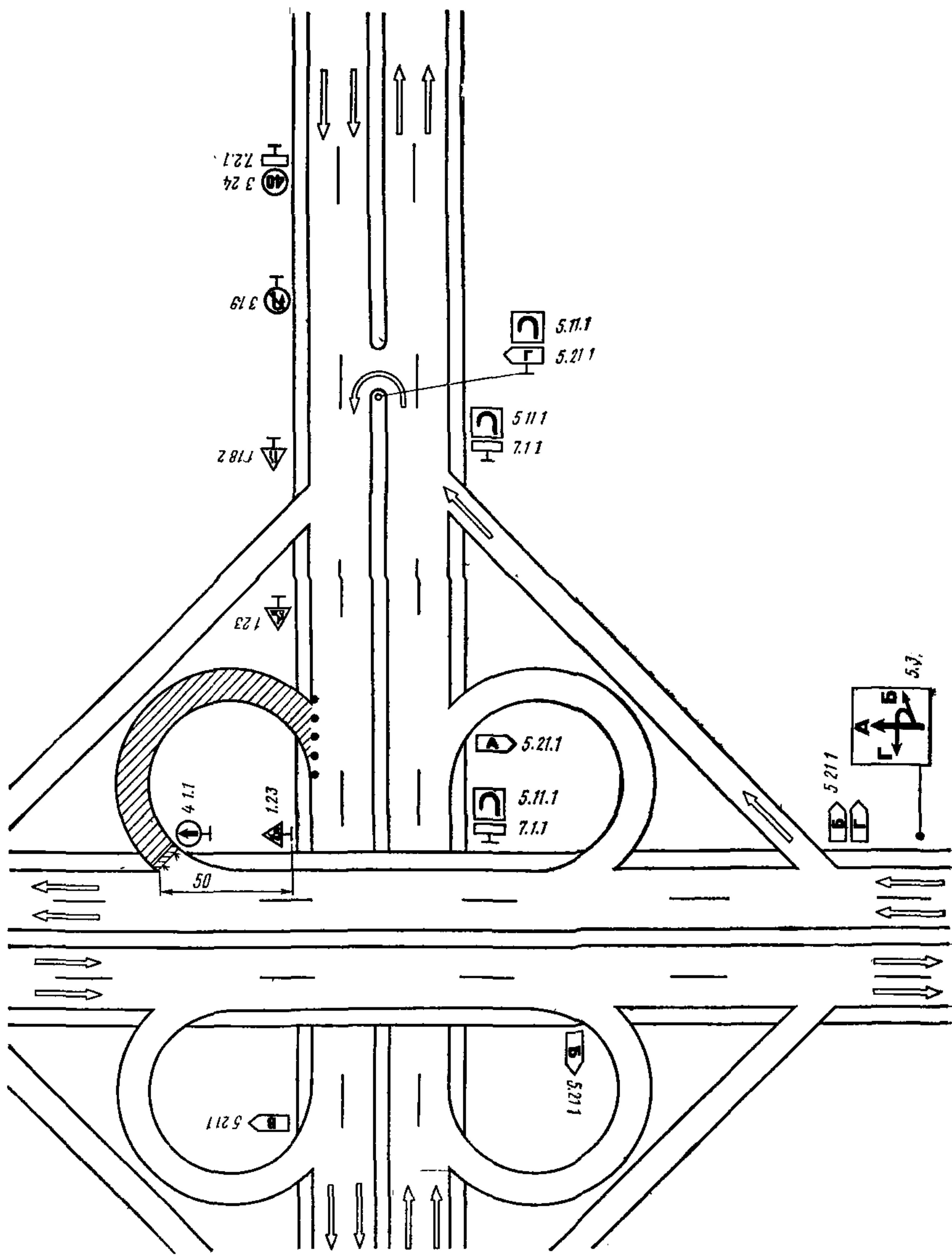
Рис. 3.23. Организация движения и ограждение места дорожных работ при закрытии левоповоротного съезда пересечения в разных уровнях с устройством разворота на одной из дорог
