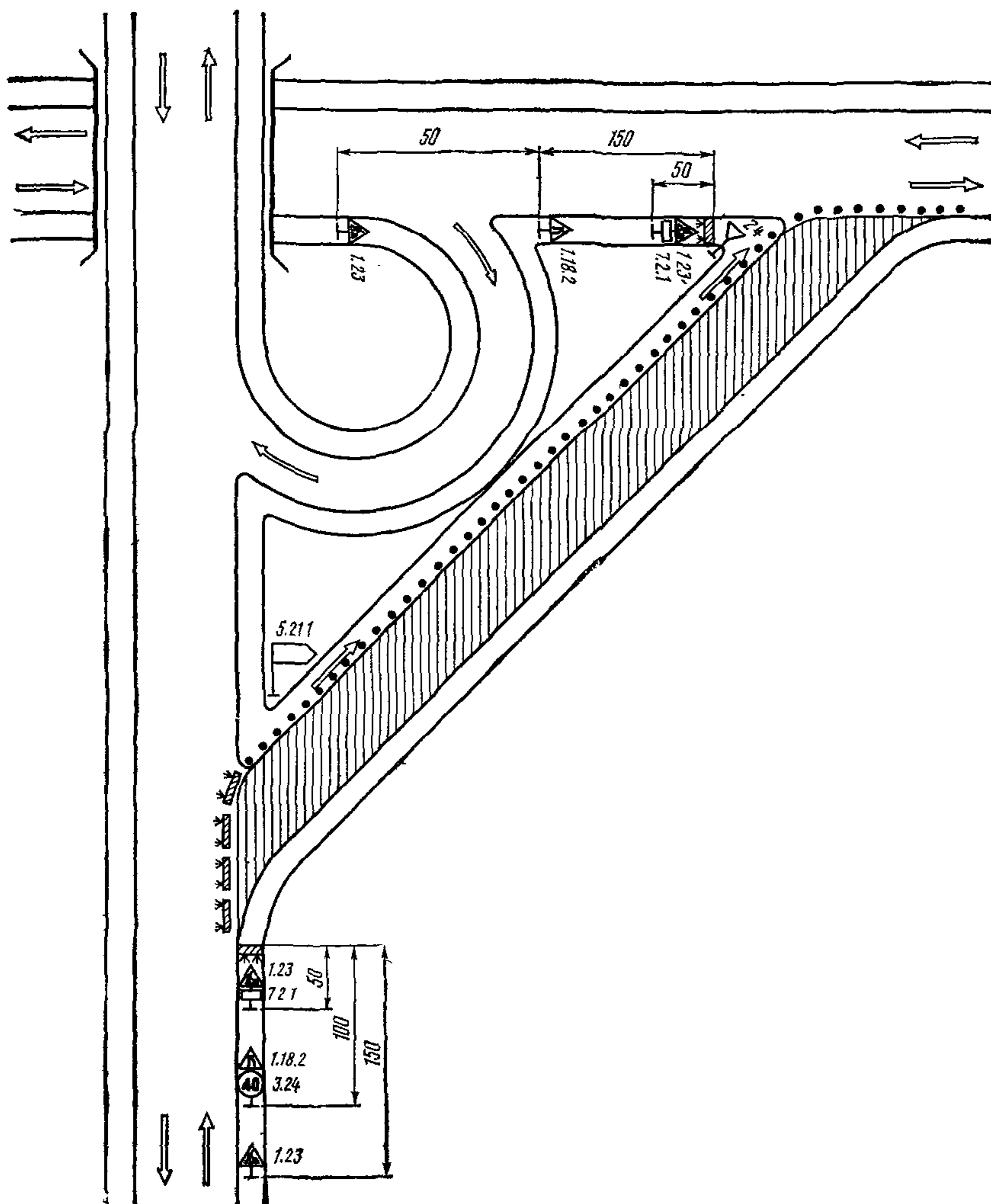
Рис. 3.19. Организация движения по обочине и ограждению места дорожных работ, выполняемых на всей ширине проезжей части правоповоротного съезда пересечения в разных уровнях
