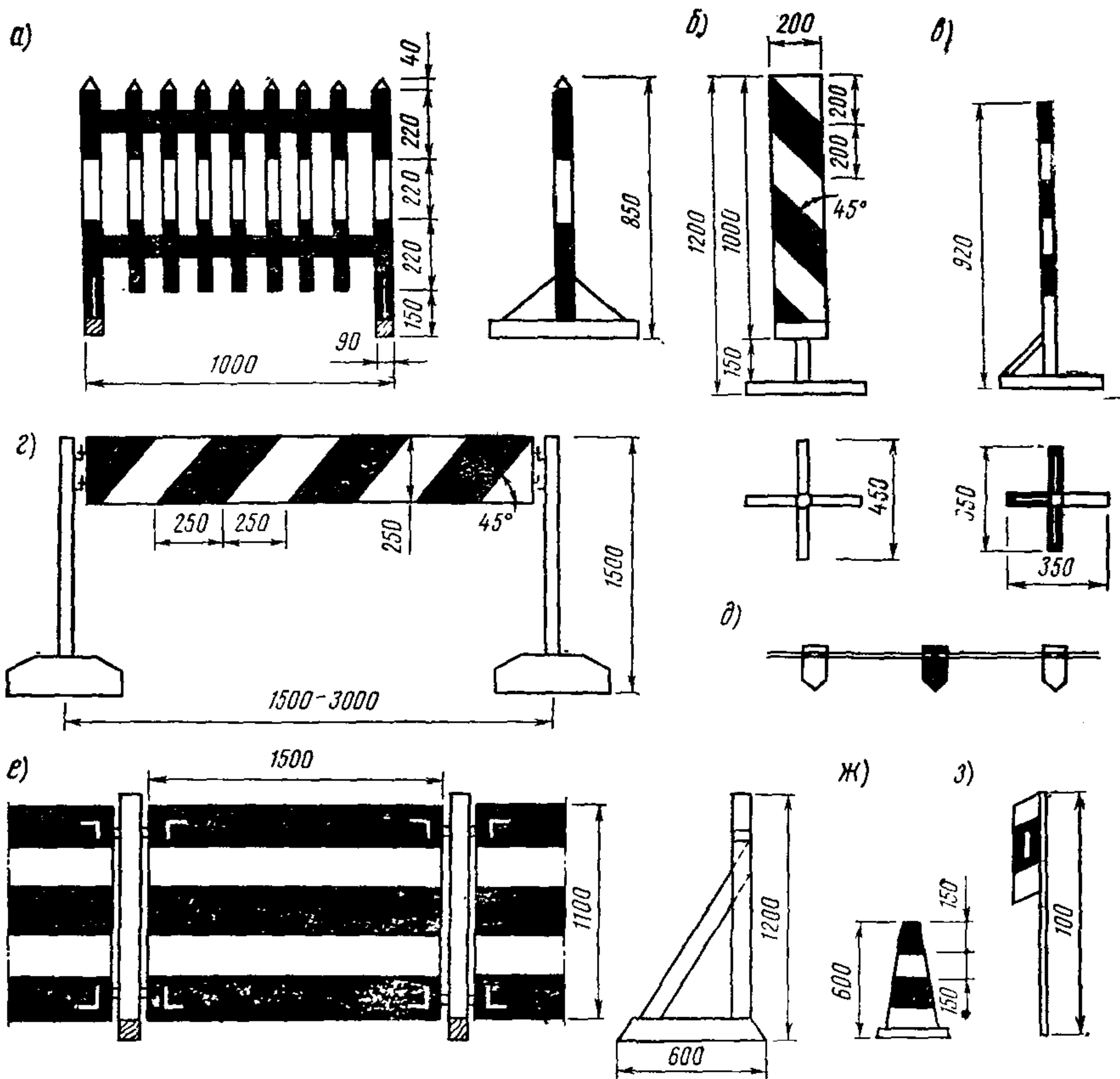
Рис. 4.2. Ограждения и направляющие устройства:
