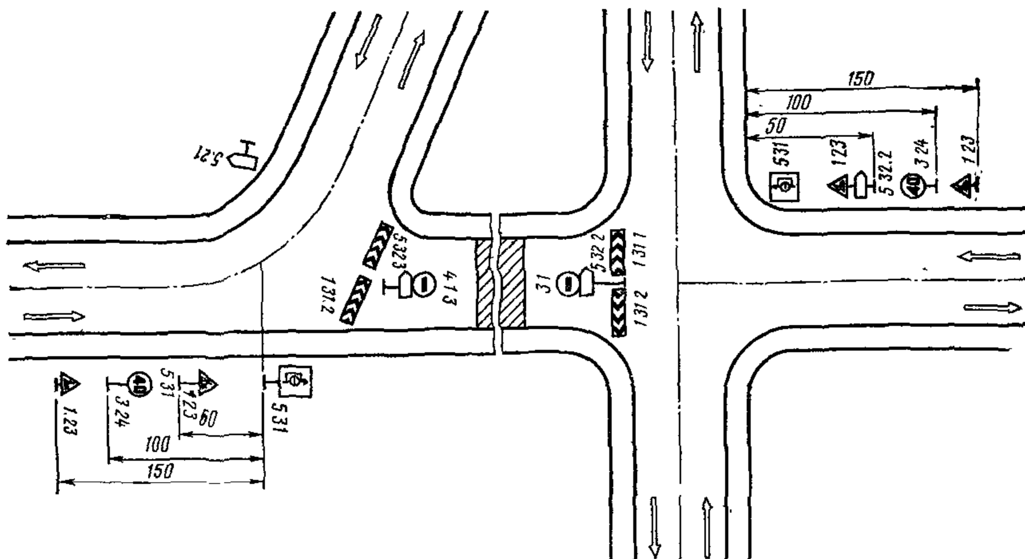
Рис. 3.30. Организация движения при производстве дорожных работ на всей ширине проезжей части и направлением потока транспорта в объезд по существующим дорогам
