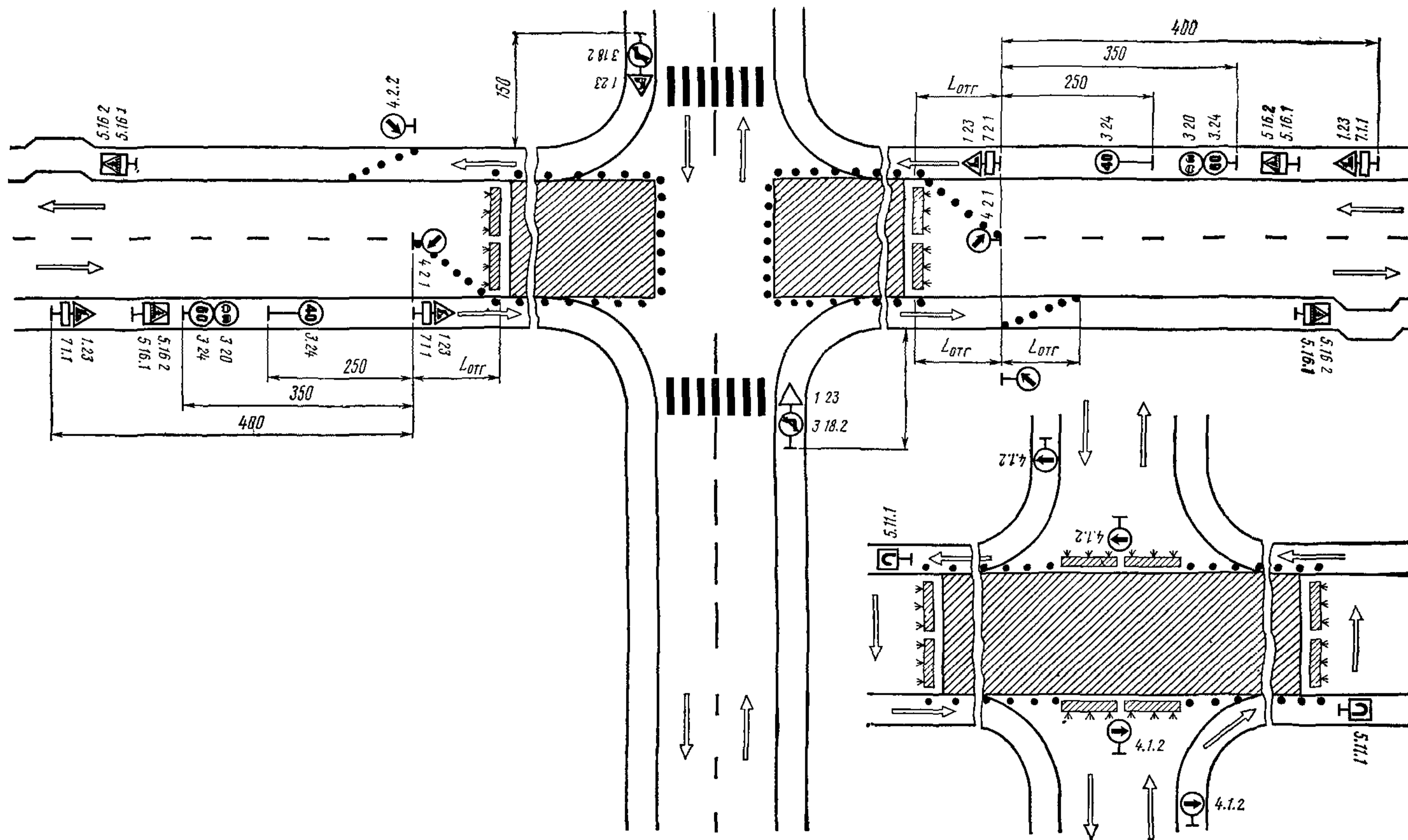
Рис. 3.16. Организация движения и ограждение мест дорожных работ, выполняемых на проезжей части главной дороги: I — пропуск транспорта в объезд ремонтируемого участка по обочинам главной дороги
