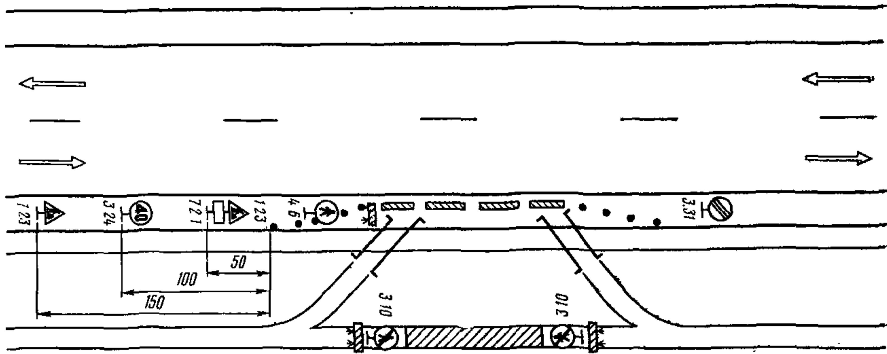
Рис. 3.25. Организация движения и ограждение места производства дорожных работ на пешеходной или велосипедной дорожке
