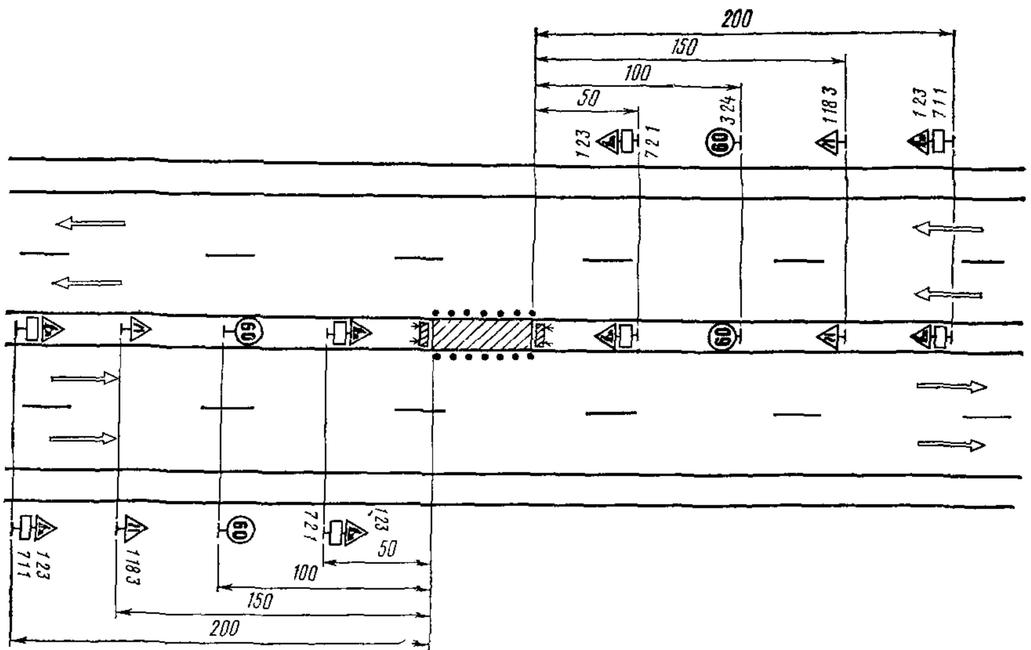
Рис. 3.7. Организация движения и ограждение мест дорожных работ, выполняемых на разделительной полосе многополосных дорог
