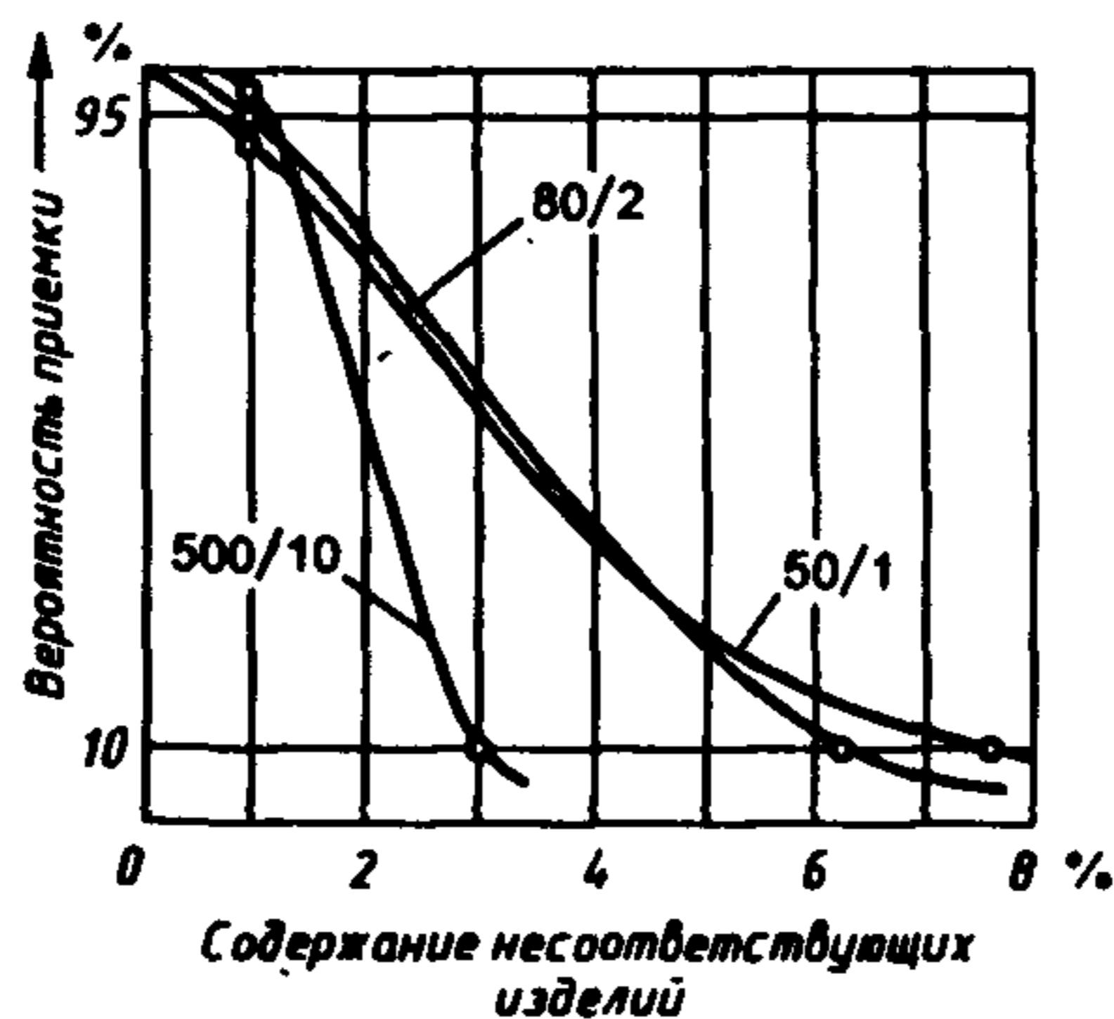
Кривые оперативных характеристик для планов выборочного контроля
