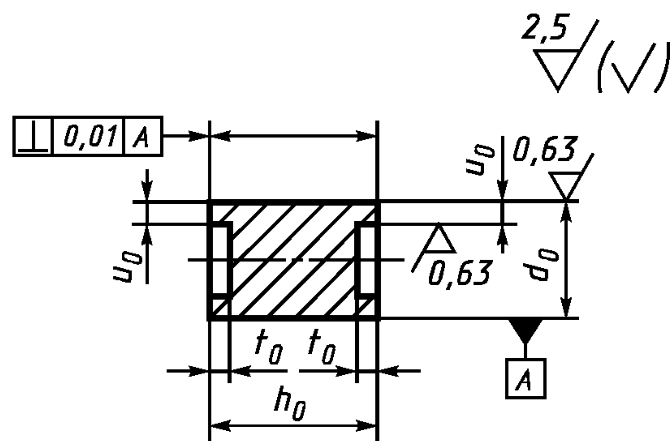
Рисунок 2 — Экспериментальные образцы IV типа
