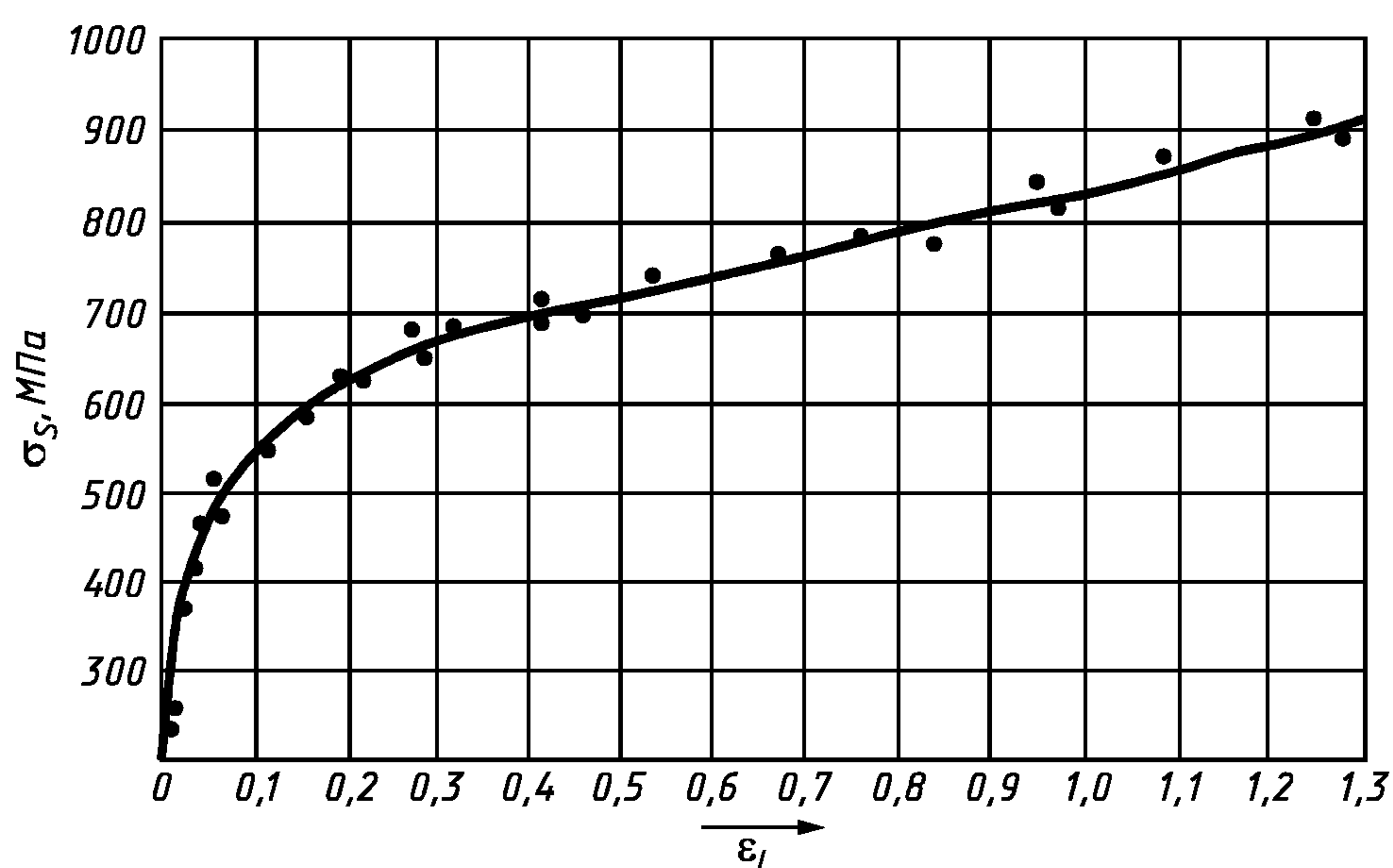
Рисунок 9 — Экспериментальная кривая упрочнения в координатах \sigma_s - \varepsilon_l
