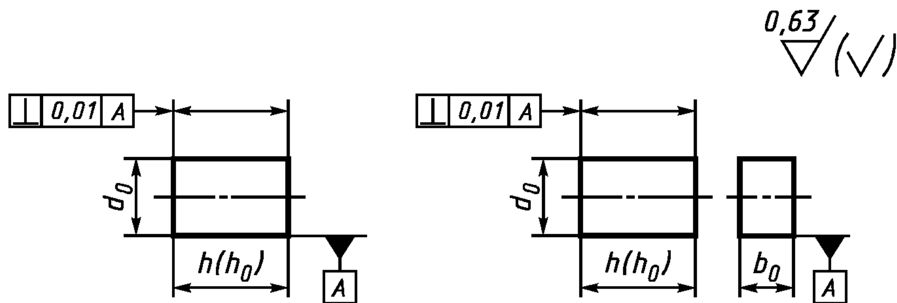
Рисунок 1 — Экспериментальные образцы I—III типов
