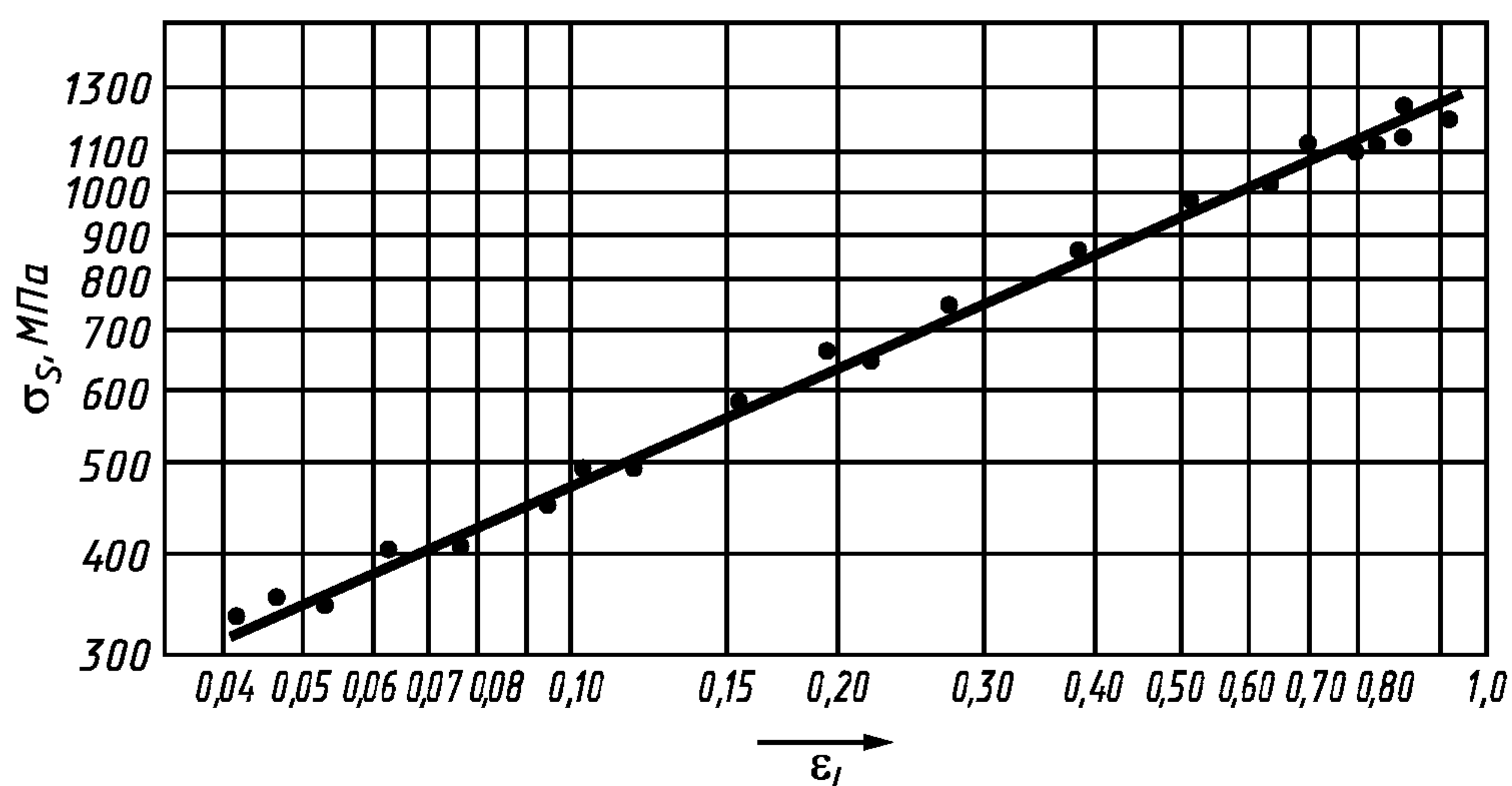
Рисунок 10 — Экспериментальная кривая упрочнения в логарифмических координатах
