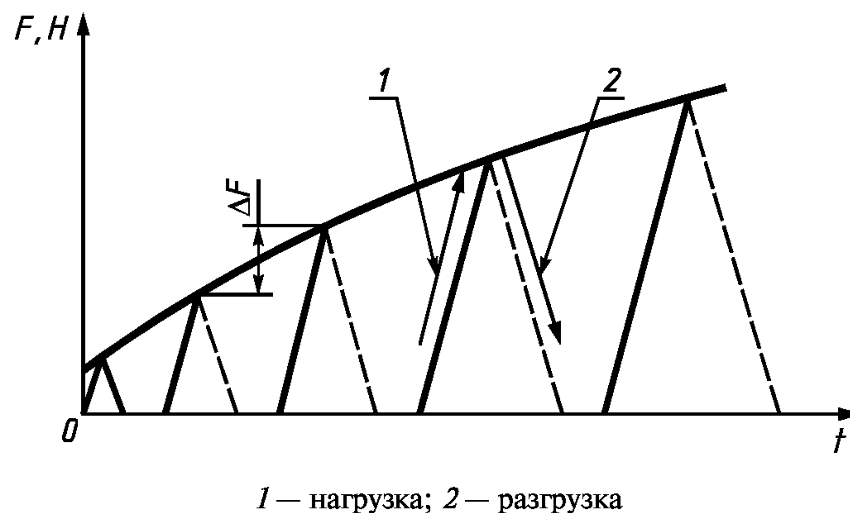
Рисунок 11 — Проведение испытаний при ступенчатом увеличении нагрузки
