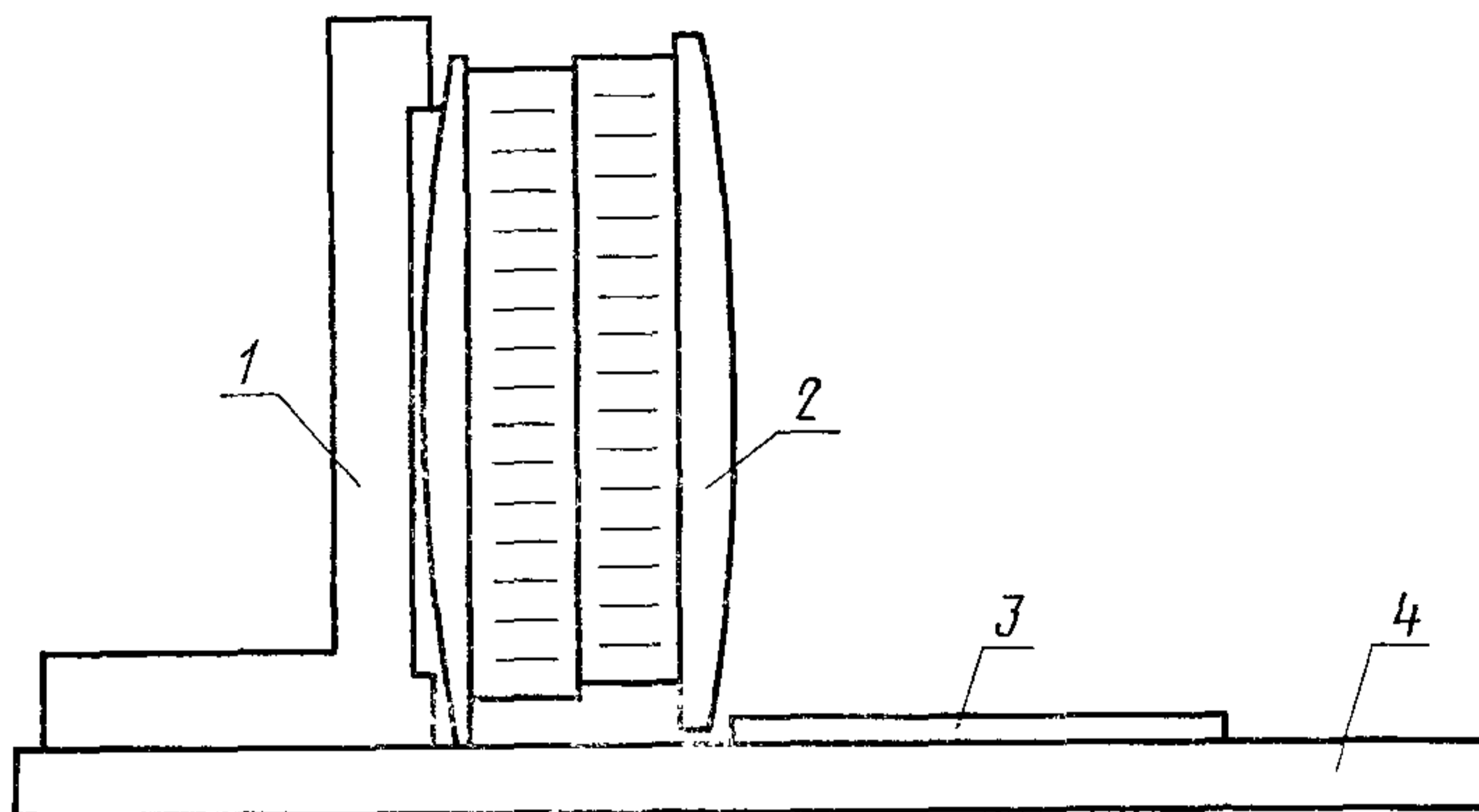
1—угловая плита; 2—блок; 3—щуп; 4—поверочная плита
