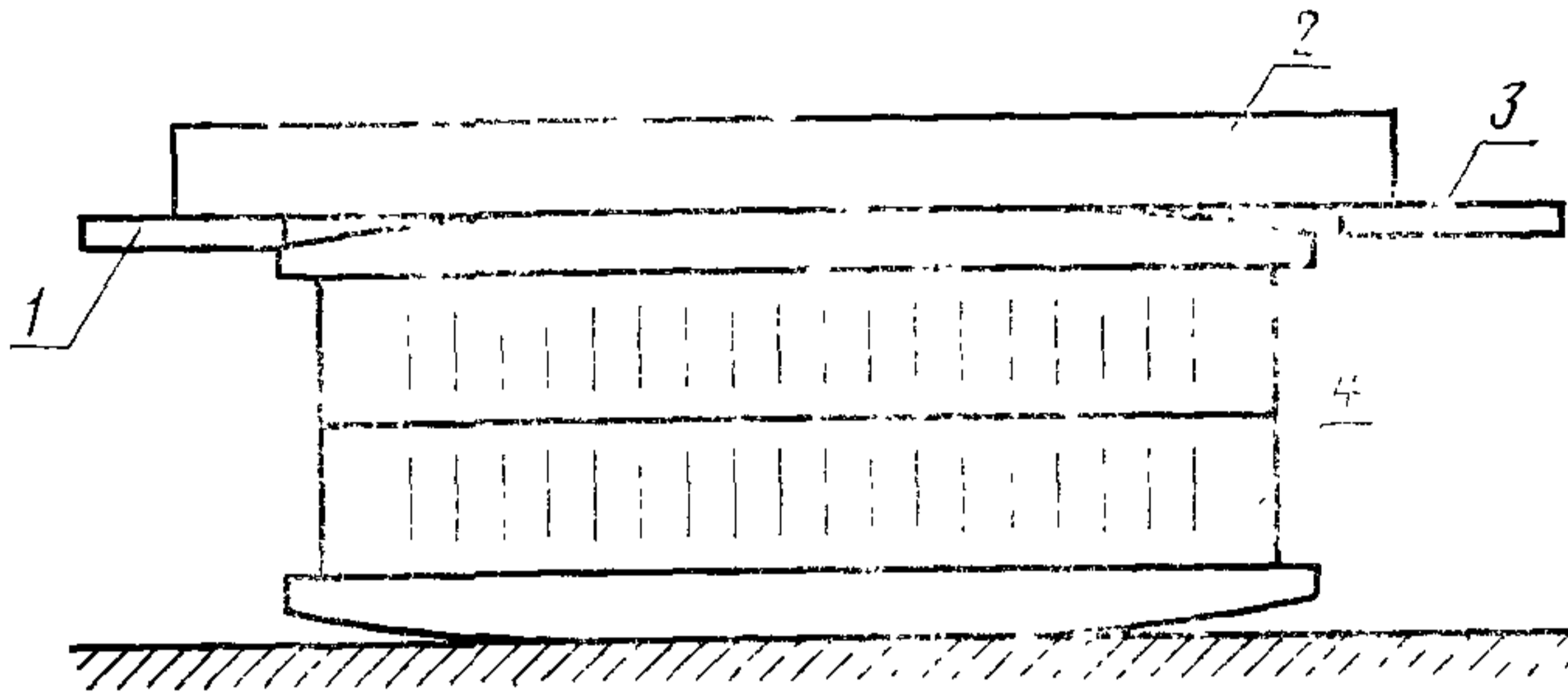
1 — щуп первый; 2 — поверочная линейка; 3 — щуп второй; 4 — блок
