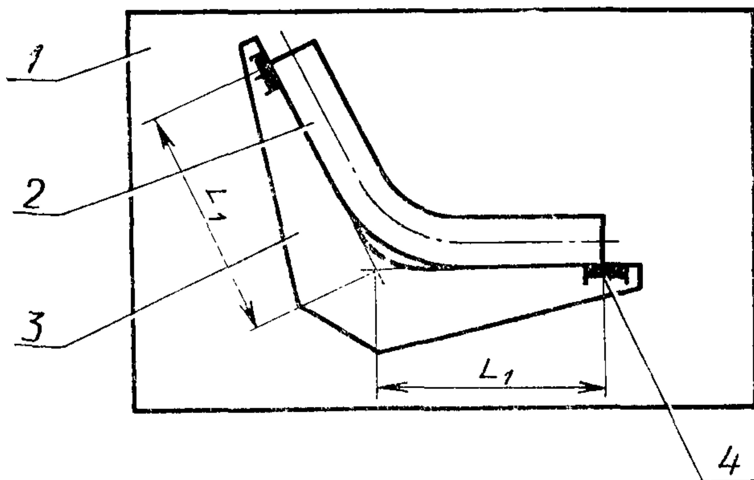
1—контрольная плита; 2—изделие; 3—шаблон; 4—поле допуска
