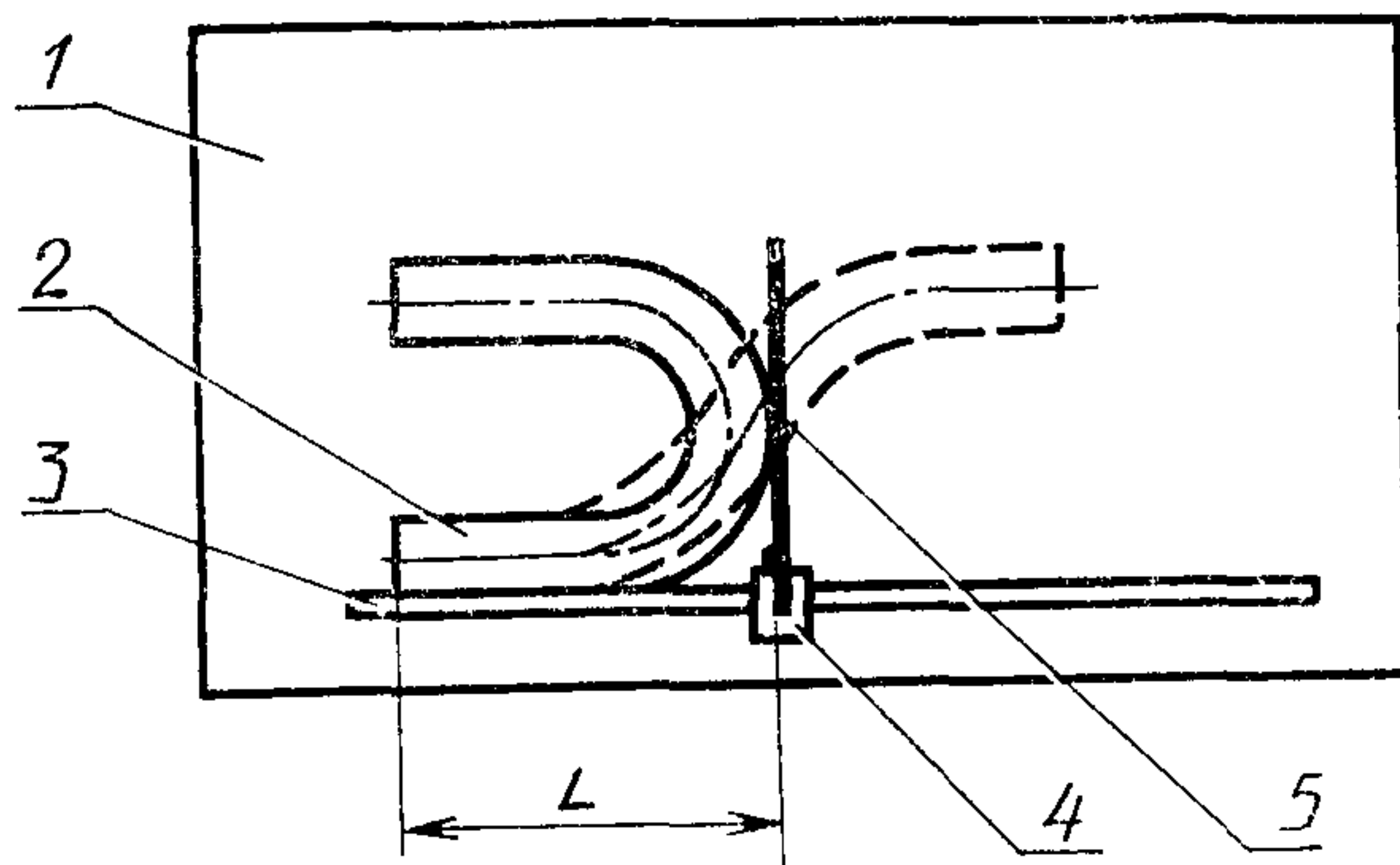
1—контрольная плита; 2—изделие; 3—контрольная линейка; 4—ползун; 5—упор
