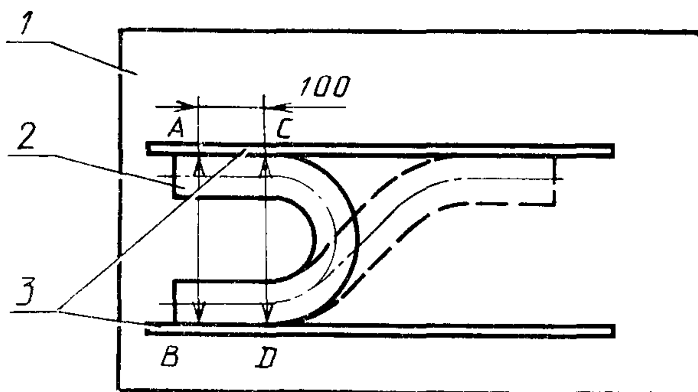
1—контрольная плита; 2—изделие, 3—поверочные линейки Черт. 16
