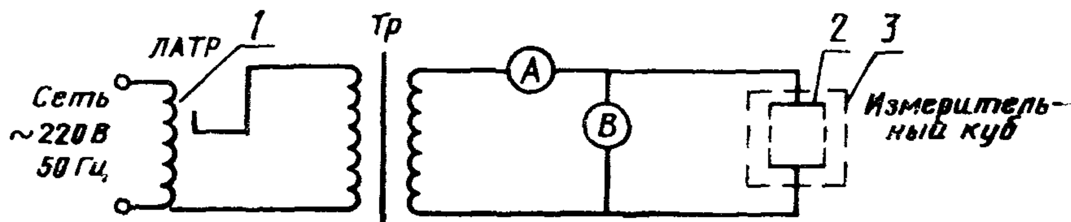
1—лабораторный регулировочный трансформатор (ЛАТР); 2—электрод; 3—измерительный куб
