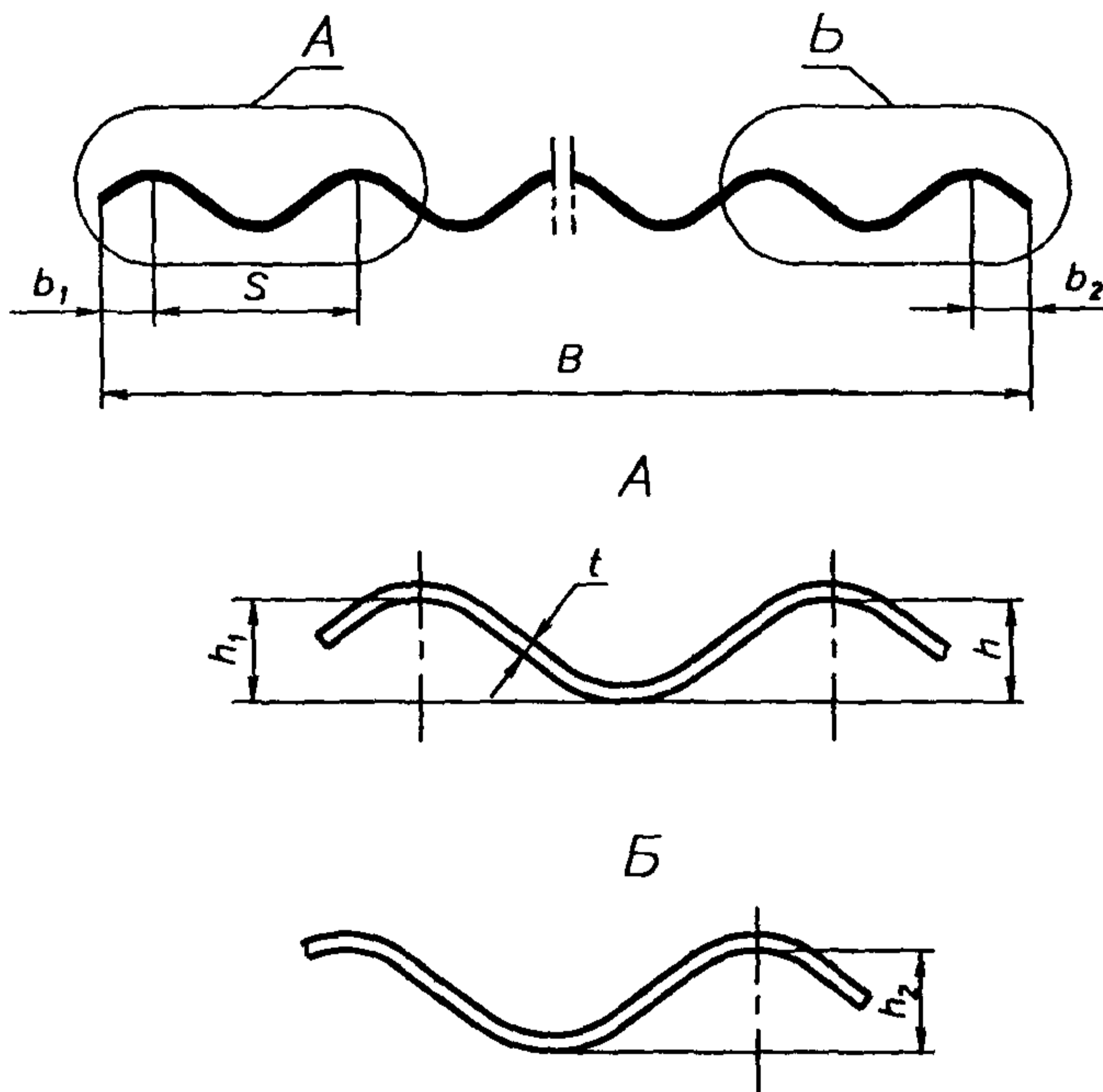
Рисунок 1 — Форма поперечного сечения волнистого листа
