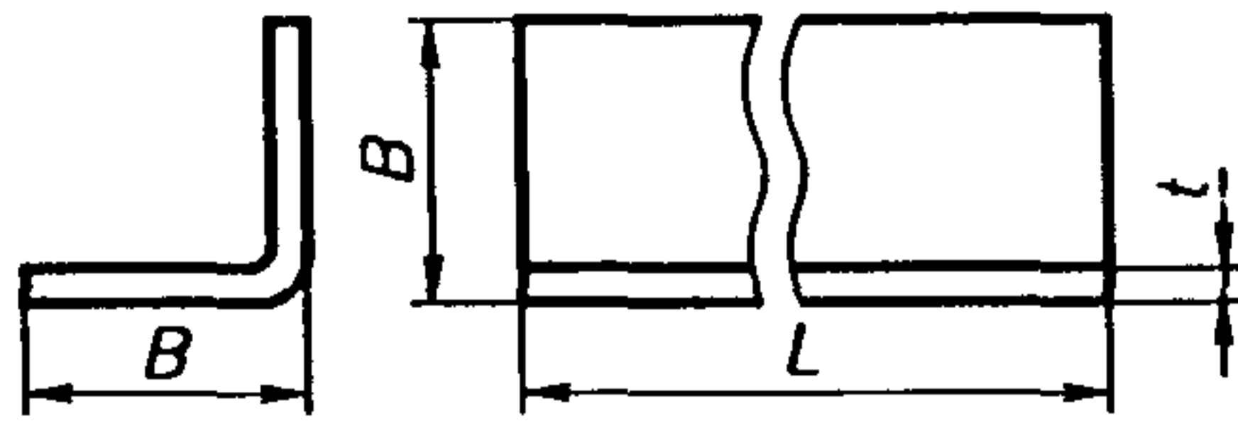
Рисунок 4 — Равнобокая угловая деталь
