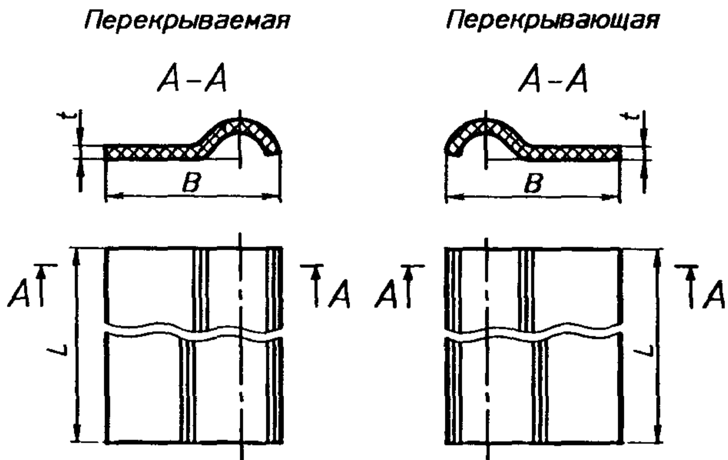
Рисунок 3 — Упрощенные коньковые детали
