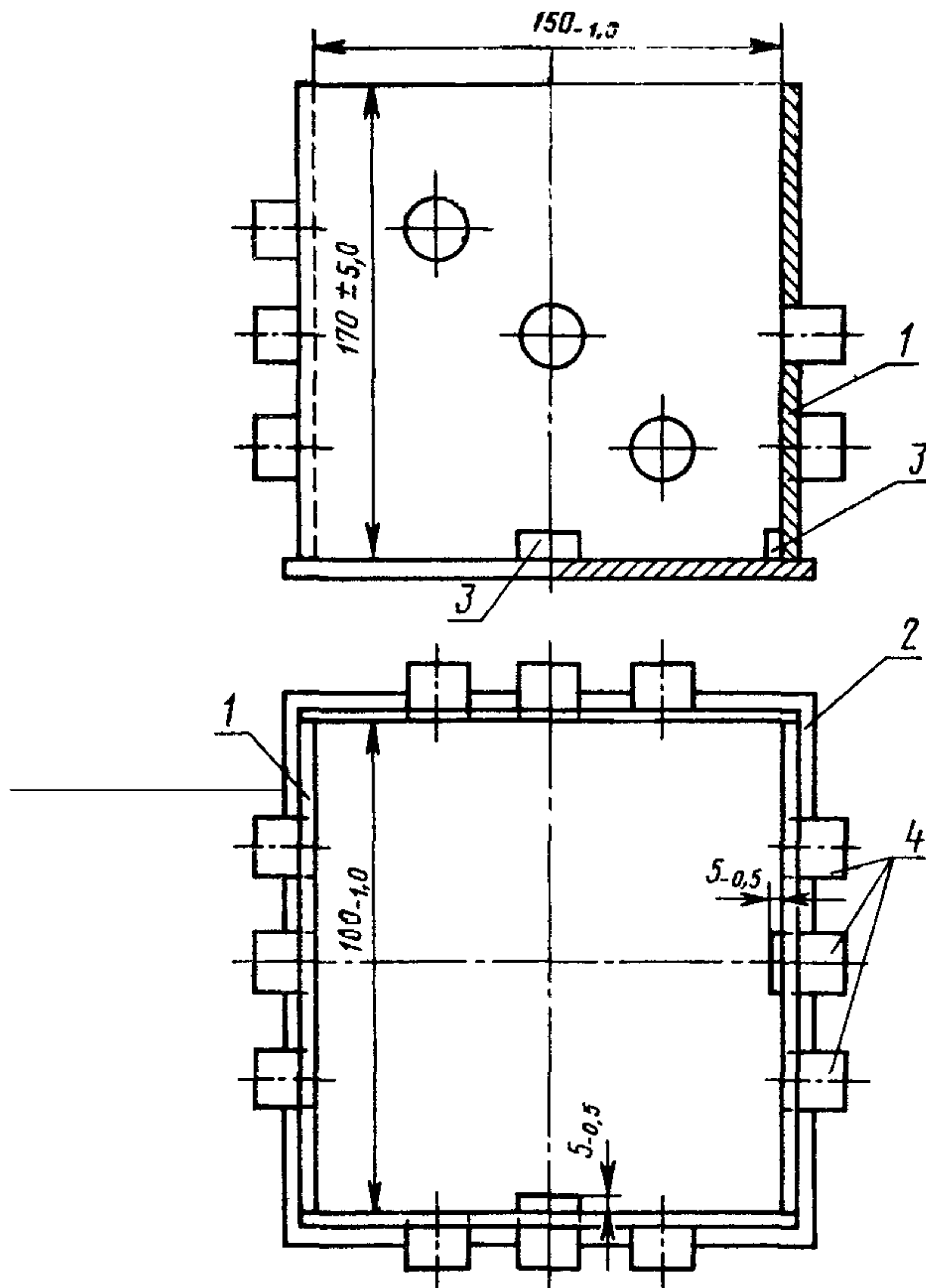
Схема испытательной ванны для образцов размерами 150 \times 150 \times 150 мм
