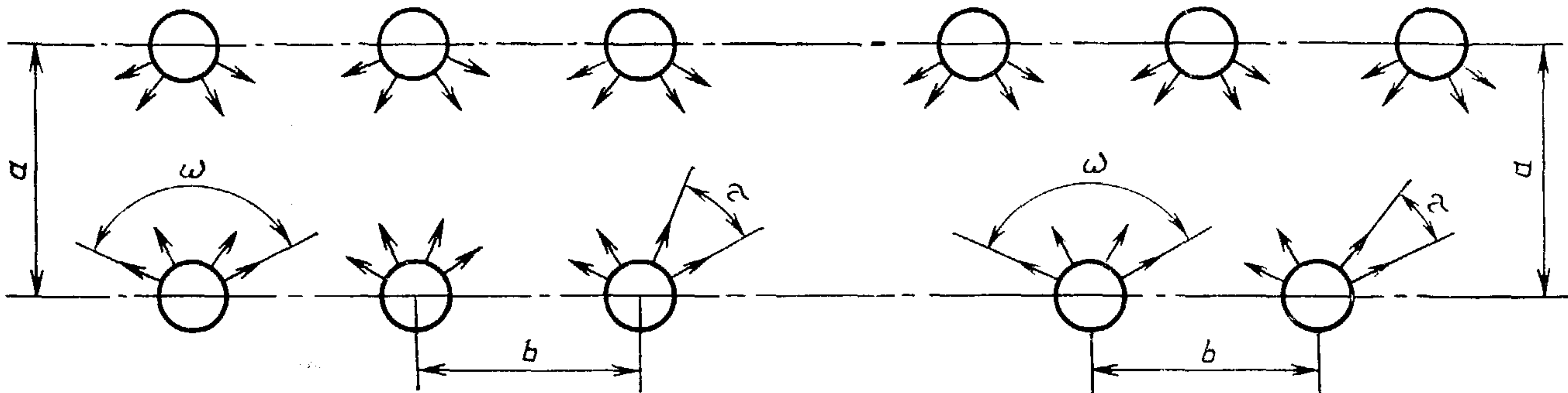
Прямоугольное расположение мачт
