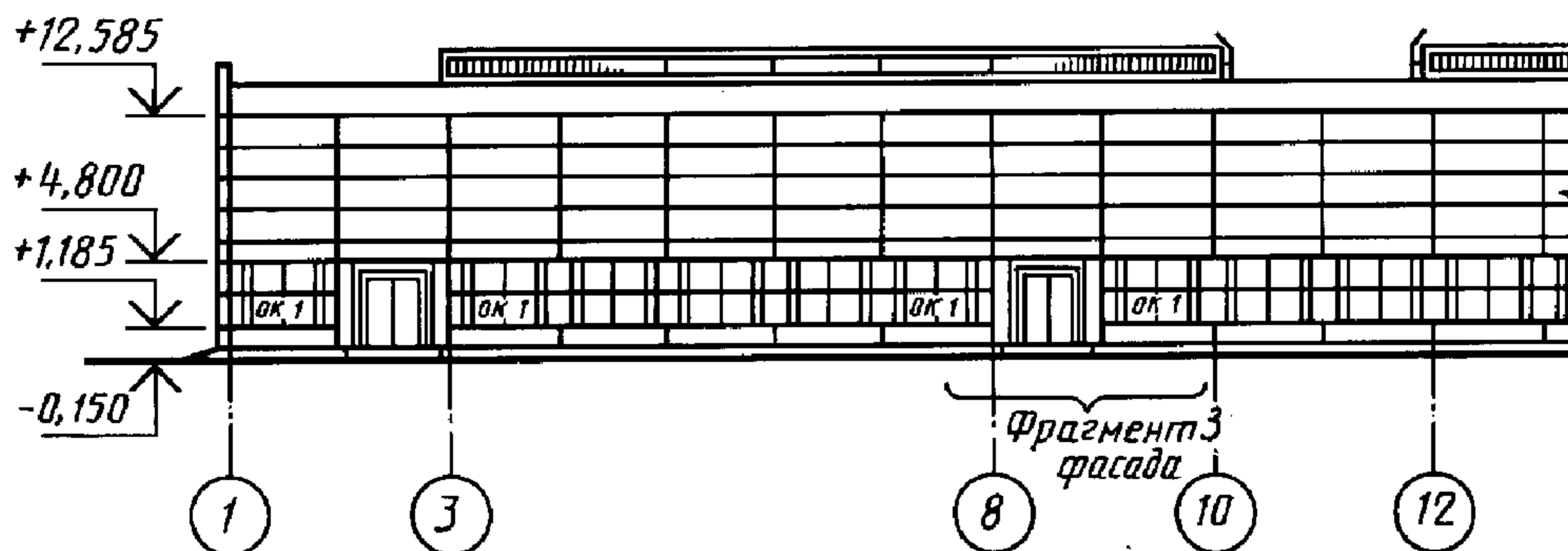
Фрагмент 3 фасада
