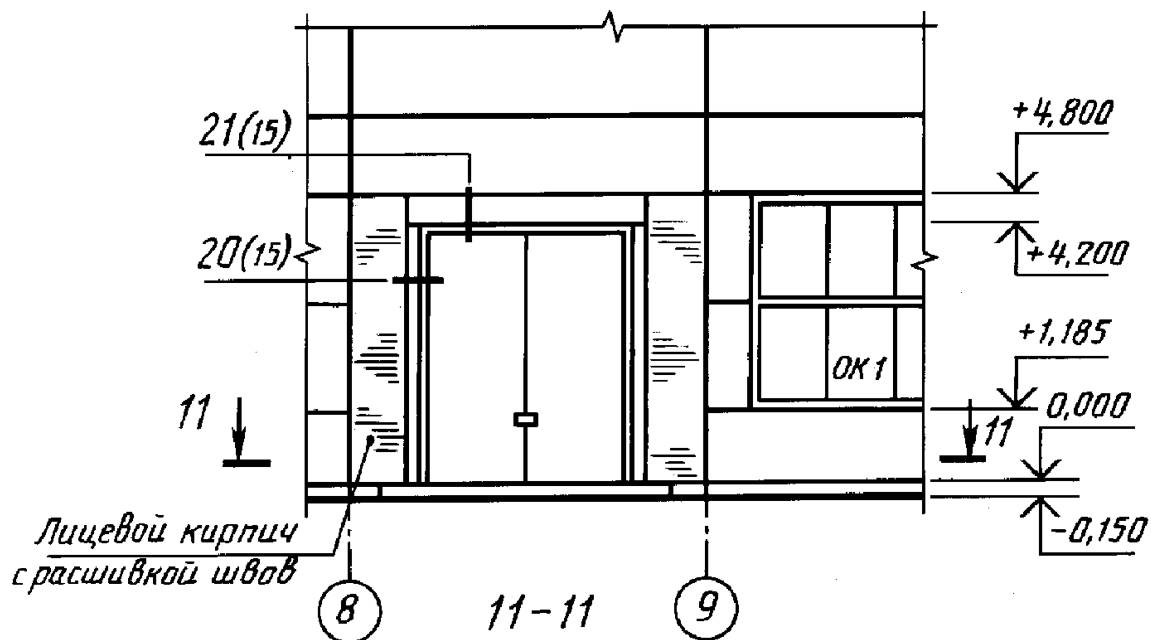
Фрагмент 3 фасада
