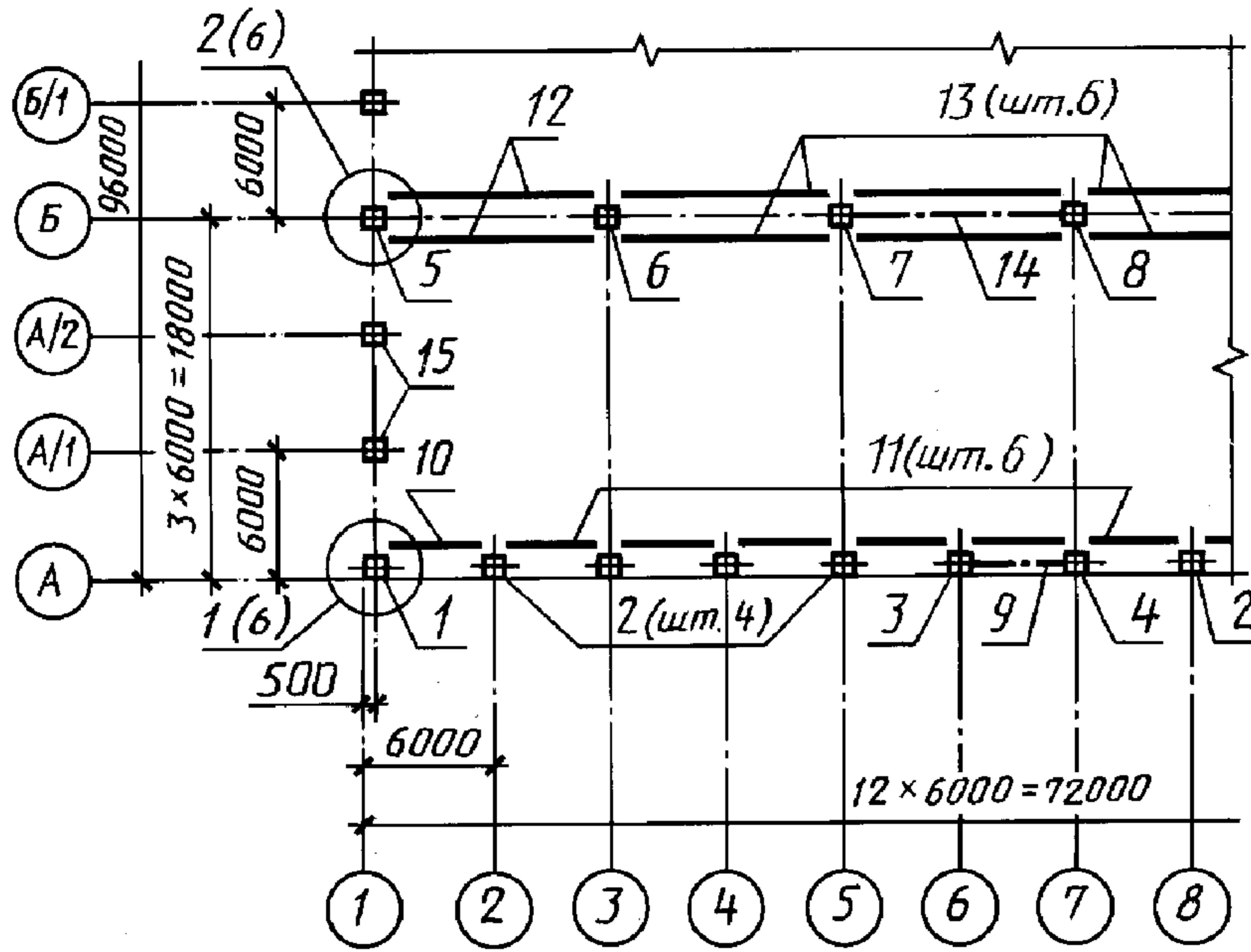
Схема расположения колонн и подкрановых балок
