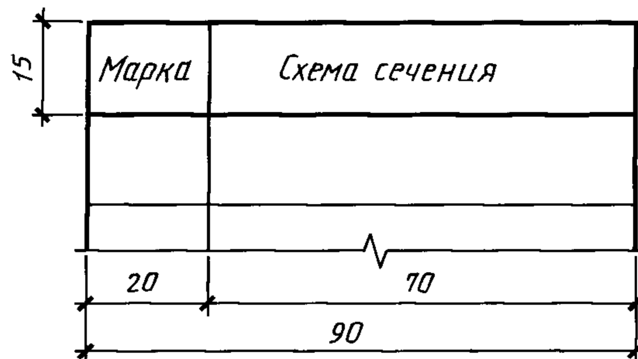
Ведомость перемычек
