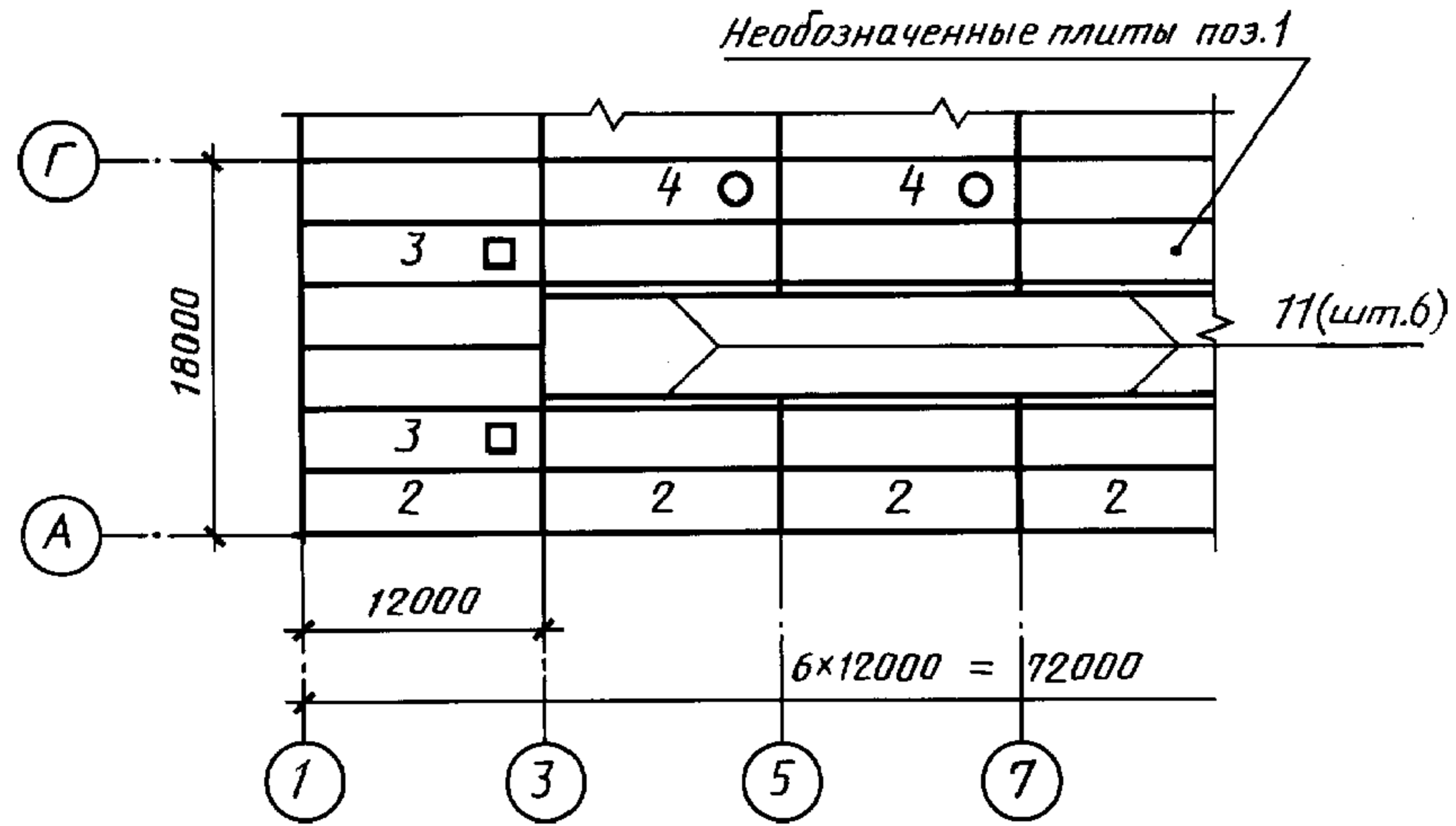
Схема расположения плит покрытия
