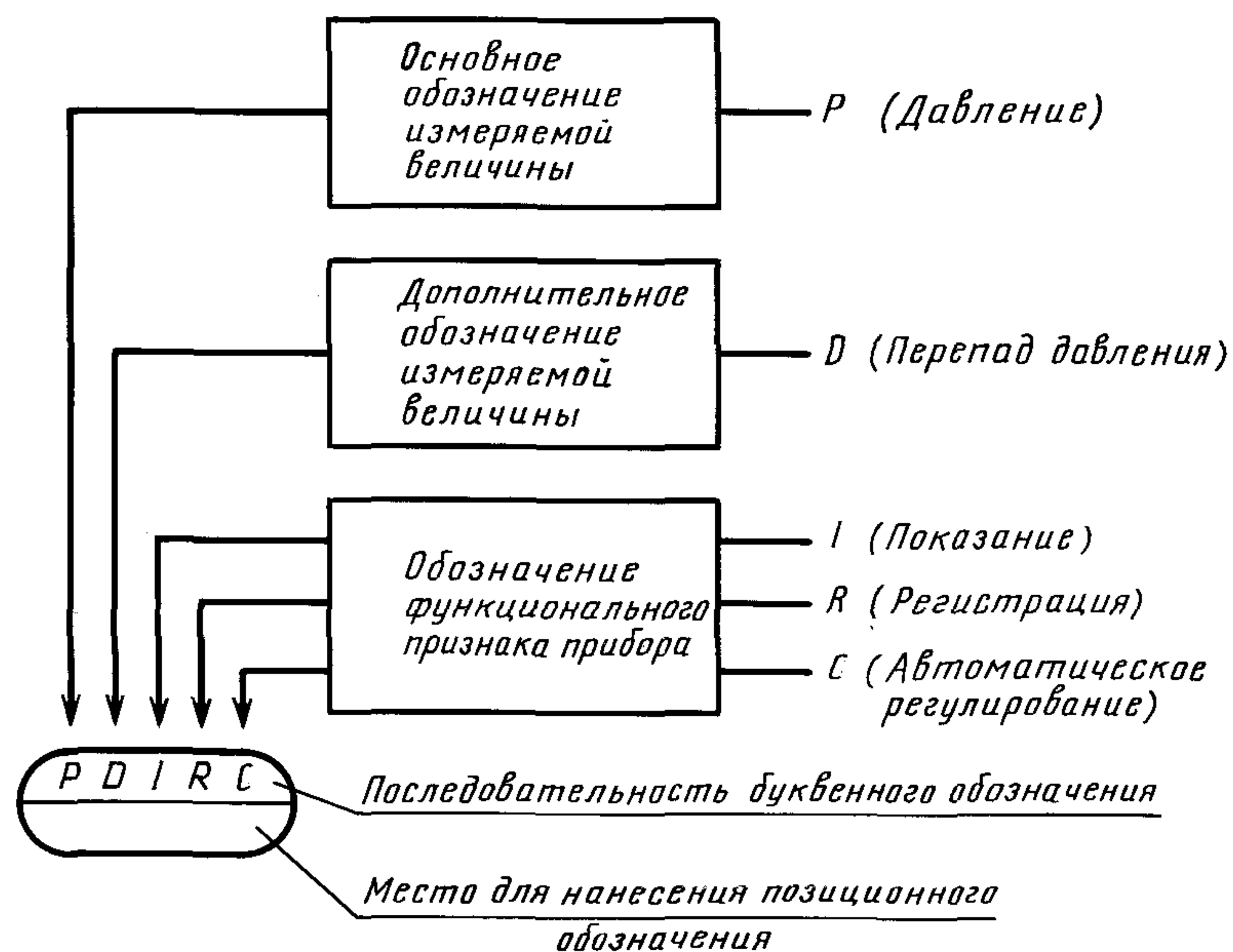
Принцип построения условного обозначения прибора
