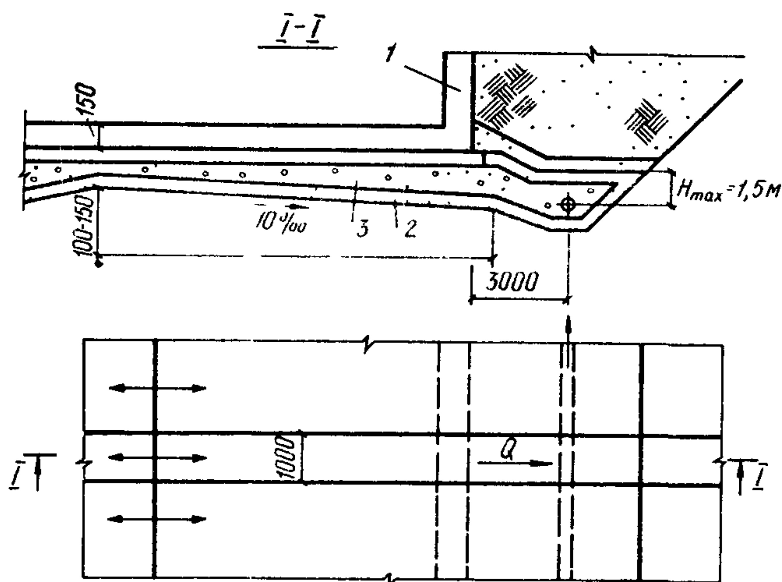
Черт. 16. Расчетная схема пластового дренажа
