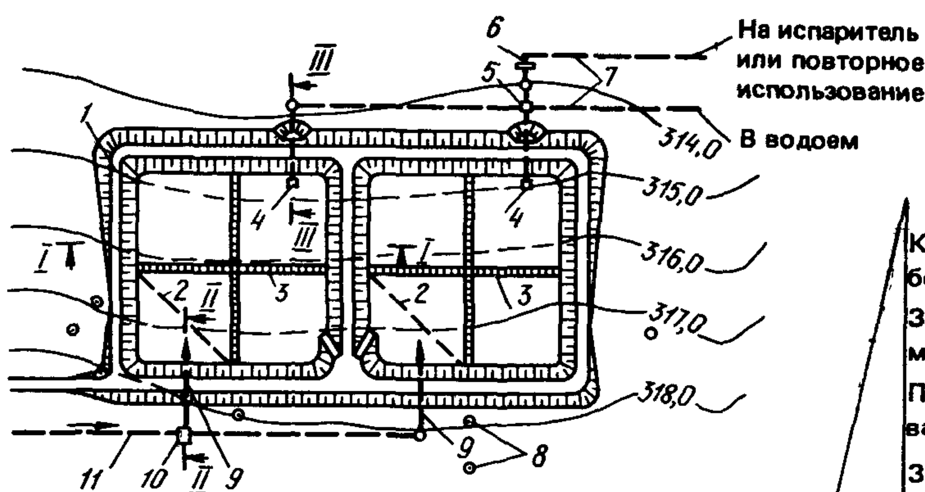
План контрольно-регулирующих прудов дождевых вод
