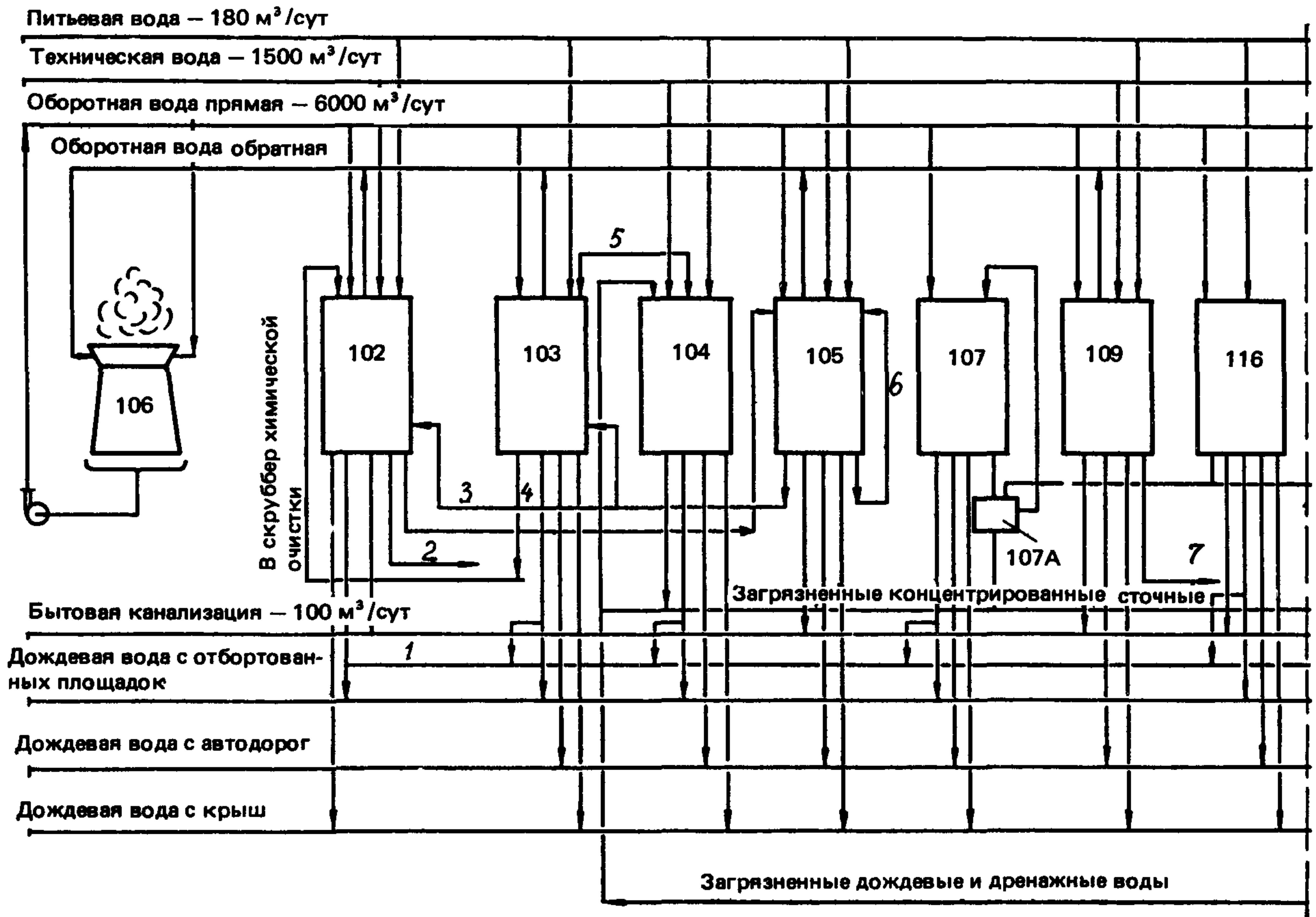
Черт. 30. Схема водопотребления, водоотведения и повторного использования сточных вод полигона по обезвреживанию 1 – первые порции дождевых вод с отбортованных площадок; 2 – соль на захоронение; 3 – известковое молоко; 4 – продув 8 – биологические очистные сооружения с доочисткой; 9 – контрольно-регулирующие пруды; 10 – загрязненные дождевые рующая емкость загрязненных дождевых и дренажных вод; 15 – станция перекачки; 101 – административный корпус; 102 – ходов и реагентов; 105 – приготовление известкового молока и склад хлористого кальция вместимостью 2×1000 м³; 106 – спецмашин и контейнеров и очистные сооружения; 108 – лабораторно-бытовой корпус и щитовая КИП; 109 – котельная с депо на 4 выезда; 113 – магазин; 114 – столовая на 155 посадочных мест; 115 – блок ремонтных мастерских; 115а – лесо ем на 50 автомашин и автобусов хозяйственного назначения; 119 – подстанция 35/10 кВ с распределительным устройством сооружения
