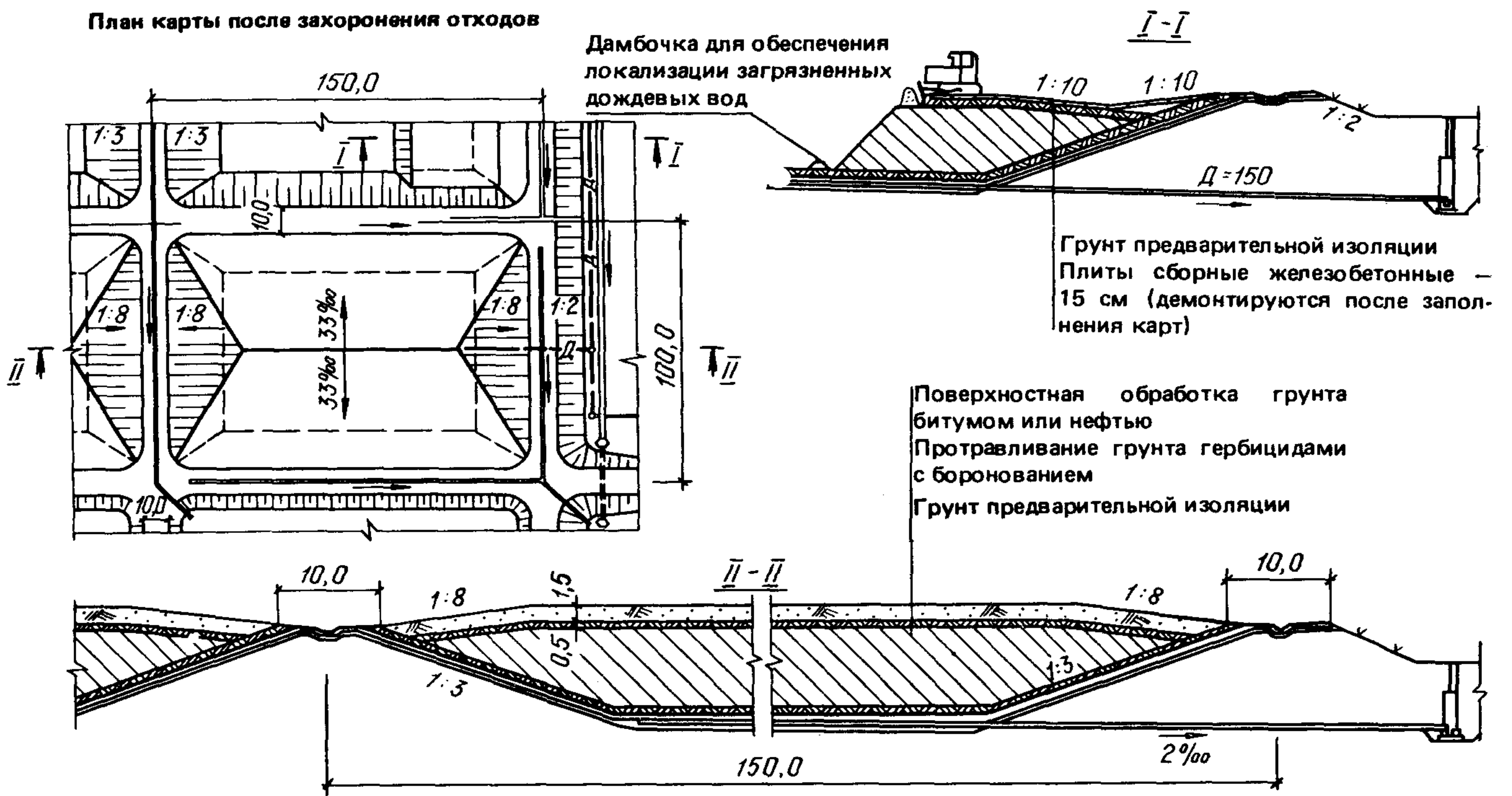
Черт. 25. Карты для захоронения отходов
