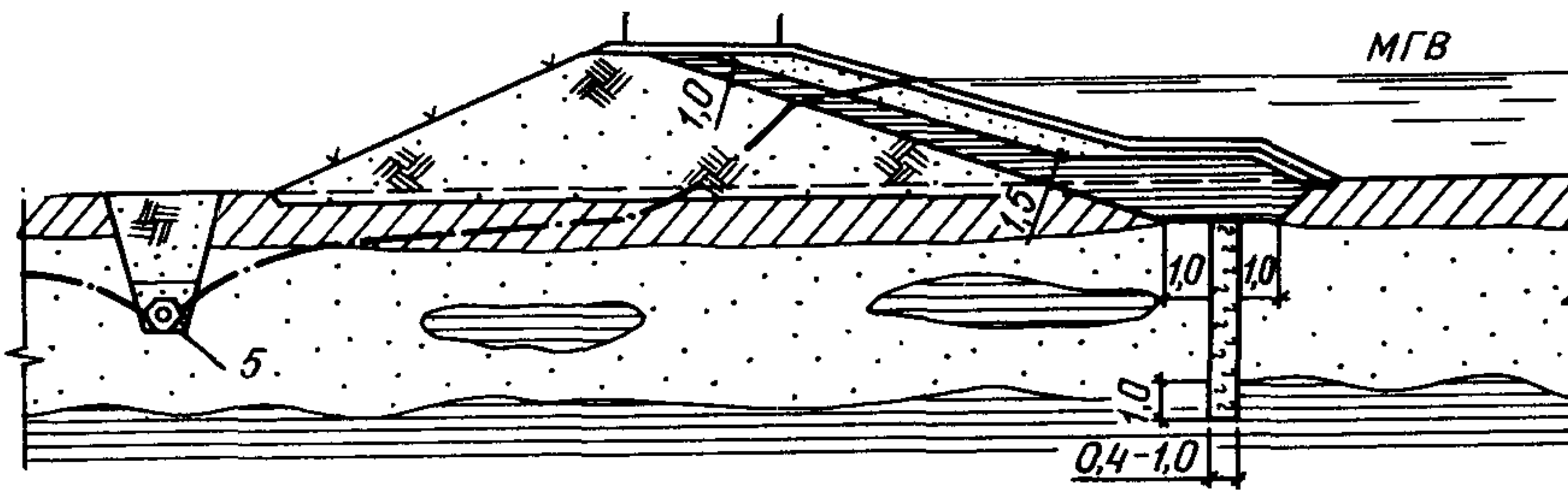
I-I (Вариант 2)
