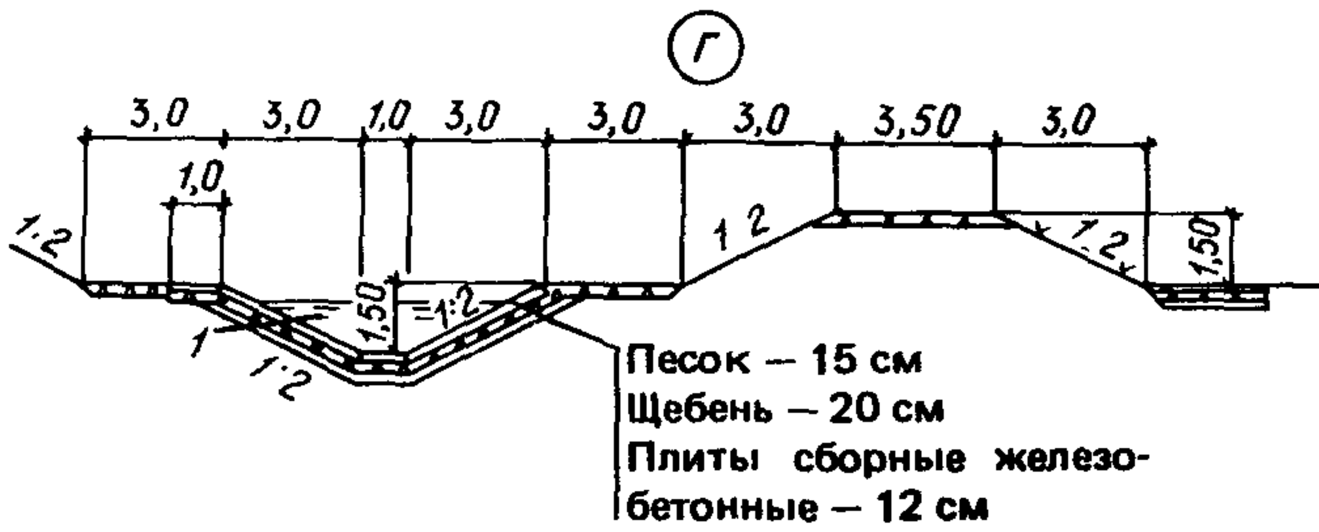
Черт. 23. Участок захоронения не утилизируемых промышленных отходов. Узлы В, Г, Д, Ж
