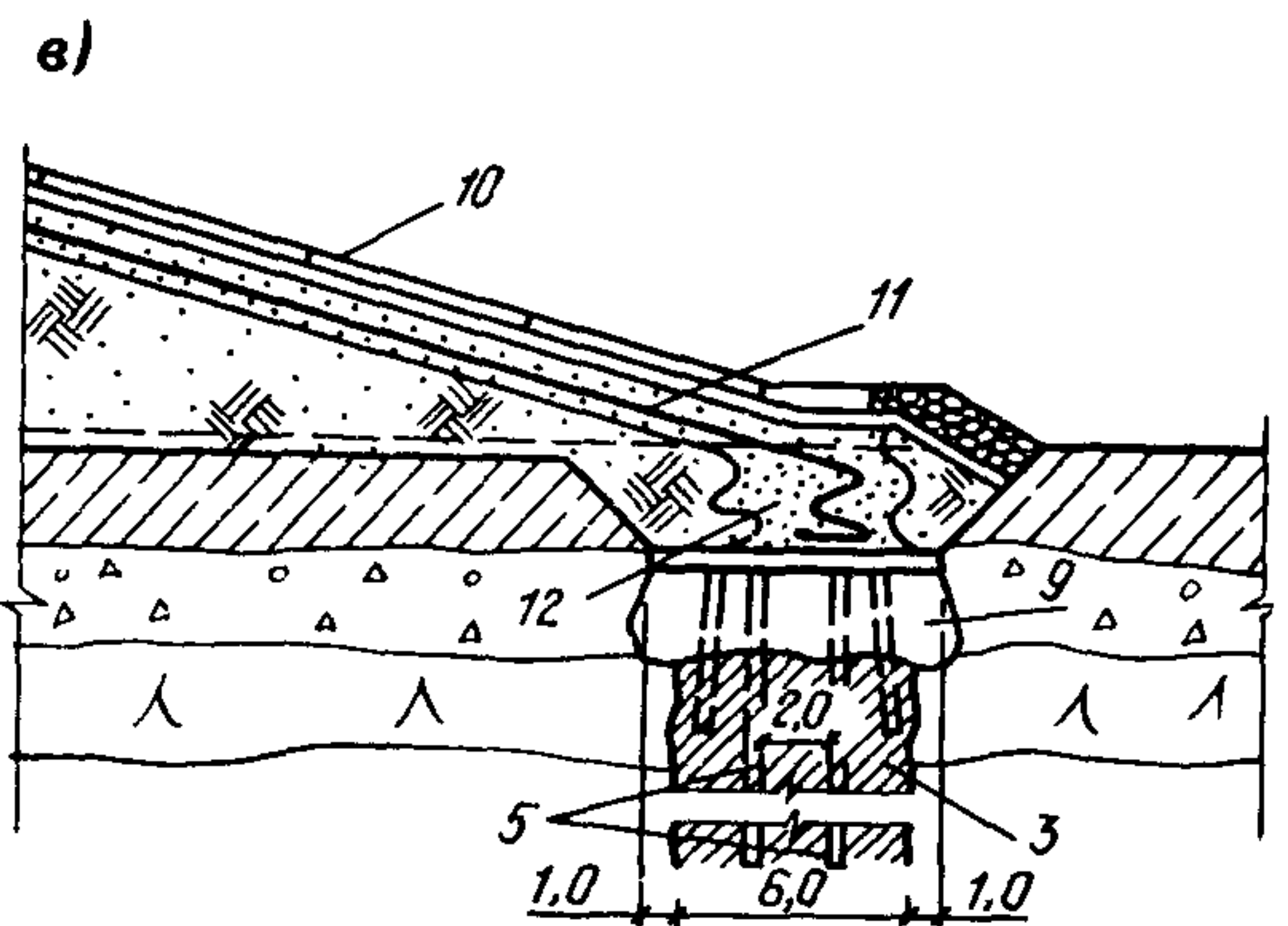
Черт. 14. Цементационная завеса. Узлы сопряжений
