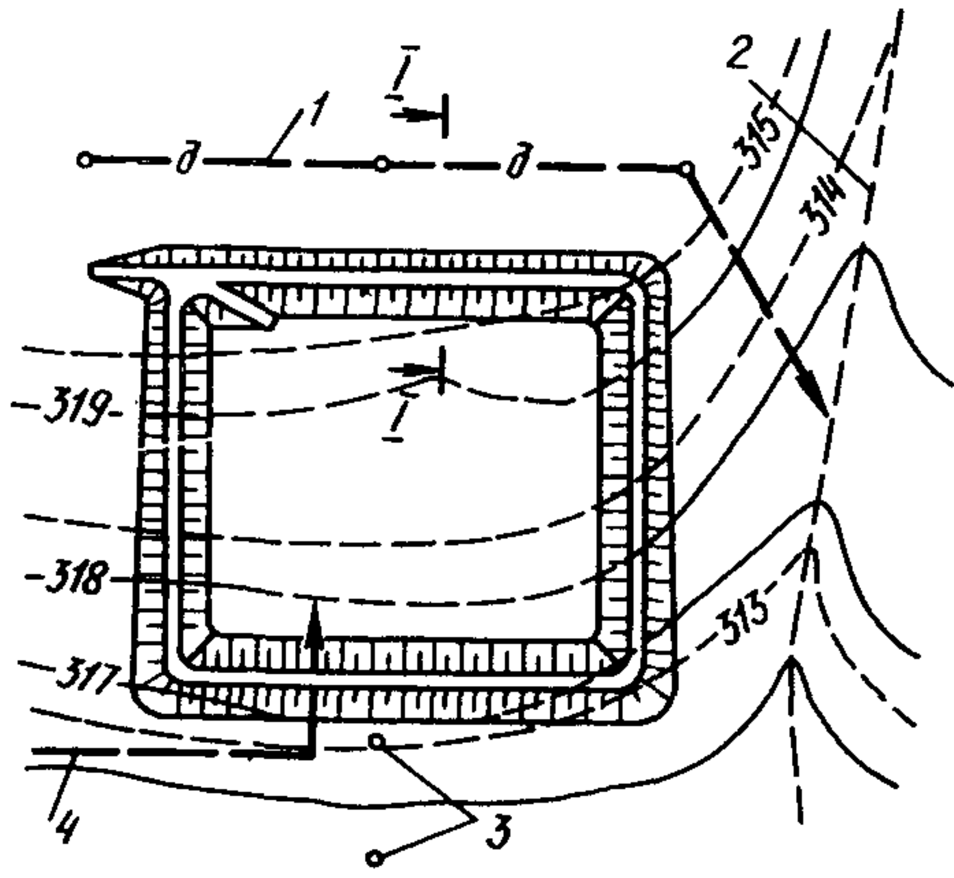
План пруда-испарителя
