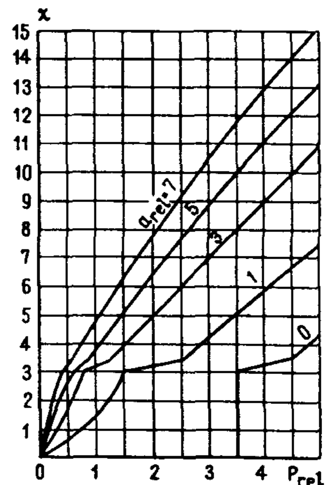
Черт. 3. График зависимости коэффициента \chi от p_{rel} при a_{rel} = const
