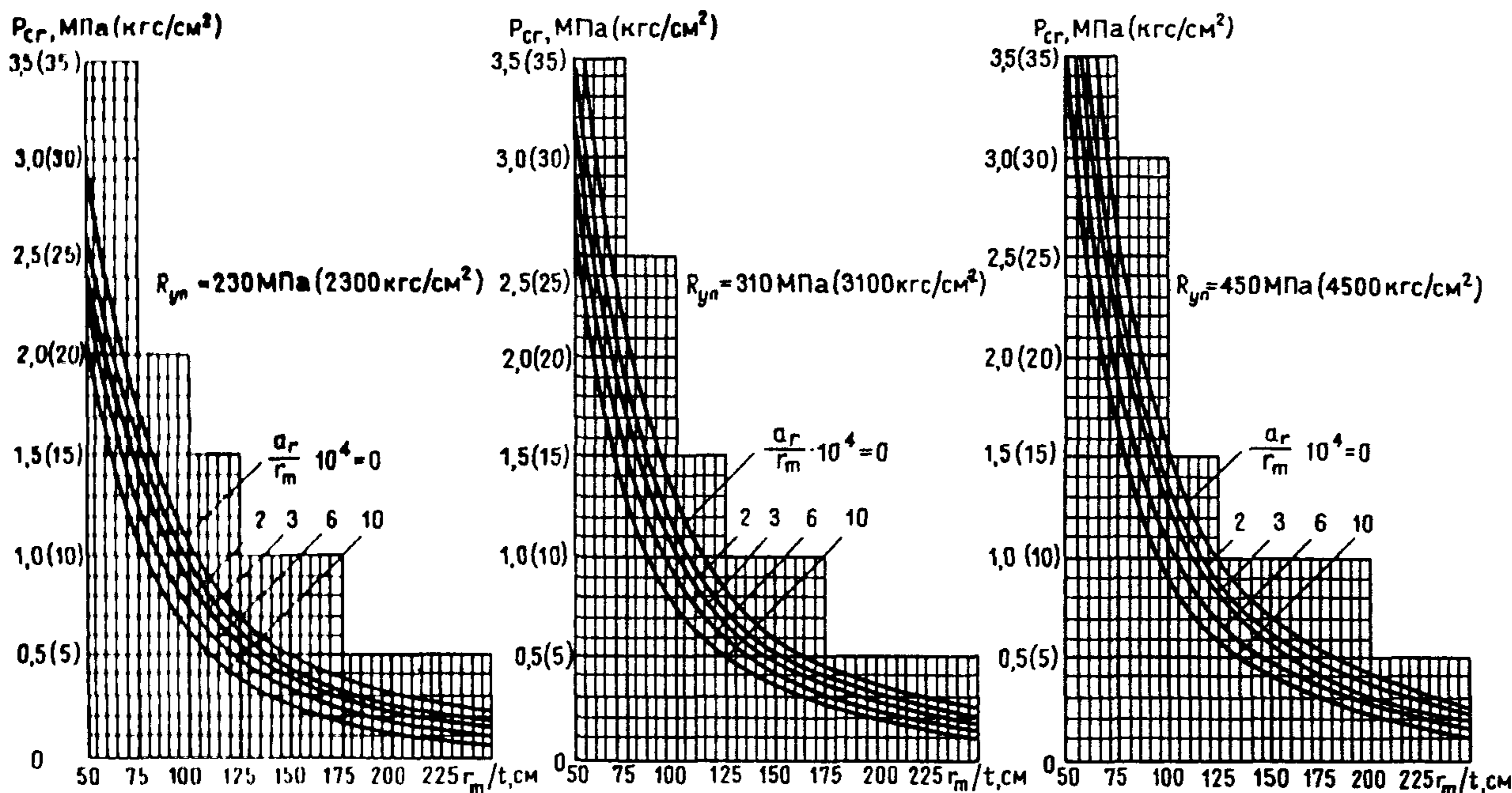
Черт. 2. Графики зависимости критического наружного давления p_{cr} от относительной толщины стенки r_m/t [ R_{yn} — нормативное сопротивление по пределу текучести стали, МПа (кгс/см 2 ); a_r — расчетный радиальный зазор между стенкой оболочки и бетоном, см; r_m — средний радиус оболочки, см; t — толщина стенки оболочки, см]
