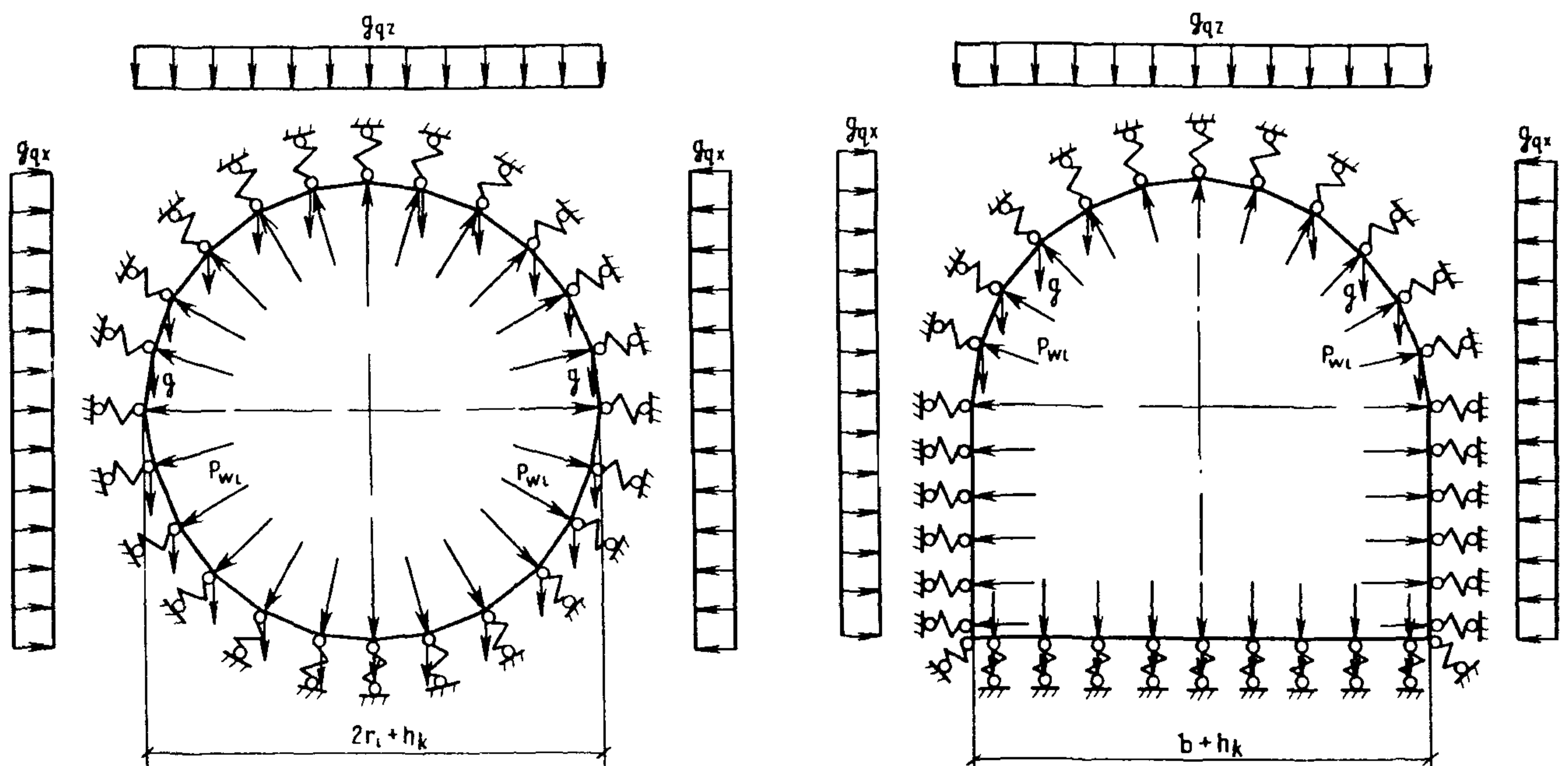
Черт. 1. Расчетные схемы обделок туннелей
