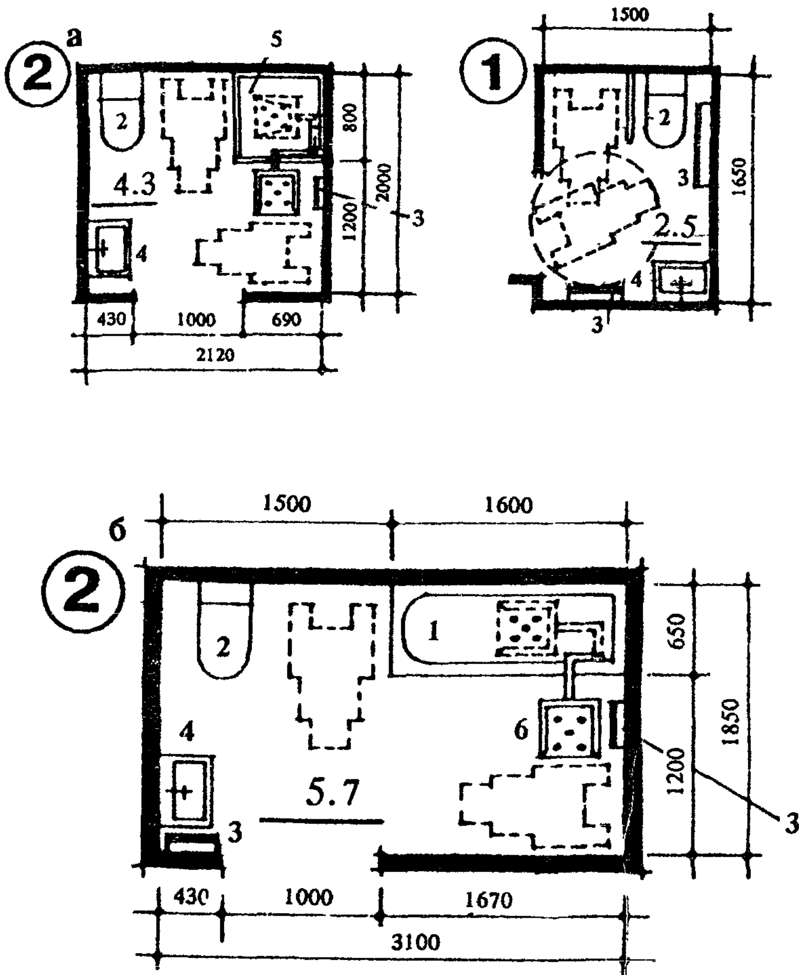
Рис. 8. Планировочные схемы санитарных узлов. Вариант 1 — Уборная с умывальником. Вариант 2 — Санитарный узел при спальняй комнате (а — вариант с душем, б — вариант с ванной). Эхспликация оборудования: 1. ванна 65x160, 2. унитаз 40x60, 3. вешалка для полотенец, 4. умывальник 60x40, 5. душевой поддон 80x80, 6. поворотное кресло.
