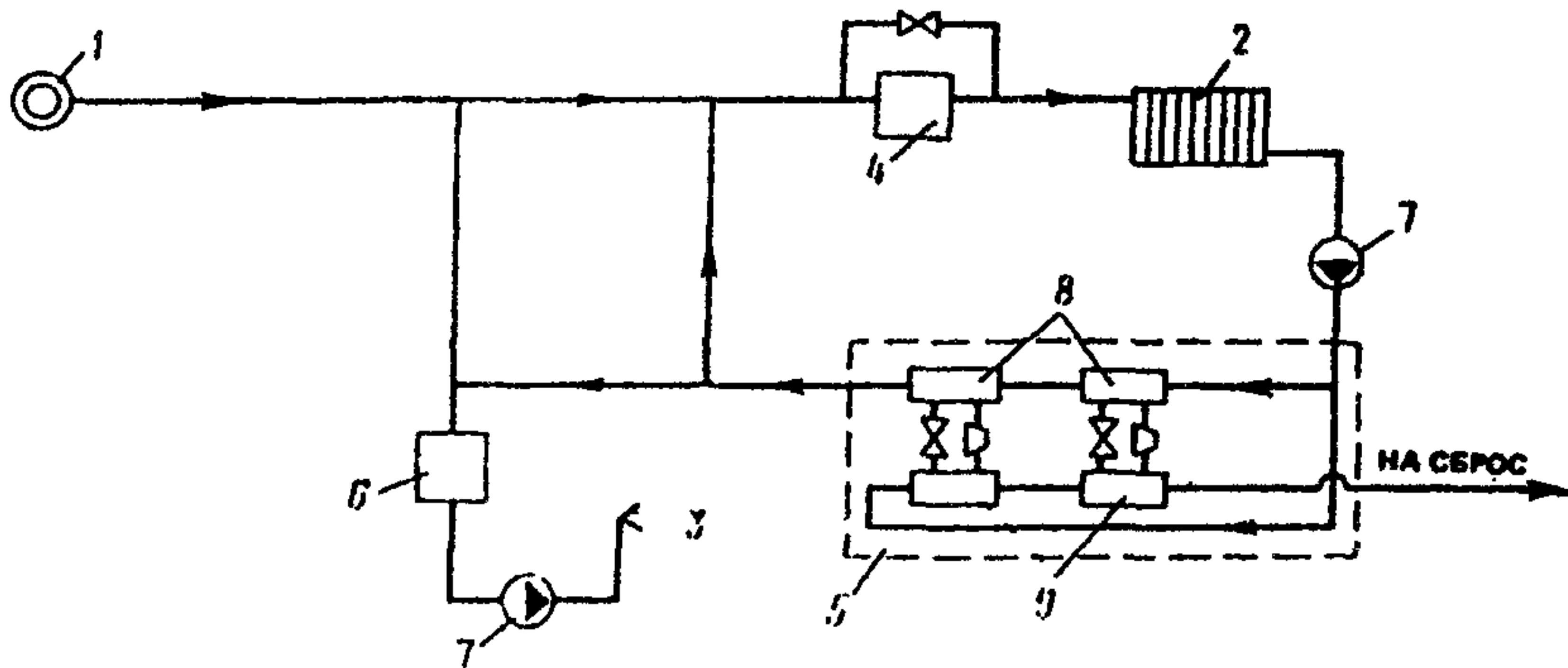
Рис. 11. Принципиальная схема системы геотермального теплоснабжения с применением пикового догрева и тепловых насосов
