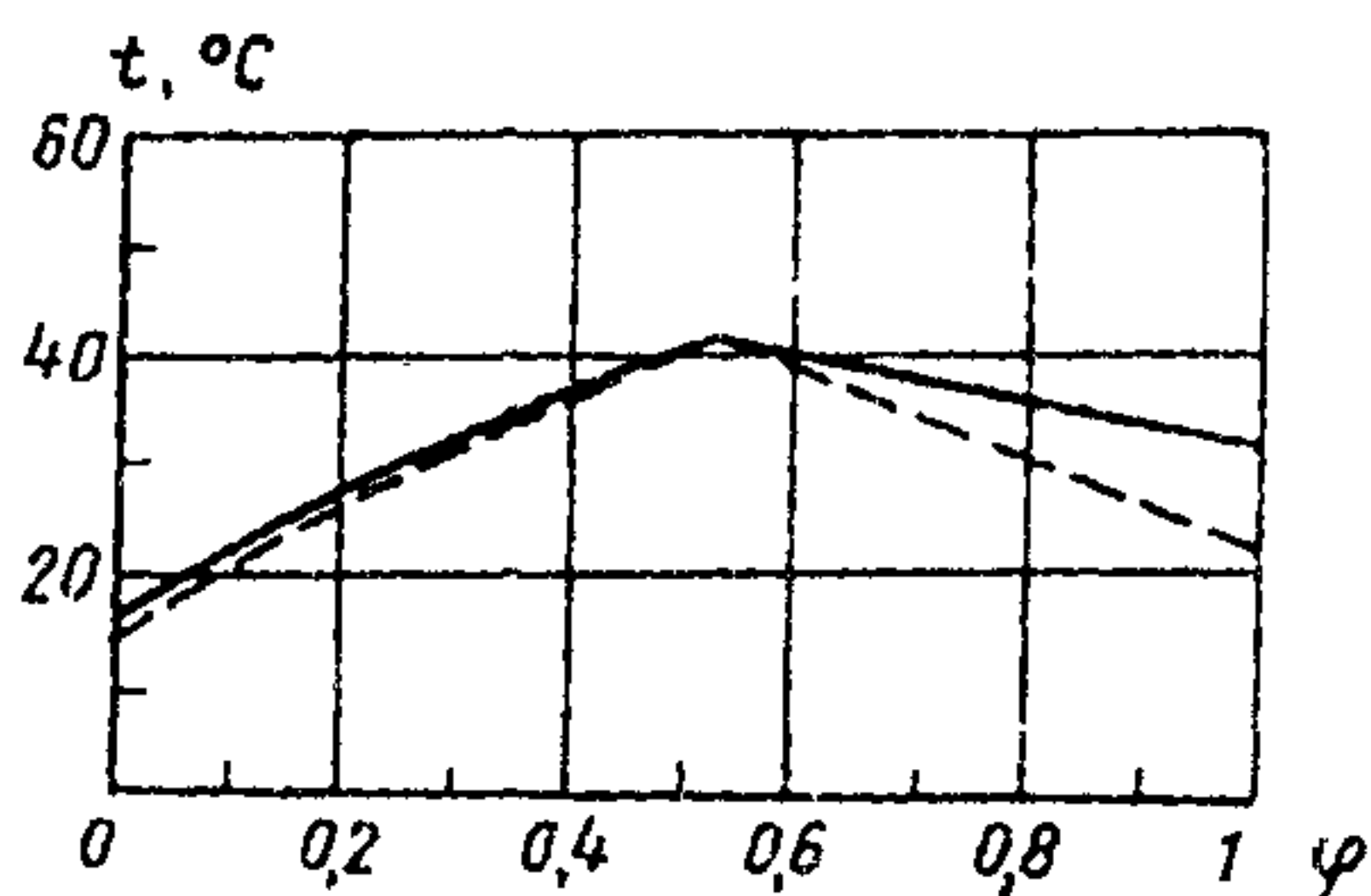
Рис. 3. Температура сбросной геотермальной воды — — — — комплексная система с пиковой котельной; - - - - - то же, с НТУ
