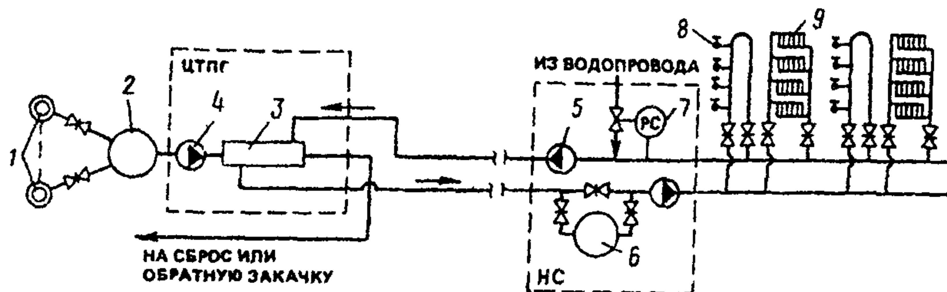
Рис. 8. Закрытая двухтрубная геотермальная система теплоснабжения 1 — геотермальные скважины термоводозабора; 2 — сборный бак-аккумулятор геотермальной воды; 3 — сетевой теплообменник; 4 — сетевой насос геотермальной воды; 5 — сетевой насос водопроводной воды; 6 — бак-аккумулятор водопроводной воды; 7 — регулятор подпитки; 8 — водоразборный кран ГВ; 9 — отопительный прибор
