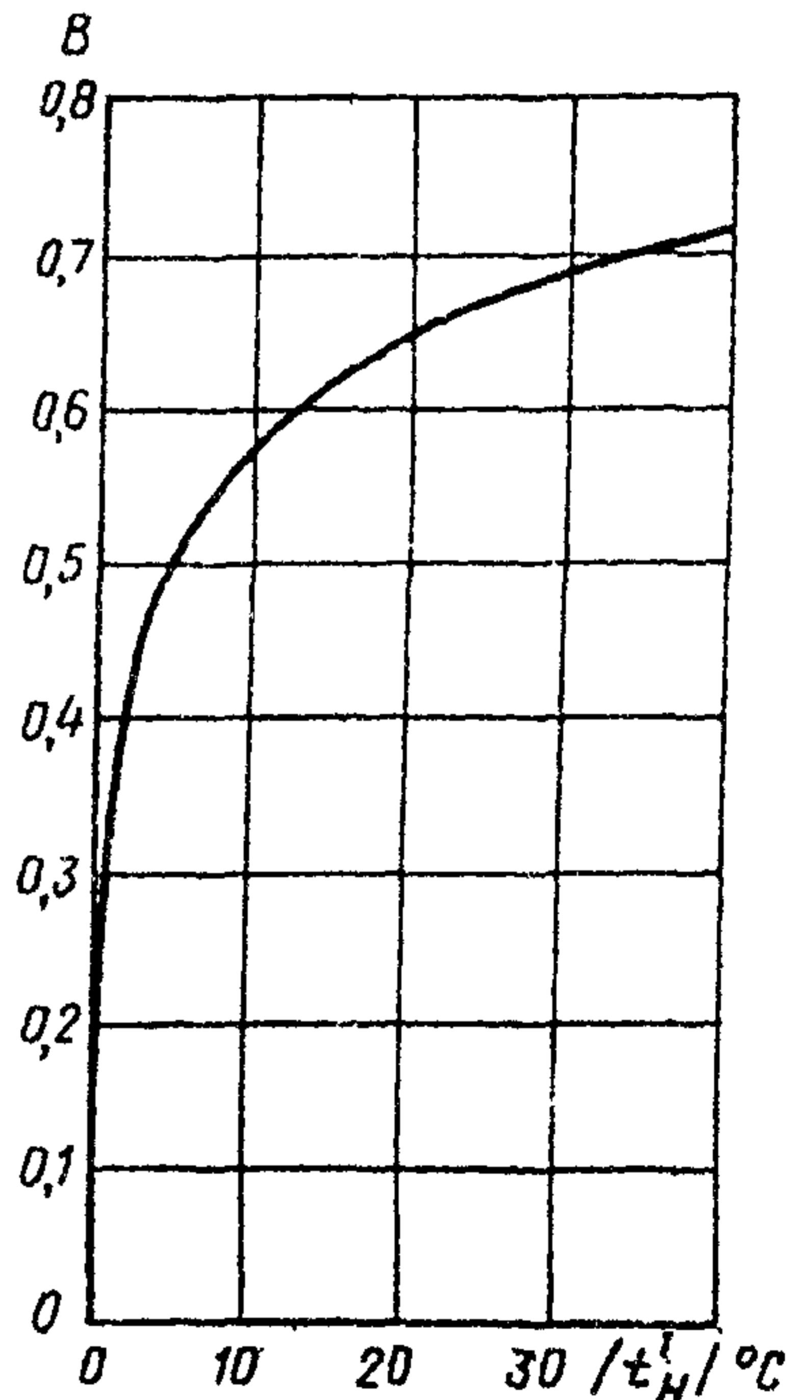
Рис. 4. Эмпирический коэффициент B для определения доли пикового догрева
