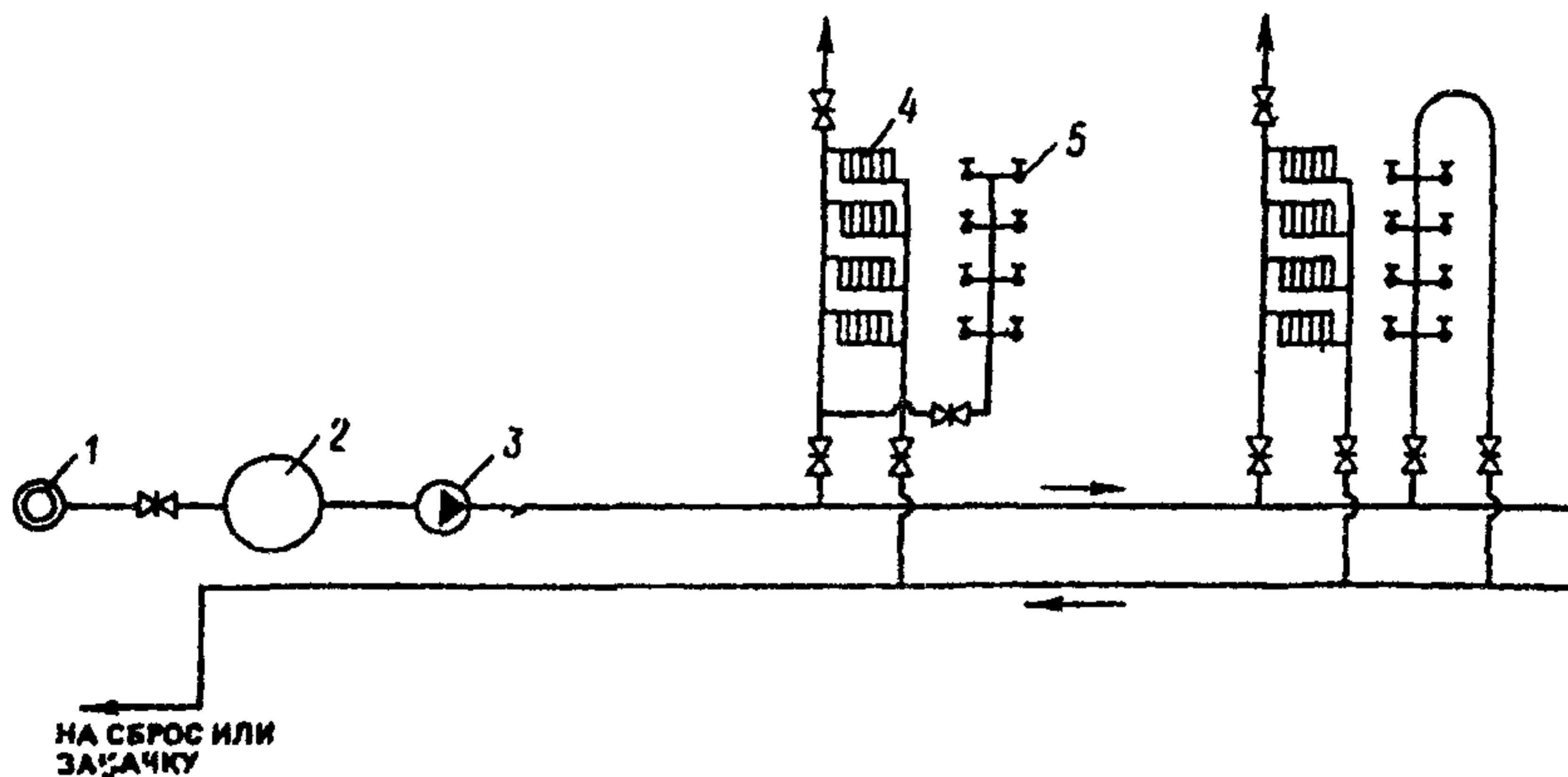
Рис. 3. Открытая двухтрубная геотермальная система теплоснабжения 1 — геотермальная скважина; 2 — бак-аккумулятор; 3 — сетевой насос; 4 — отопительные приборы; 5 — водоразборный кран
