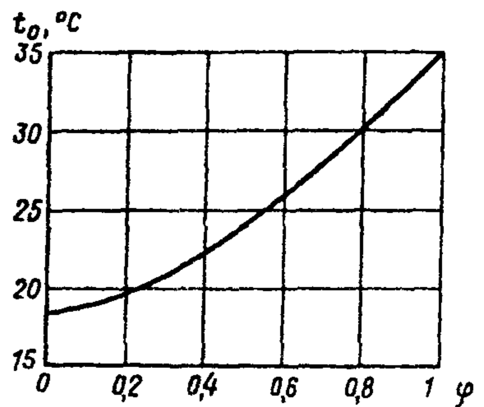
Рис. 2. График температуры обратной воды при количественном регулировании отопительной нагрузки ( t''_T = 80 \text{ }^\circ\text{C} , t''_0 = 35 \text{ }^\circ\text{C} , t_B = 18 \text{ }^\circ\text{C} )
