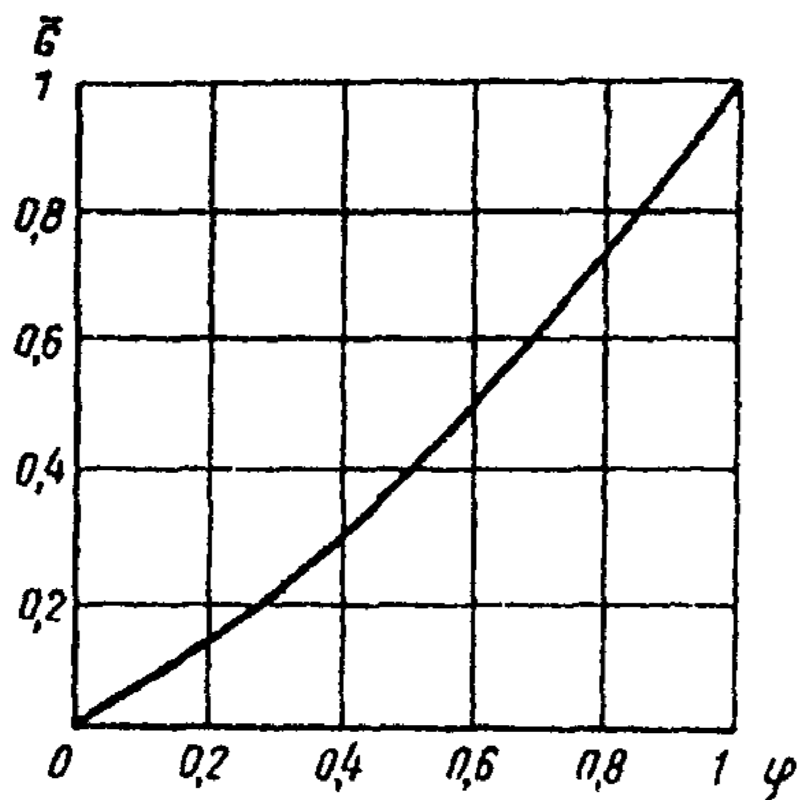
Рис. 1. График расхода теплоносителя при количественном регулировании отопительной нагрузки ( t''_T = 80 \text{ }^\circ\text{C} , t''_0 = 35 \text{ }^\circ\text{C} , t_B = 18 \text{ }^\circ\text{C} )
