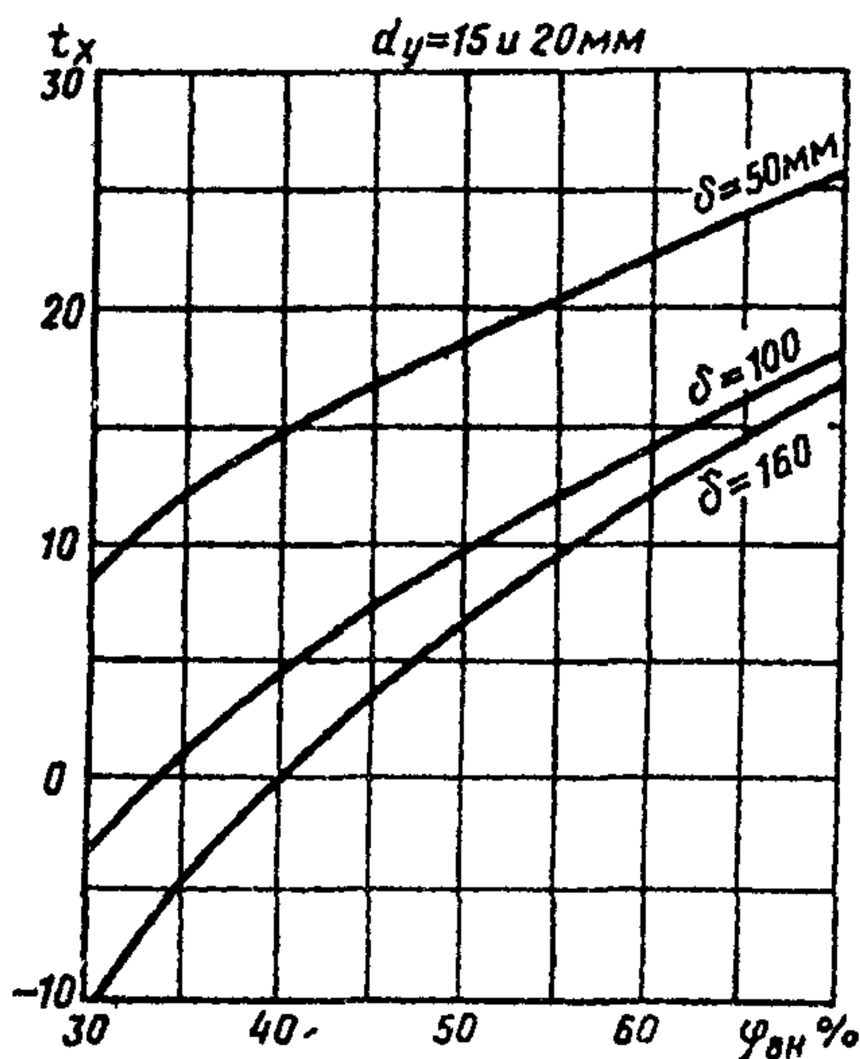
Рис. 5. Зависимость температуры хладоносителя от относительной влажности внутреннего воздуха \varphi_{вн} d_y — условный диаметр труб, мм; \delta — толщина слоя тяжелого бетона, по нейтральной оси которого замонтированы трубы, мм.
