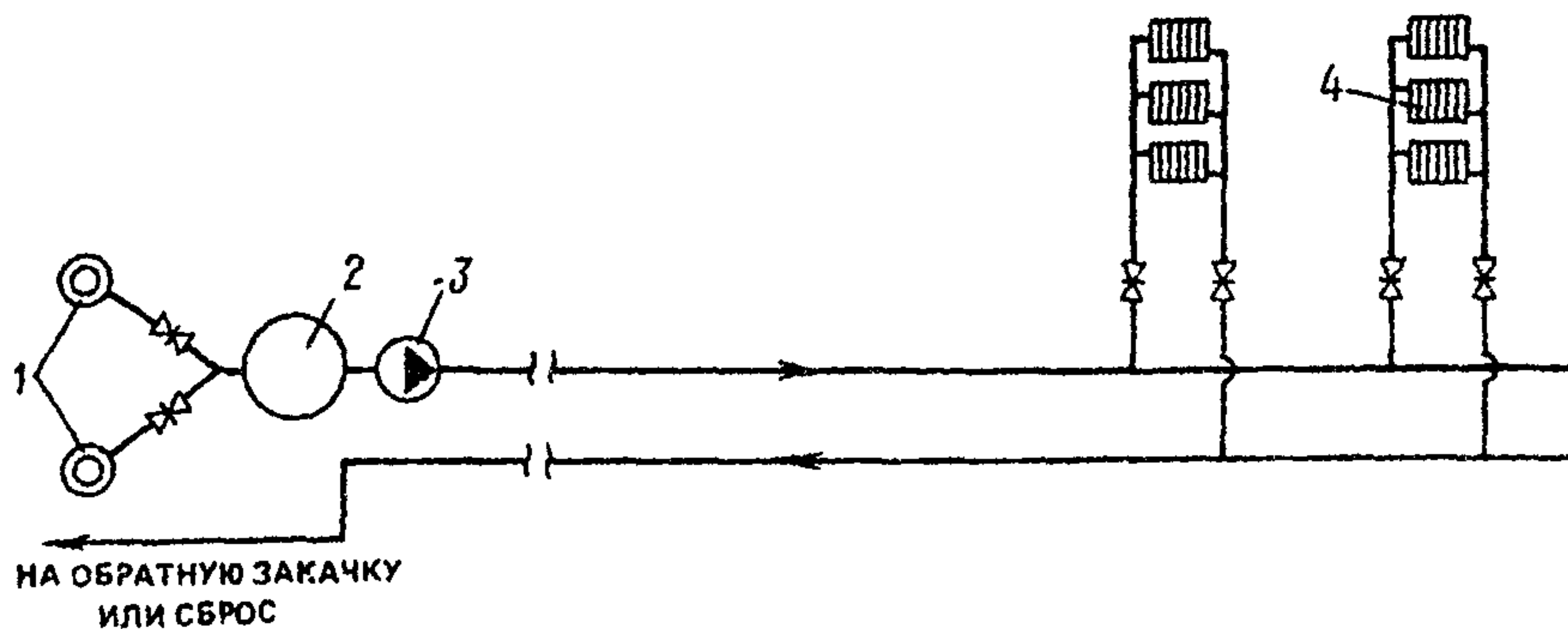
Рис. 9. Геотермальная система теплоснабжения с зависимым присоединением отопления (ГВ отсутствует) 1 — геотермальные скважины; 2 — промежуточный бак-аккумулятор геотермальной воды; 3 — сетевой насос; 4 — отопительные приборы
