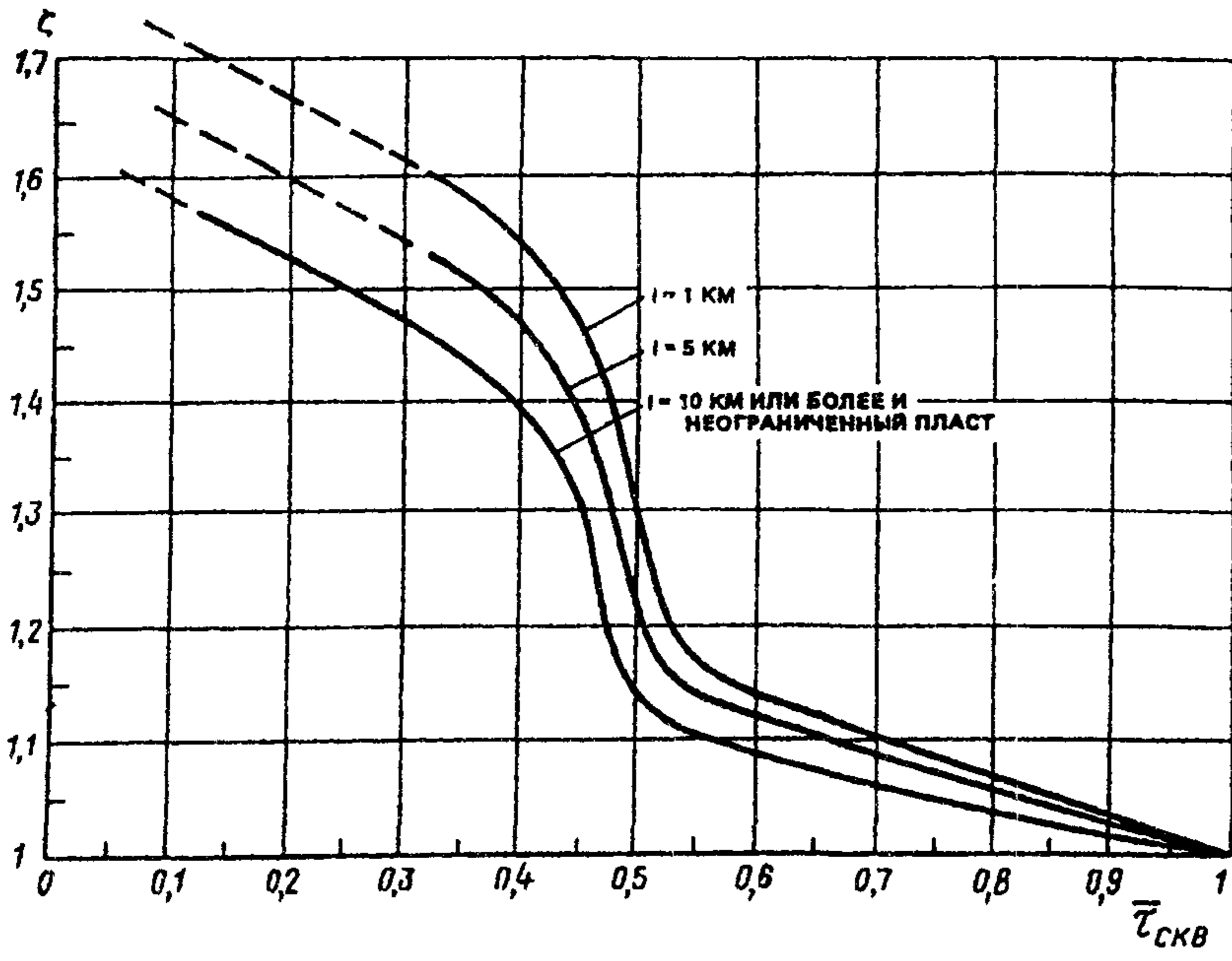
Рис. 1. Графики для определения степени относительного увеличения расчетного дебита термоводозабора
