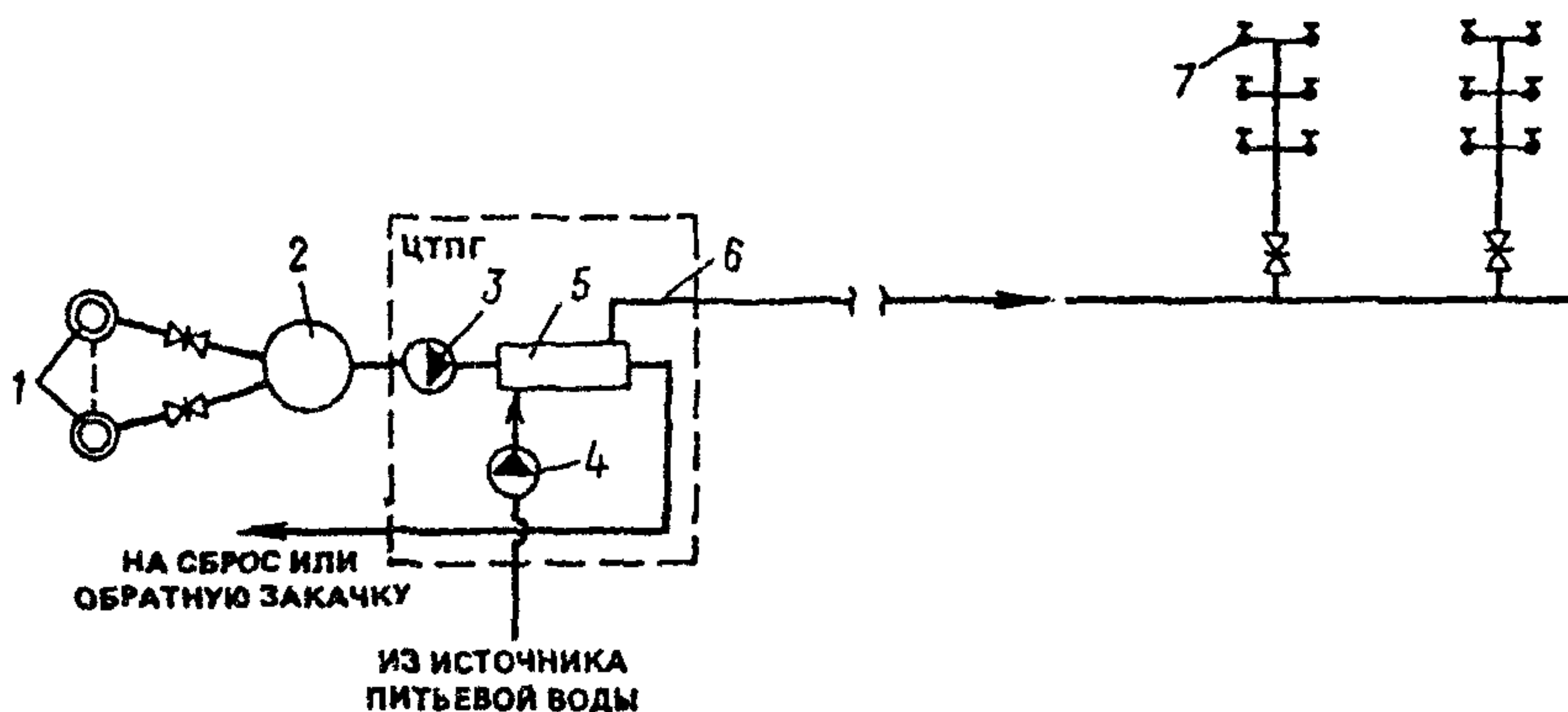
Рис. 4. Однострубно́й закрытая геотермальная система горячего водоснабжения с источником питьевой воды, расположенным на термоводозаборе 1 — геотермальные скважины термоводозабора; 2 — сборный бак-аккумулятор геотермальной воды; 3 — сетевой насос геотермальной воды; 4 — сетевой насос питьевой воды; 5 — сетевой теплообменник; 6 — однострубно́й транзитная теплотрасса; 7 — водоразборный кран
