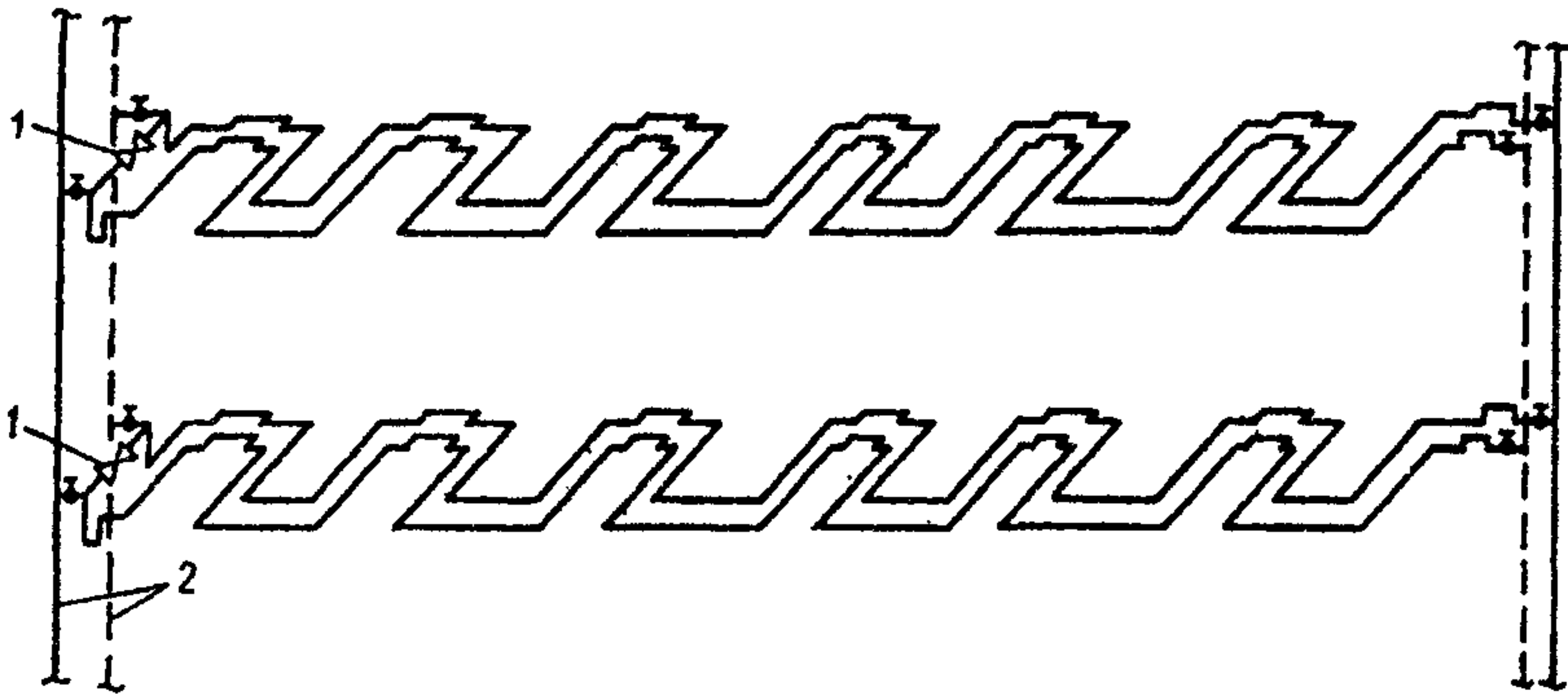
Рис. 8. Система отопления — охлаждения с дополнительными стояками 1 — задвижка на перемычке, открытая зимой и закрытая летом; 2 — дополнительные стояки для режима охлаждения
