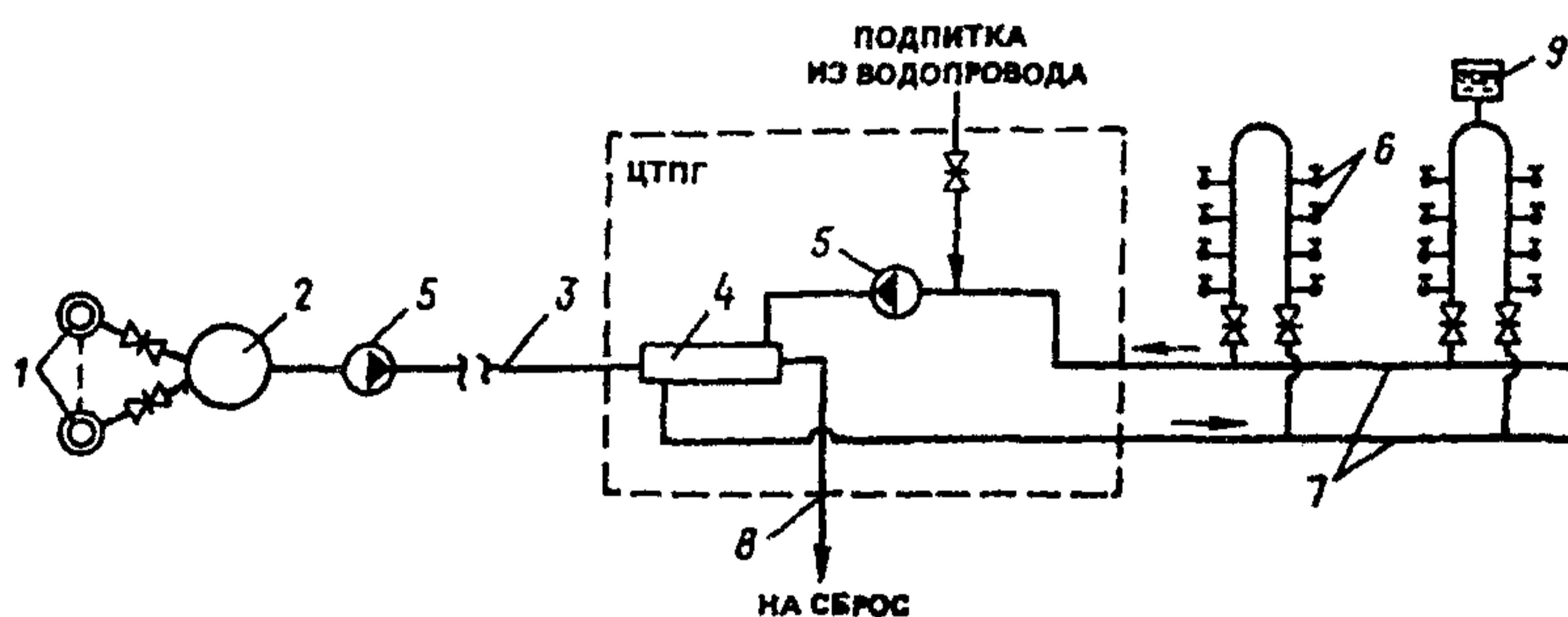
Рис. 5. Однострунная закрытая геотермальная система горячего водоснабжения
