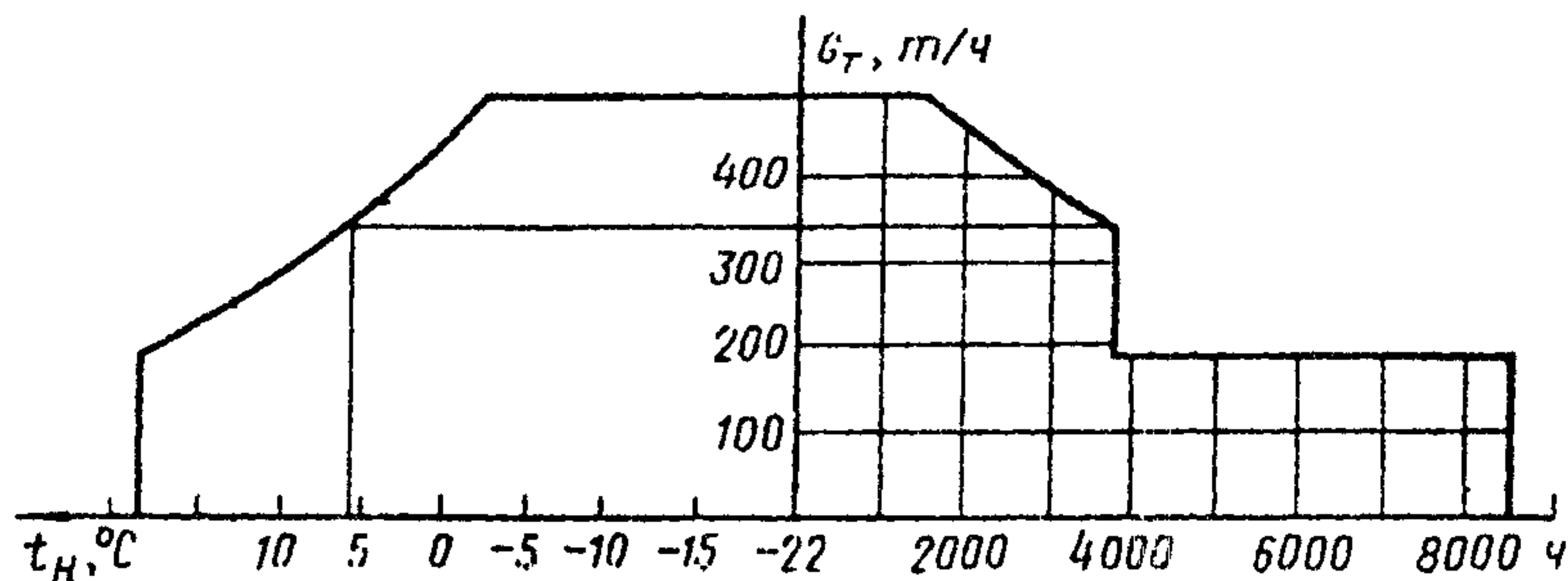
Рис. 2. График продолжительности расхода геотермального теплоносителя
