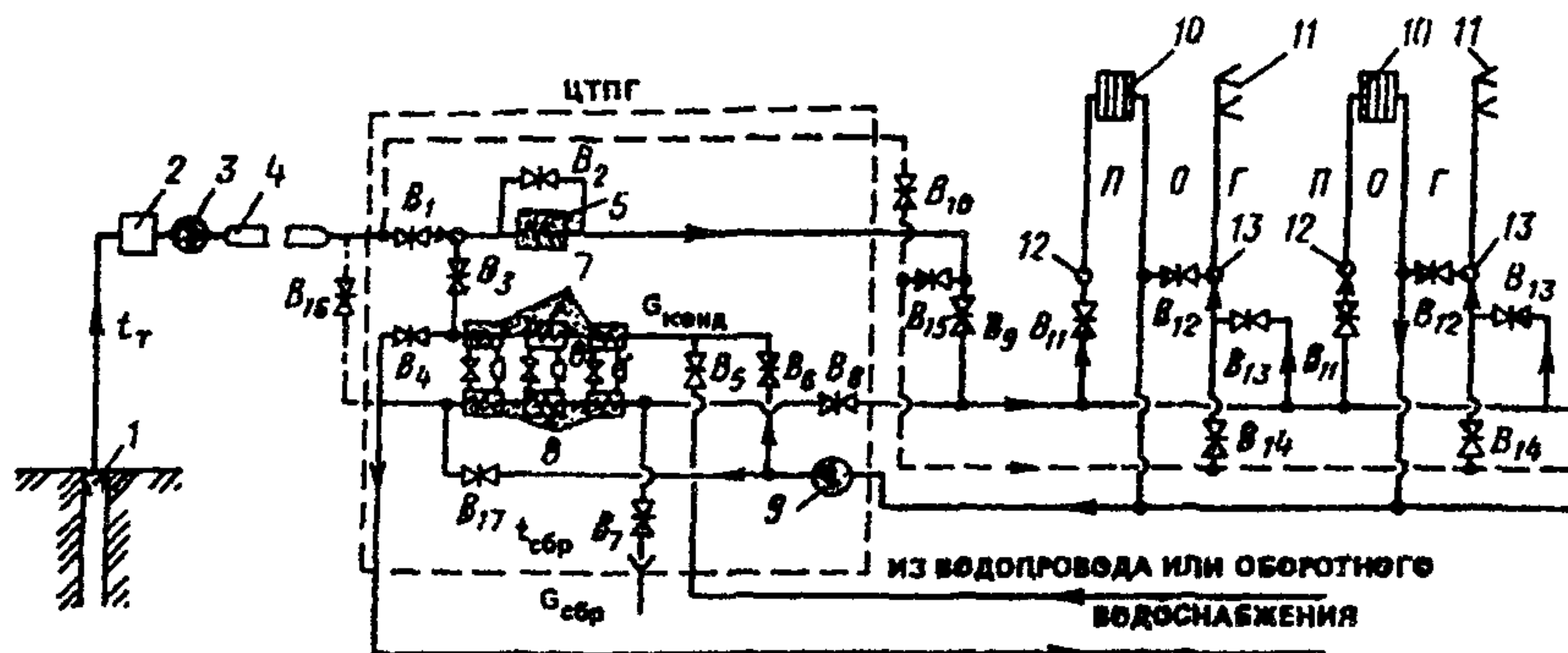
Рис. 12. Система централизованного теплохладоснабжения с тепловыми насосами
