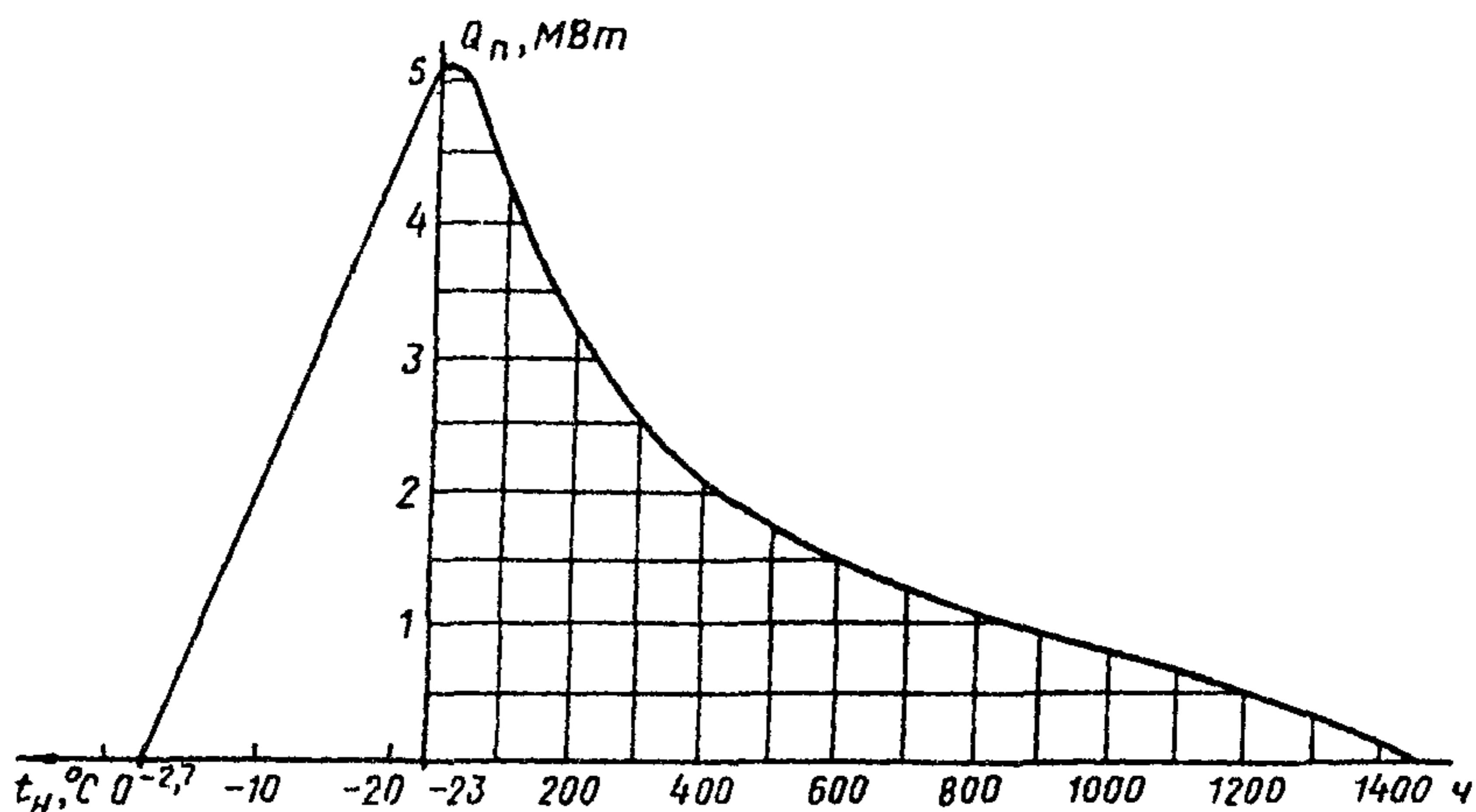
Рис. 1. График продолжительности тепловой нагрузки пикового источника теплоты
