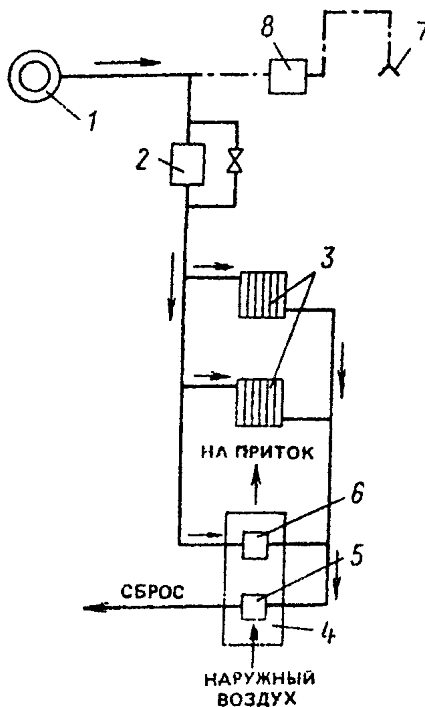
Рис. 14. Принципиальная схема системы геотермального теплоснабжения с комбинированным использованием систем водяного и воздушного отопления
