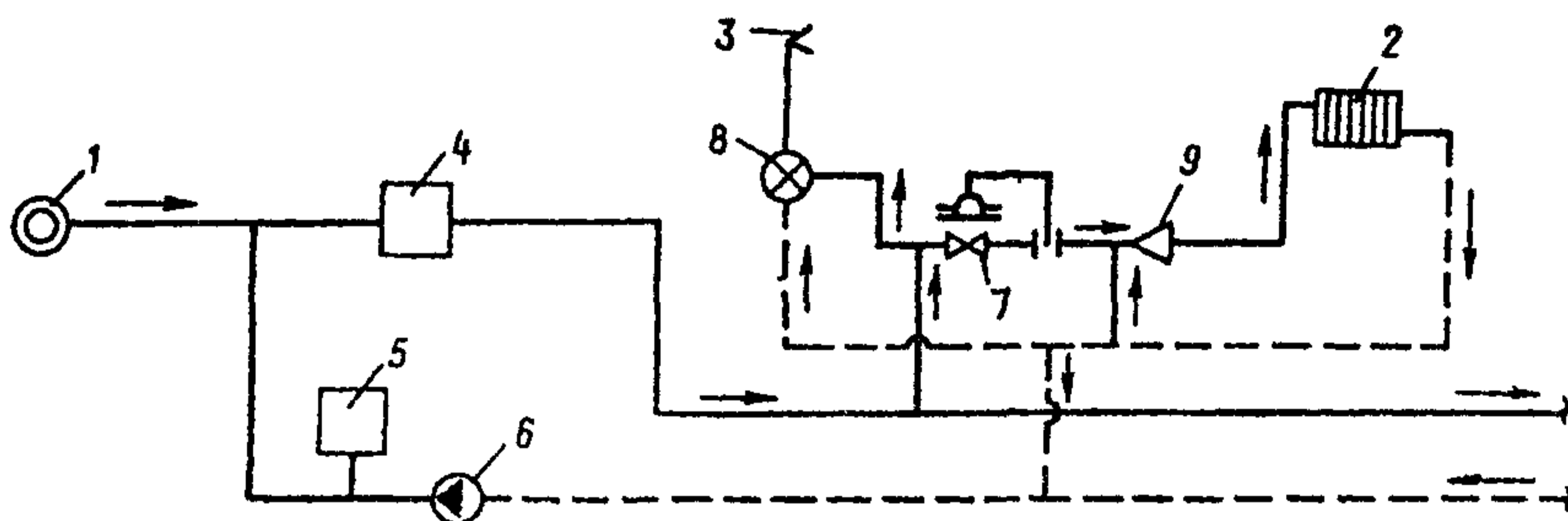
Рис. 10. Принципиальная схема бессливной системы геотермального теплоснабжения
