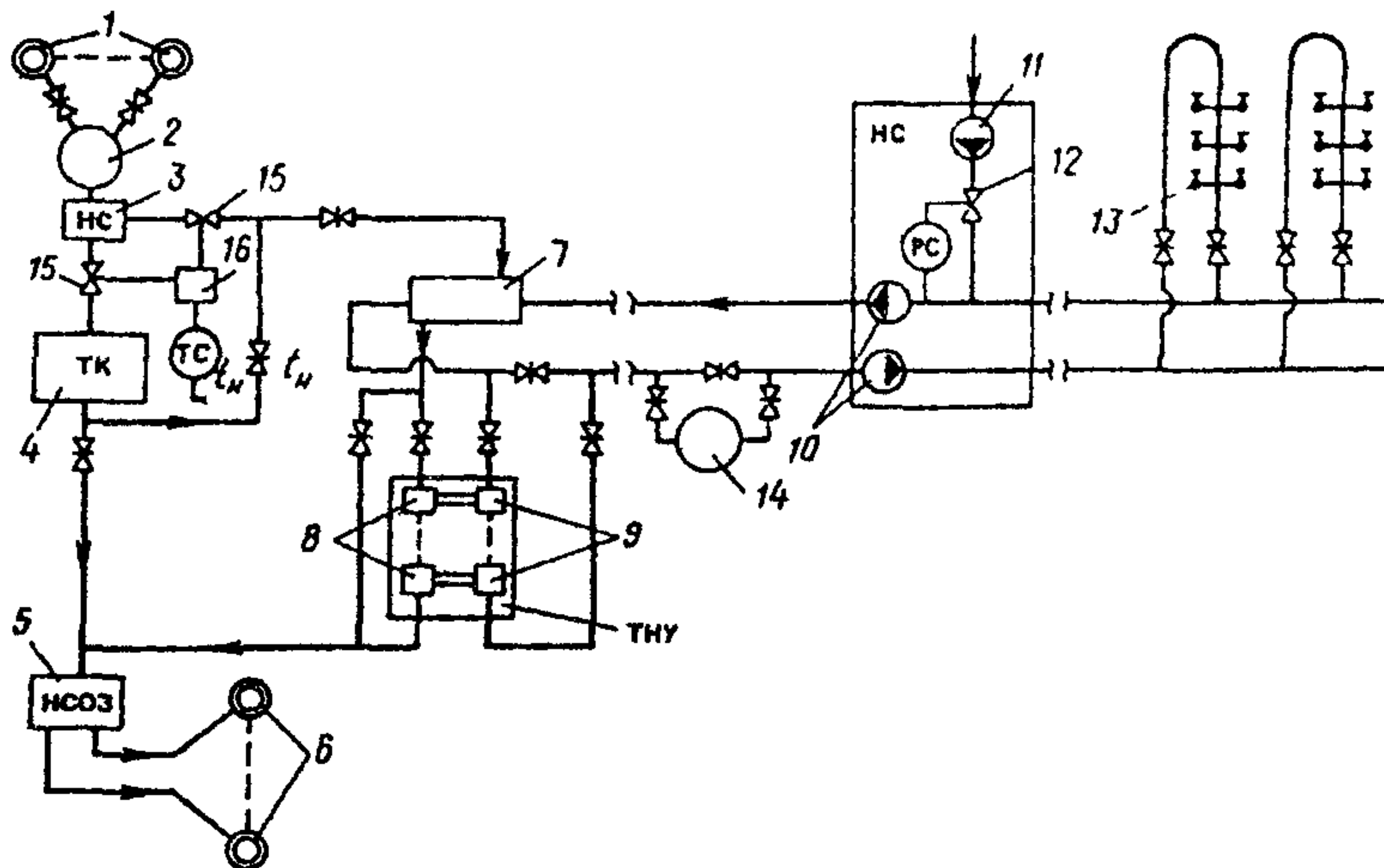
Рис. 16. Комплексная двухтрубная геотермальная система теплоснабжения с ТНУ 1 — геотермальные скважины; 2 — промежуточная емкость; 3 — насосная станция; 4 — отопление тепличного комбината; 5 — насосная станция обратной закачки; 6 — скважины обратной закачки; 7 — сетевой теплообменник; 8 — испарители ТНУ; 9 — конденсаторы ТНУ; 10 — сетевые насосы; 11 — подпиточный насос; 12 — регулятор подпитки; 13 — водоразборный кран; 14 — сетевой бак-аккумулятор; 15 — регулирующие задвижки; 16 — регулятор
