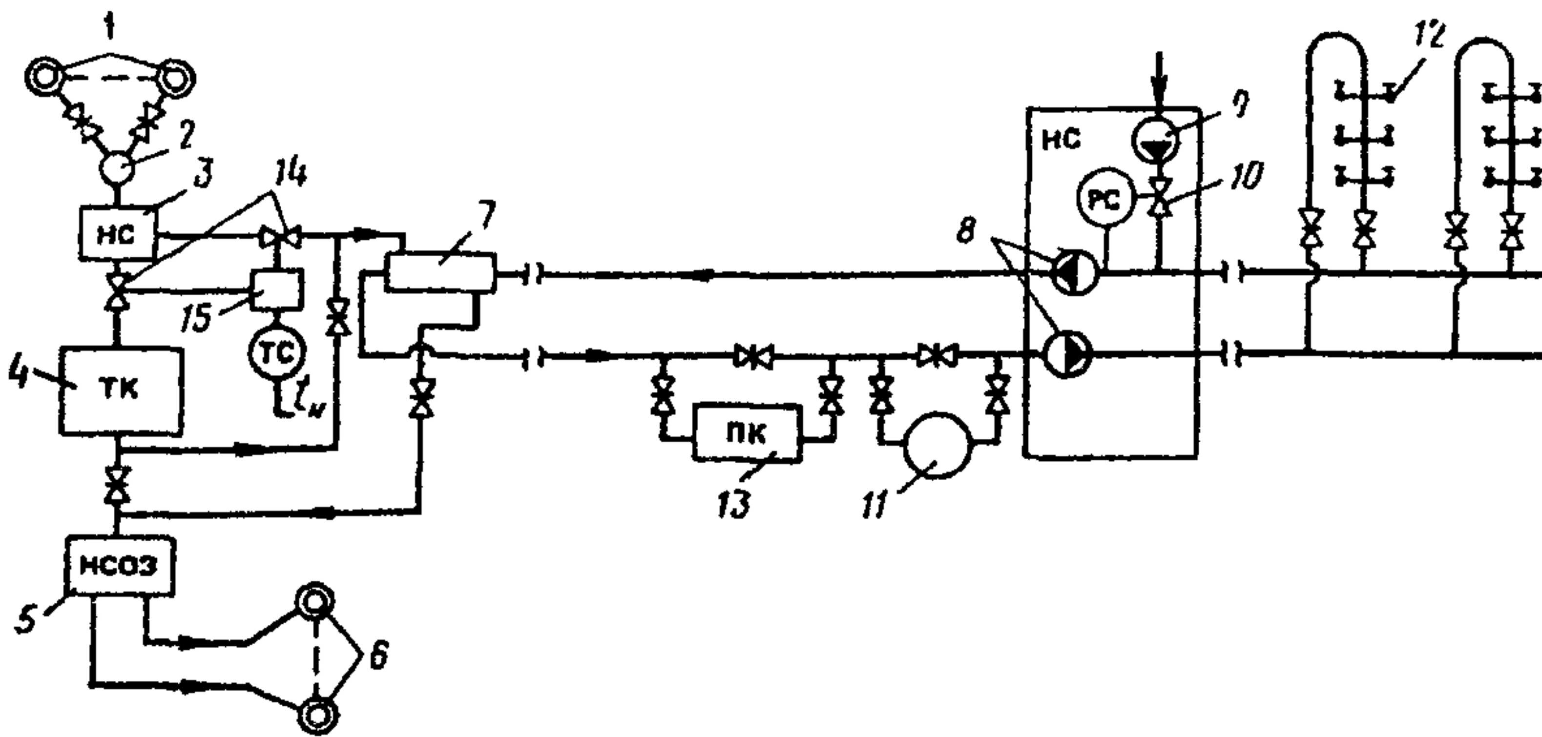
Рис. 15. Комплексная двухтрубная геотермальная система теплоснабжения с пиковой котельной
