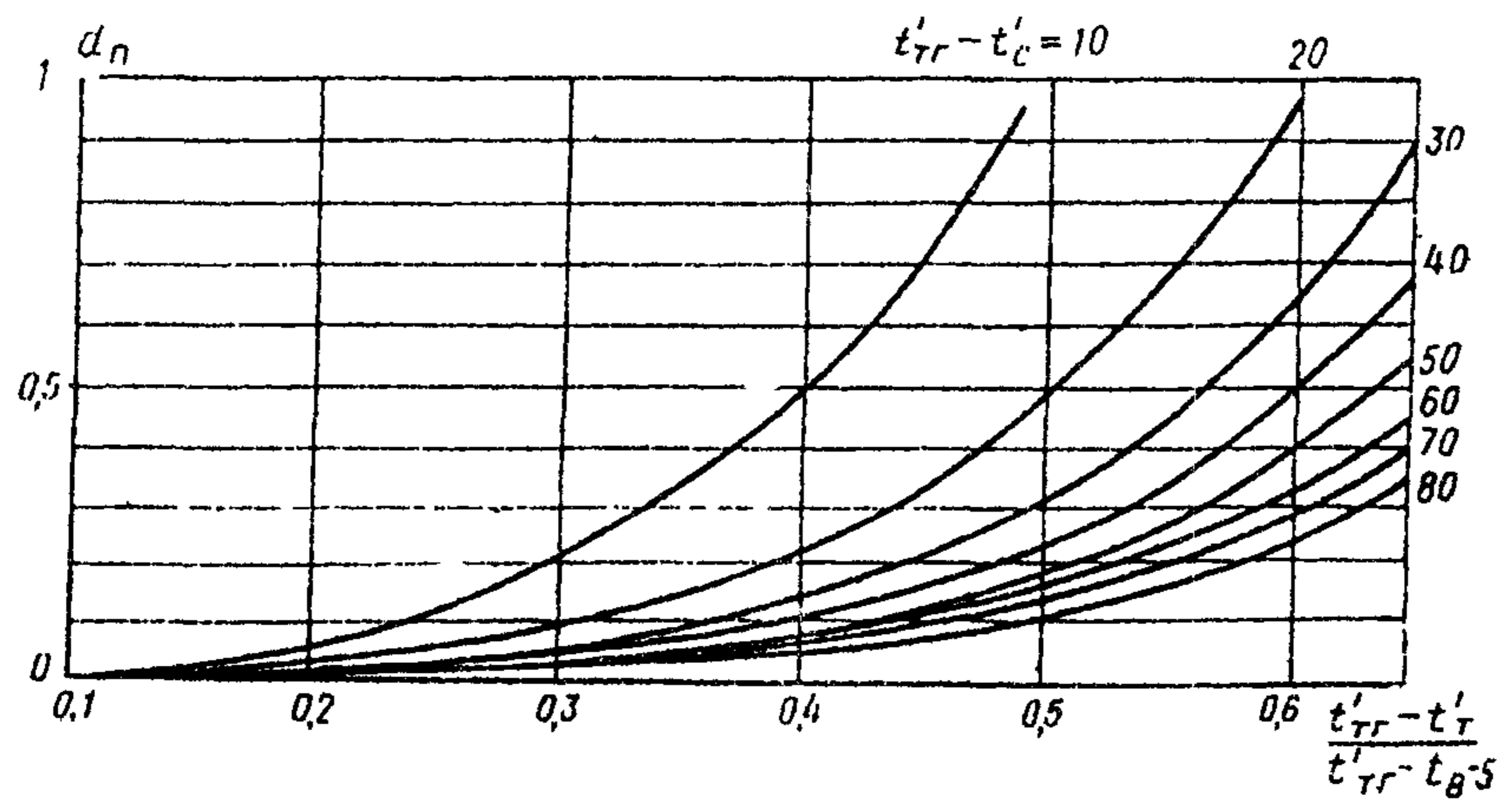
Рис. 2. Графики для определения доли пикового догрева при отоплении
