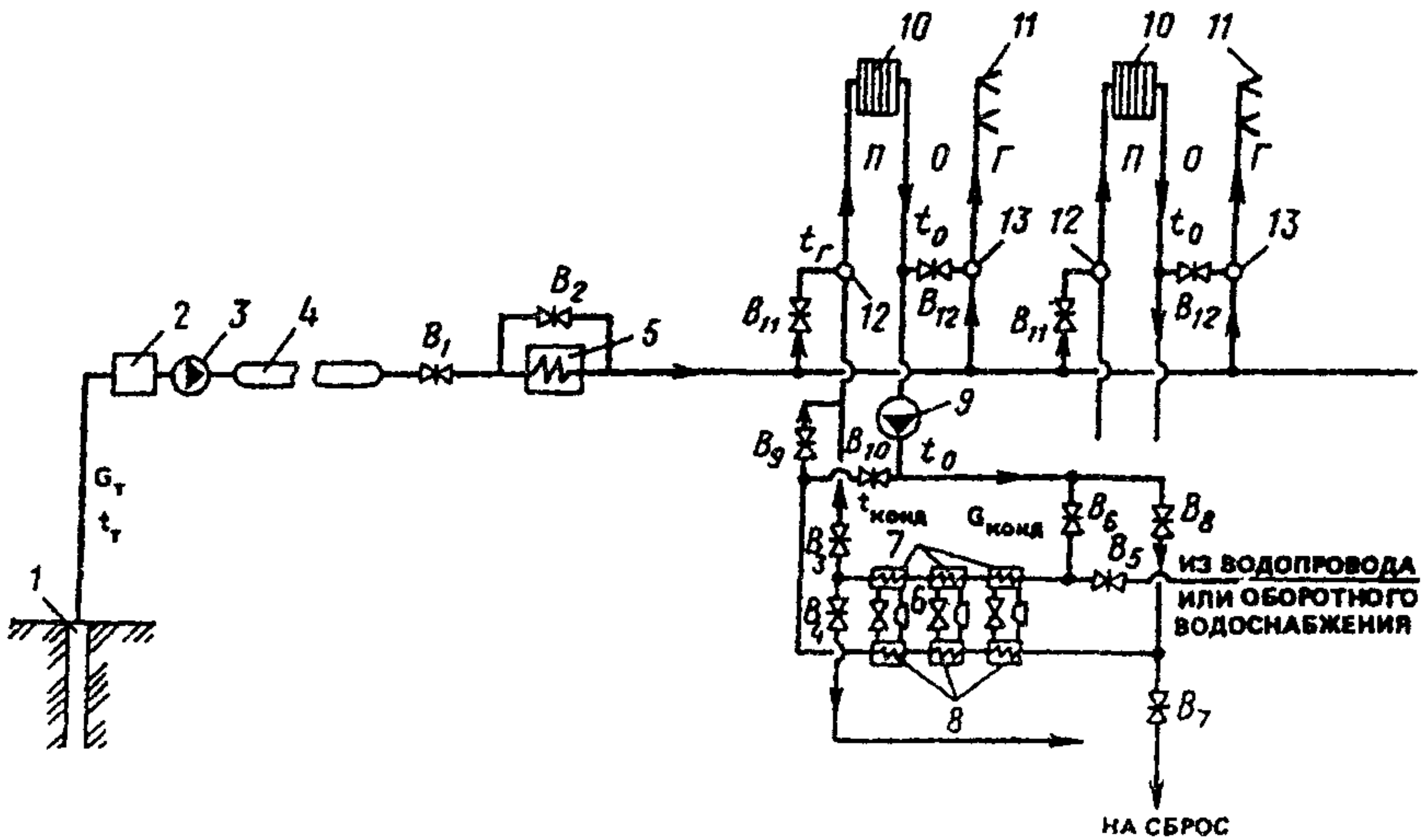
Рис. 13. Система децентрализованного теплохладоснабжения с тепловыми насосами
